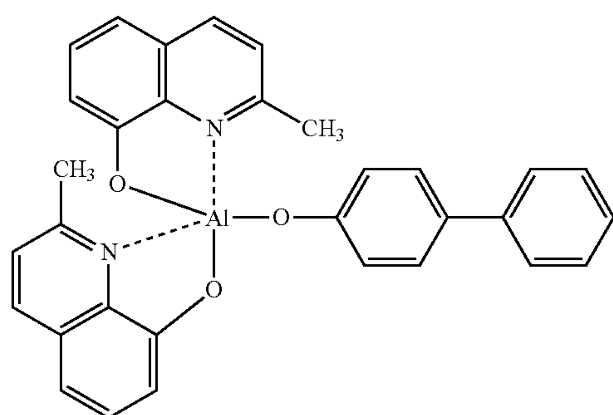
(BAlq)
