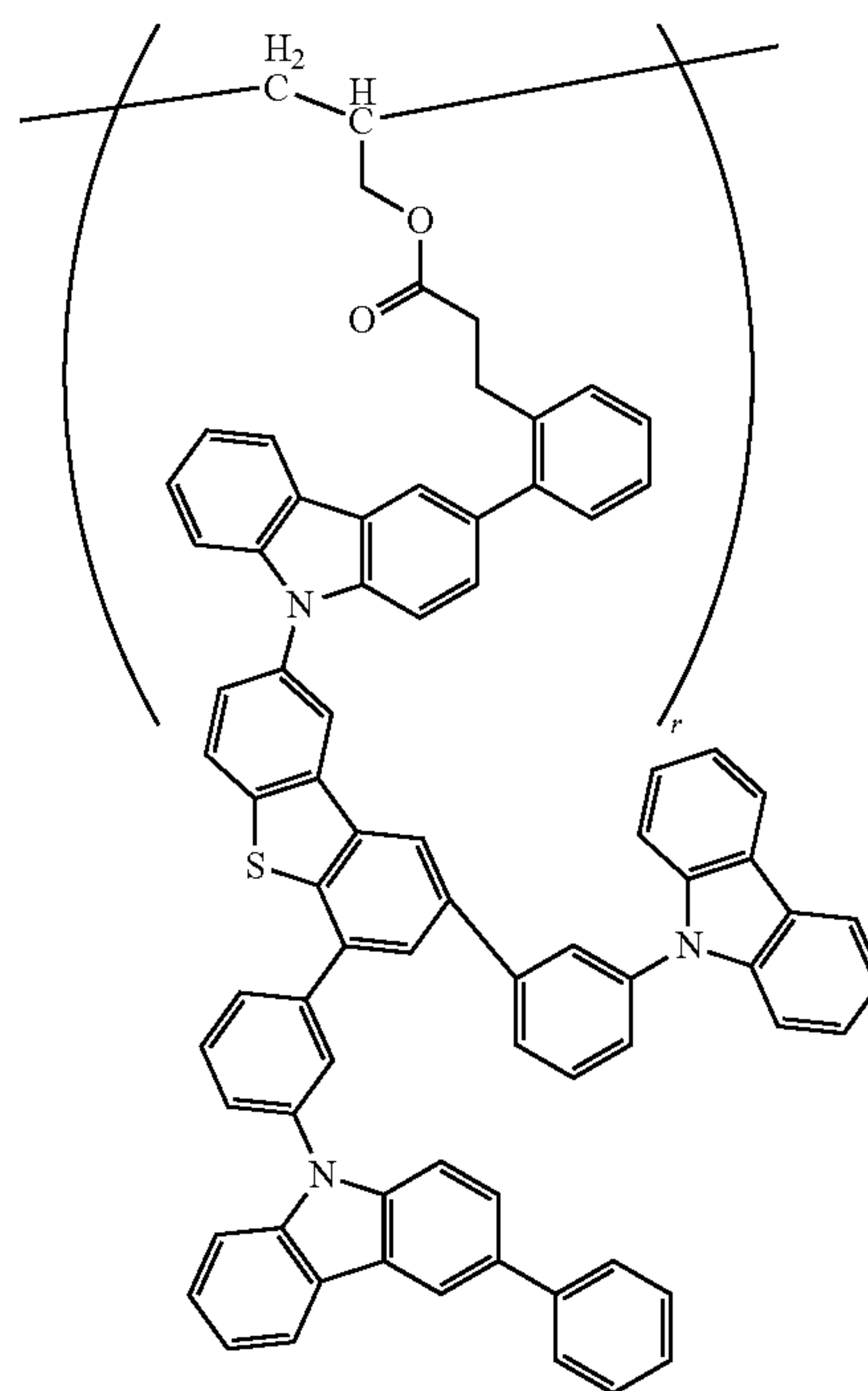
III-61
