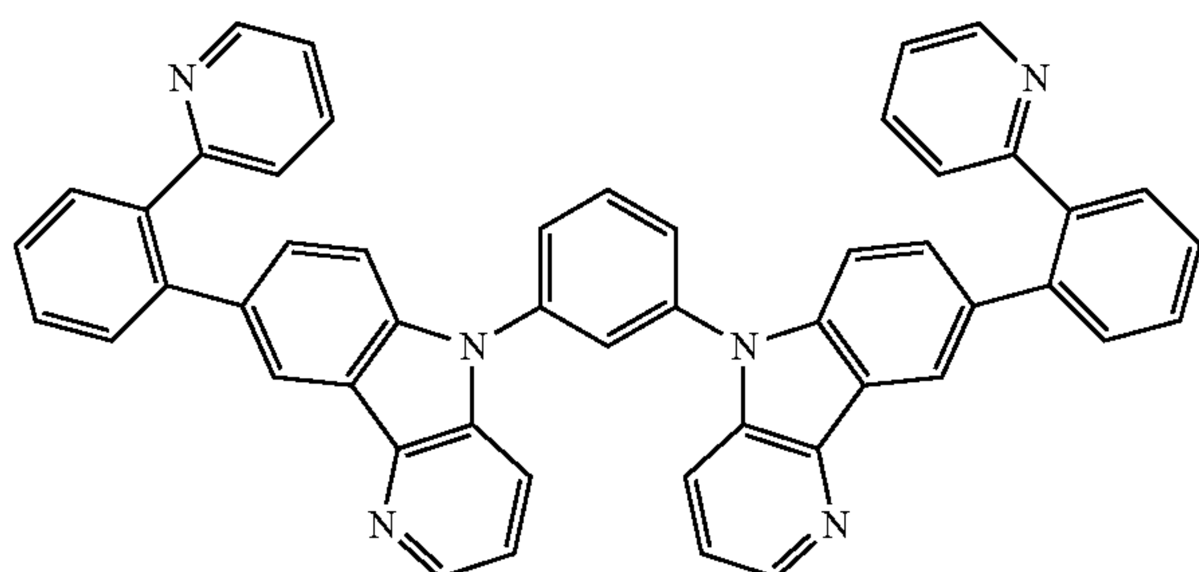
ET-11
