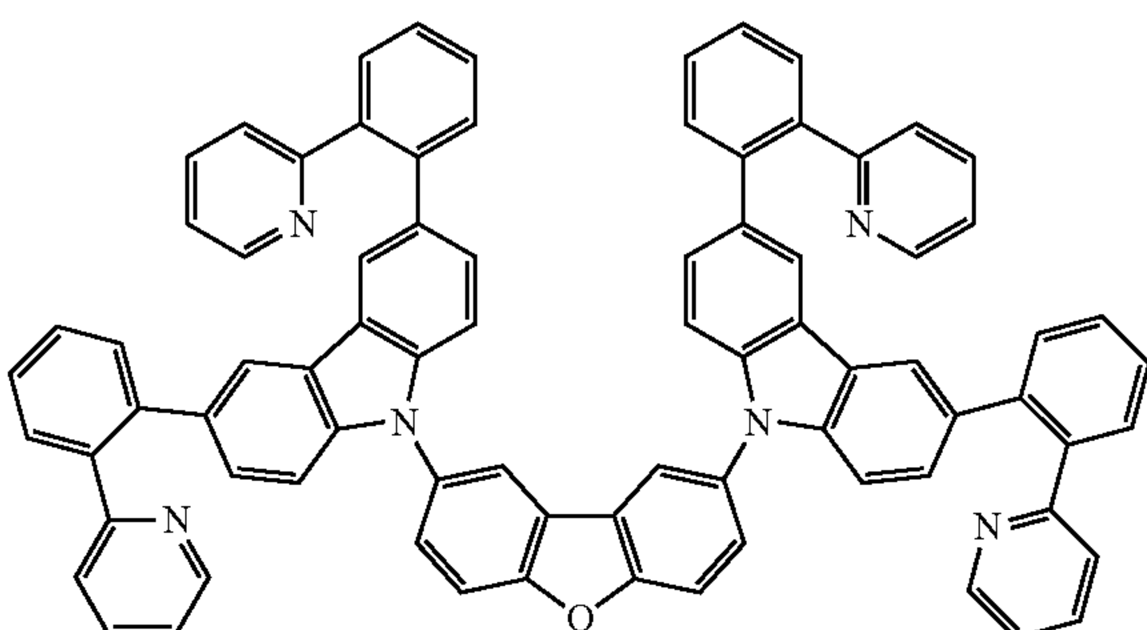
ET-11
