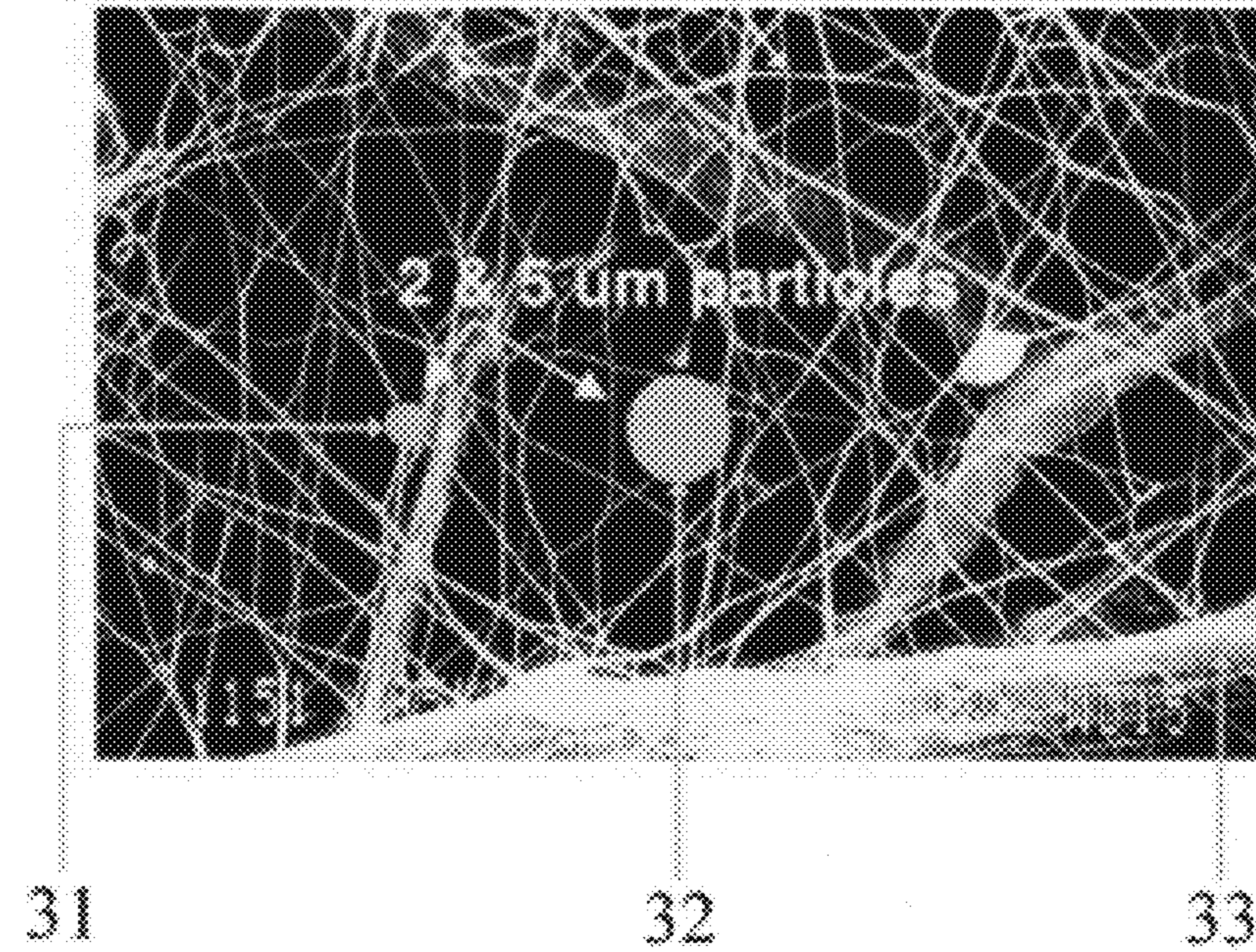
FIG. 3B Ultra-Web
