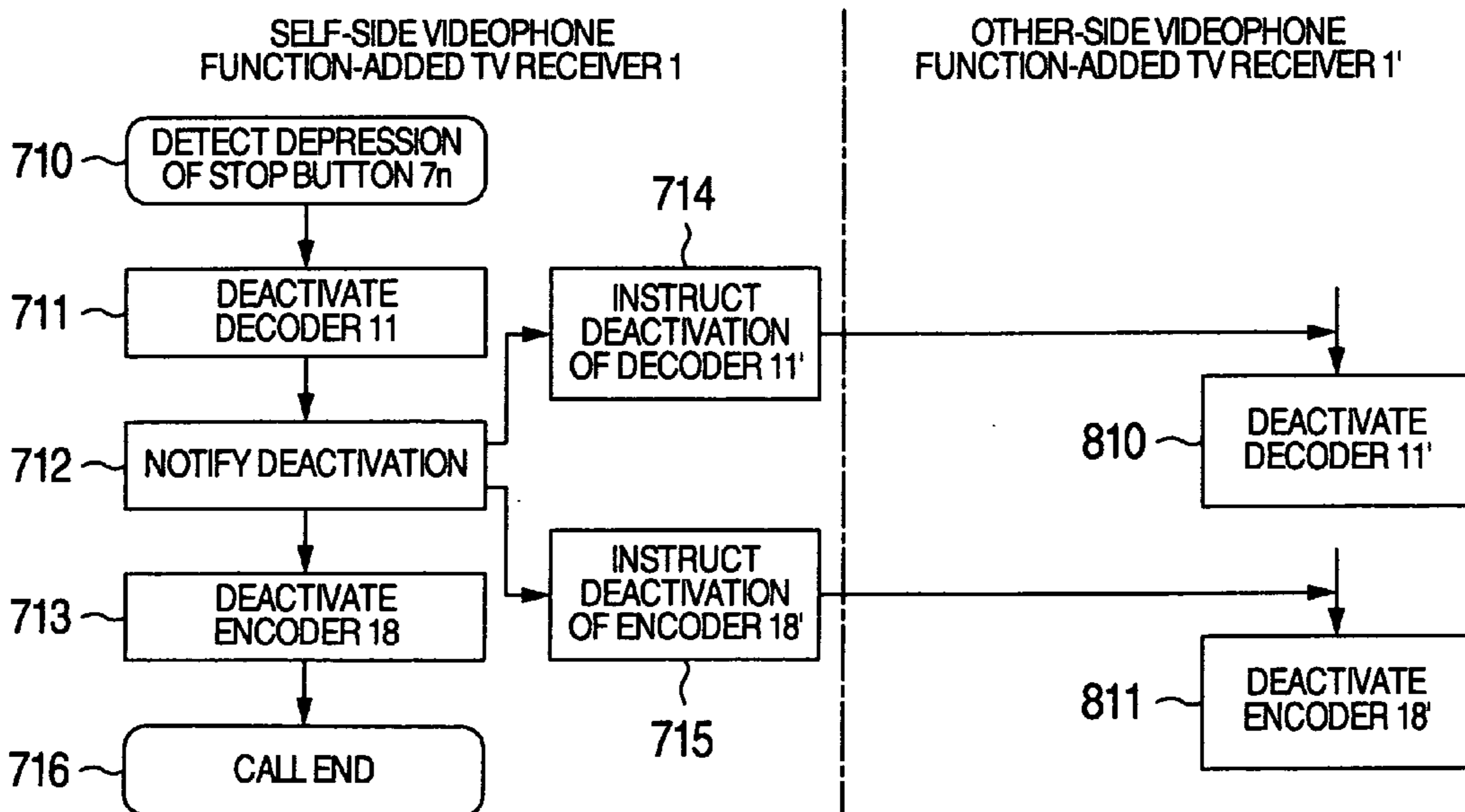
FIG.7B
