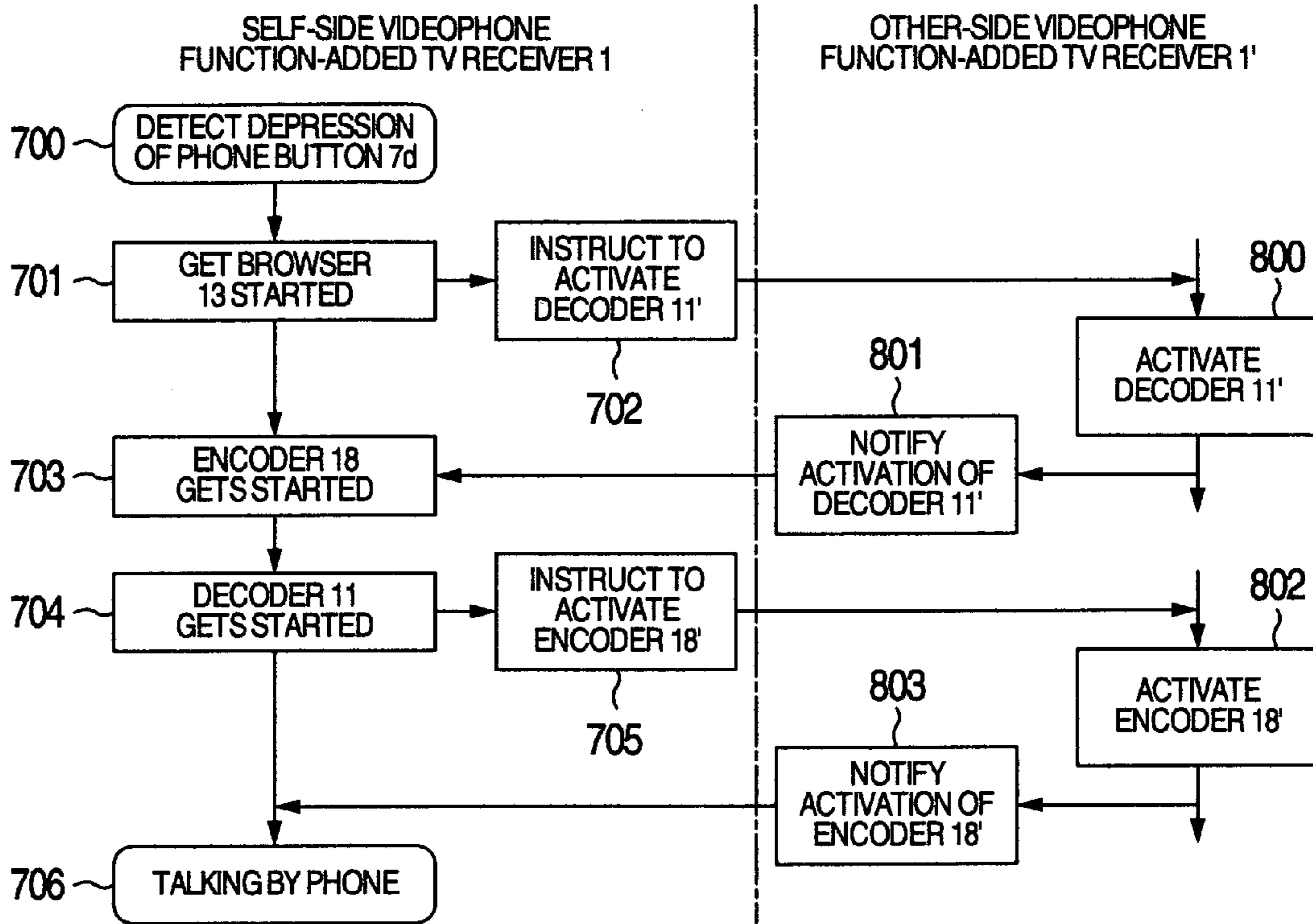
FIG.7A
