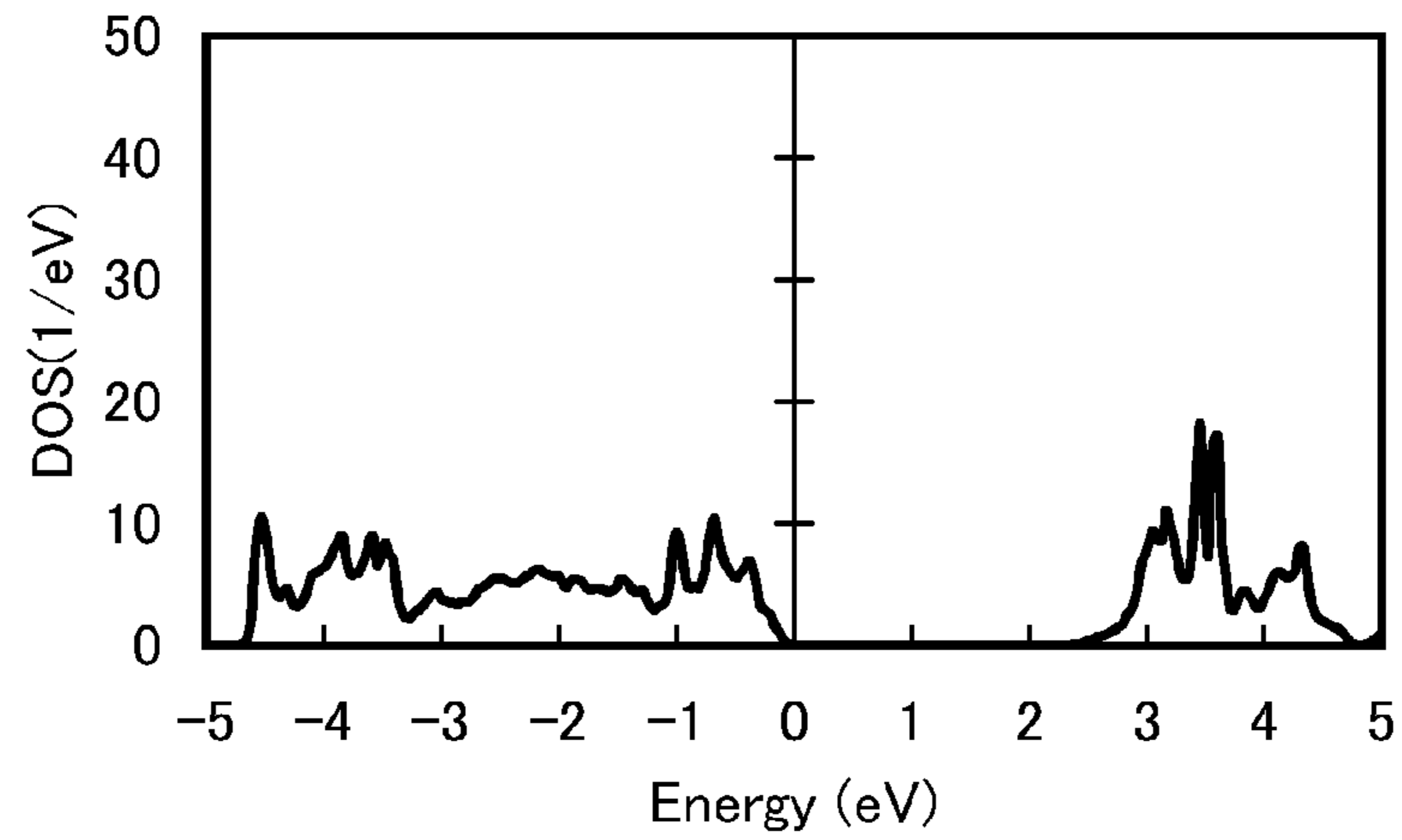
FIG. 12B \text{TiO}_2 (Rutile type)
