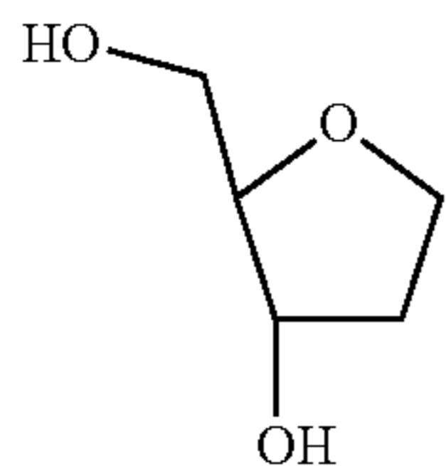
1,2-Dideoxyribose
