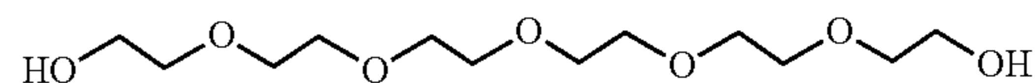
Hexaethylene glycol
