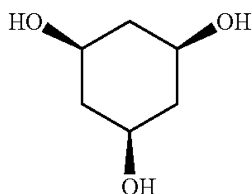
cis-1,3,5-Cyclohexanetriol
