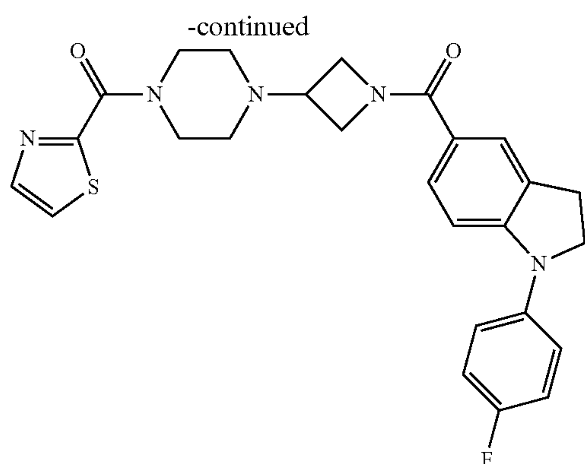
Cpd 885
