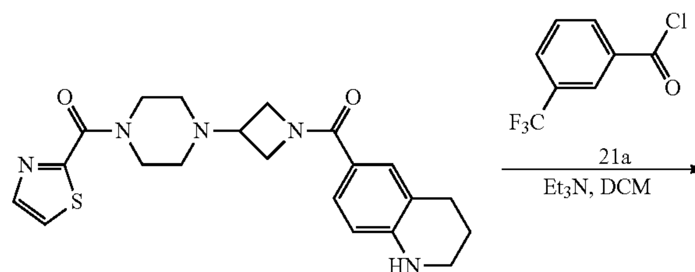
Cpd 357
