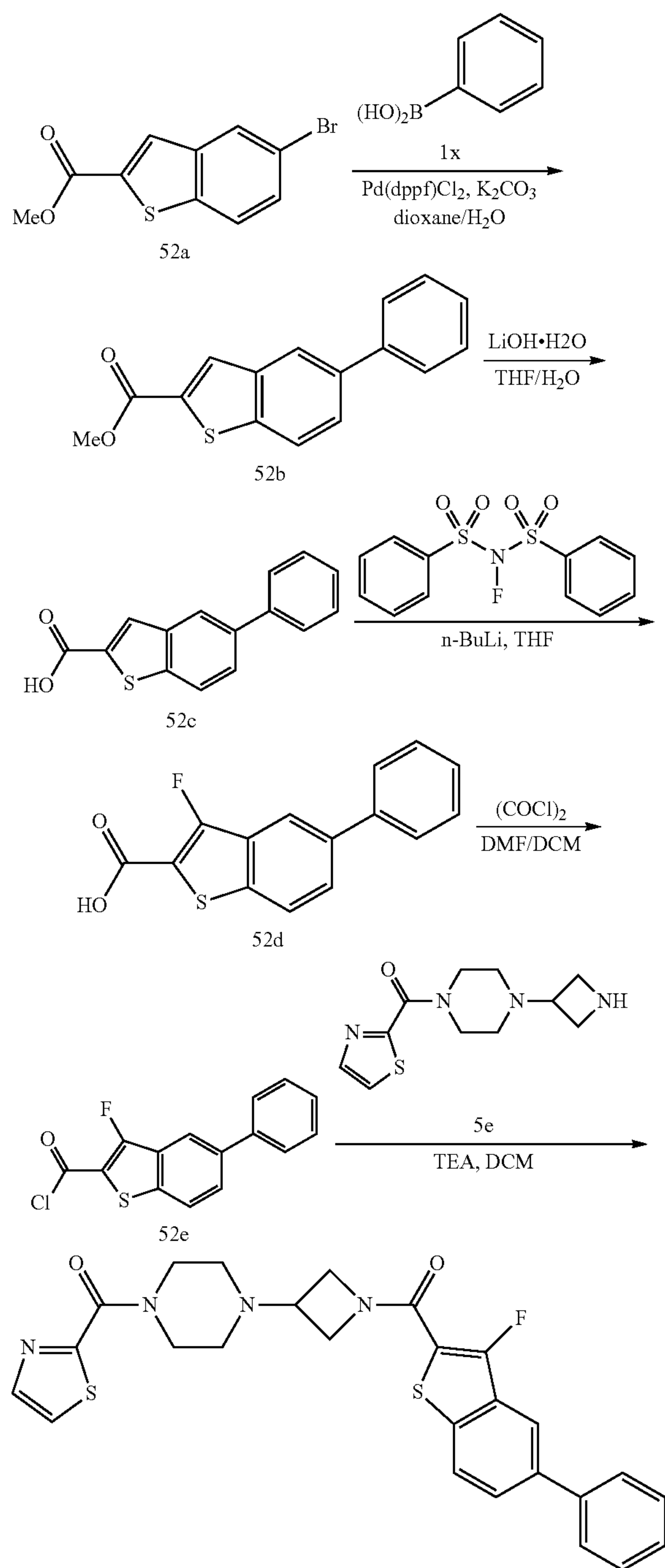
Cpd 1315
