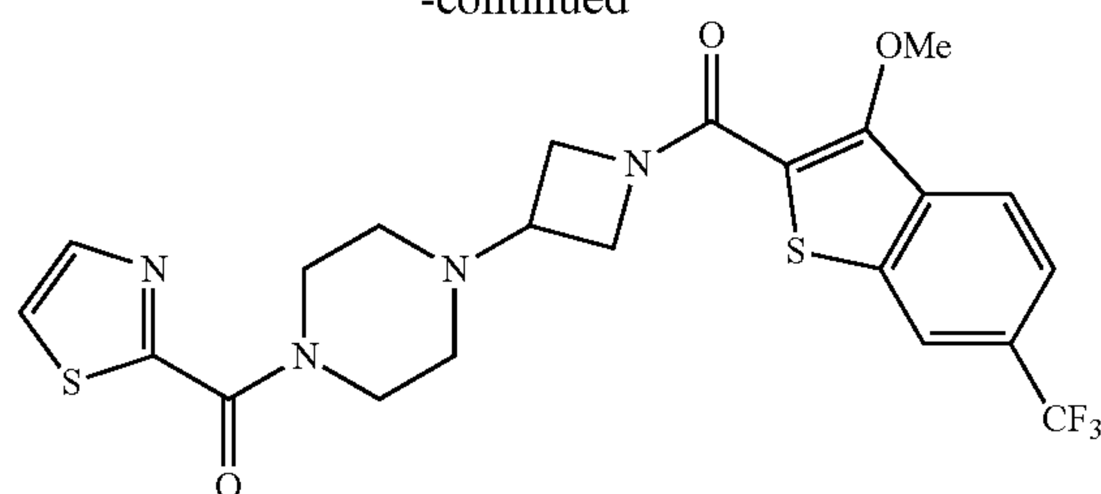
Cpd 649
