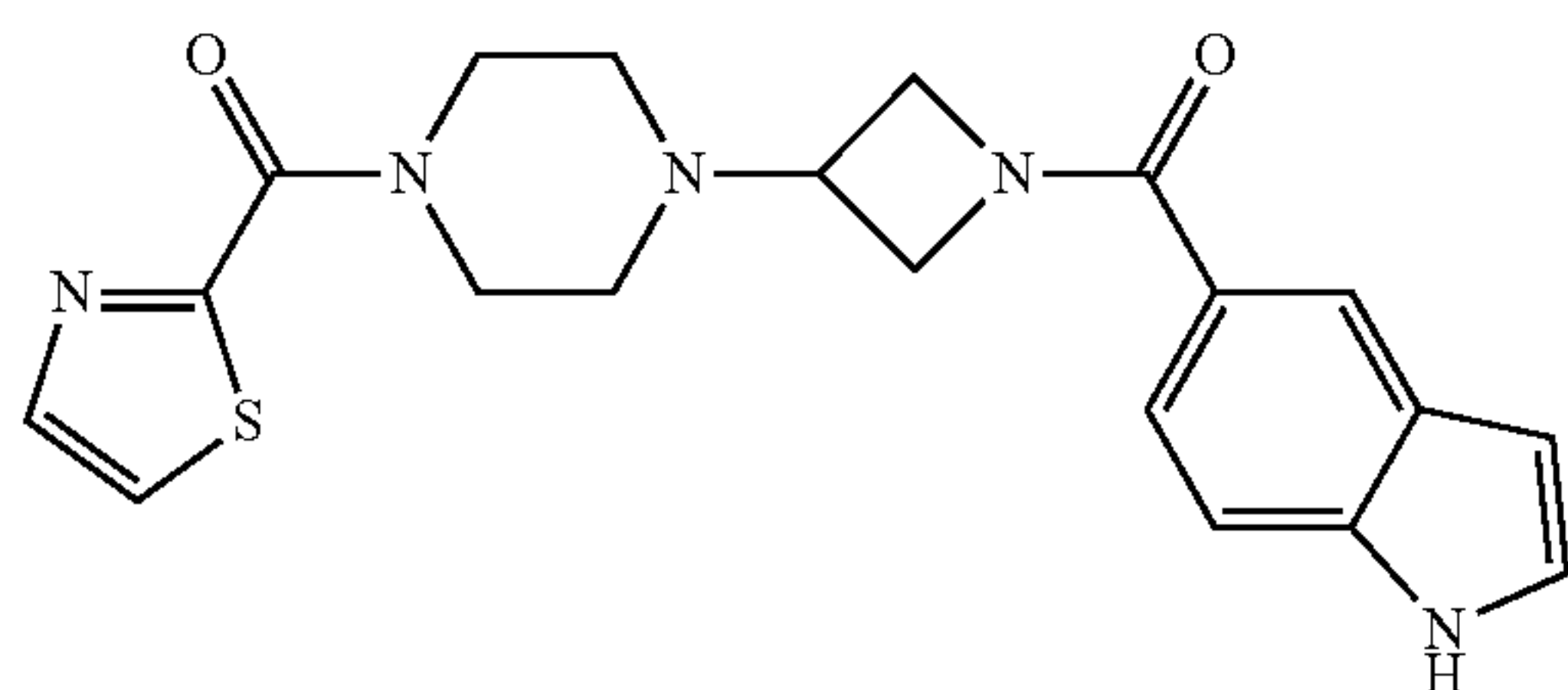
Cpd 911
