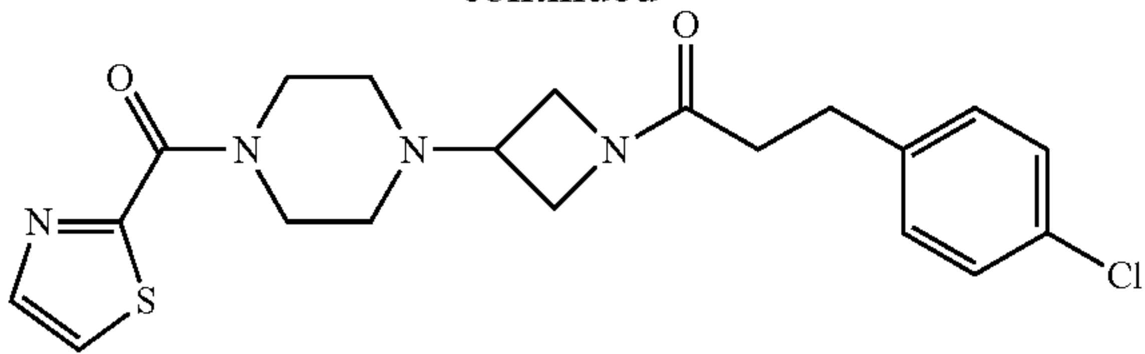
Cpd 269
