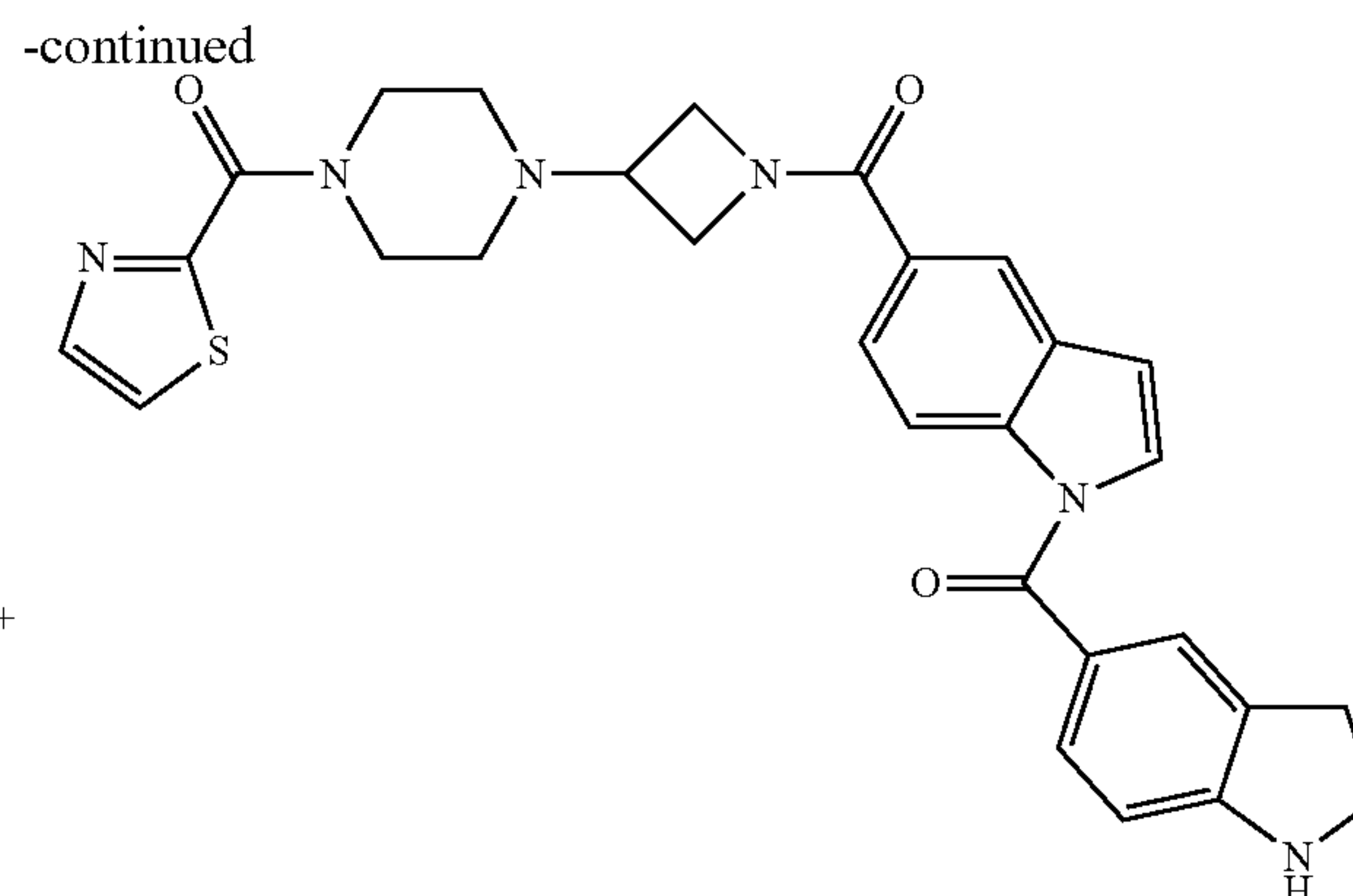
Cpd 988
