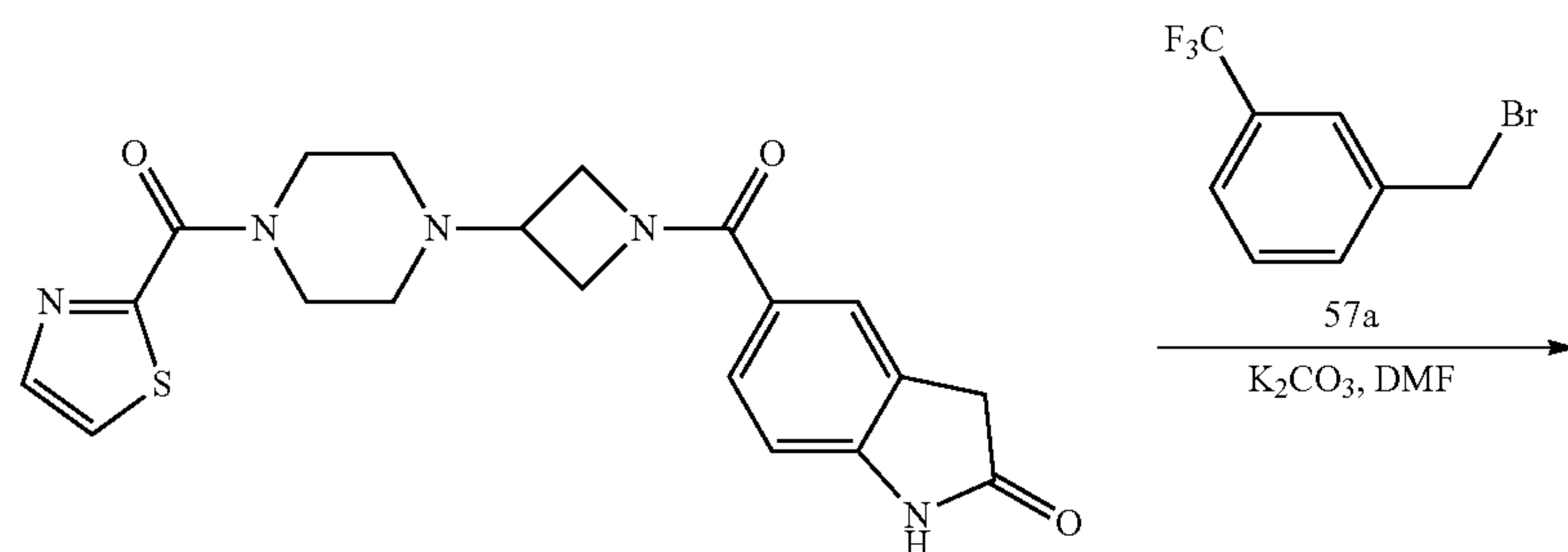
Cpd 918
