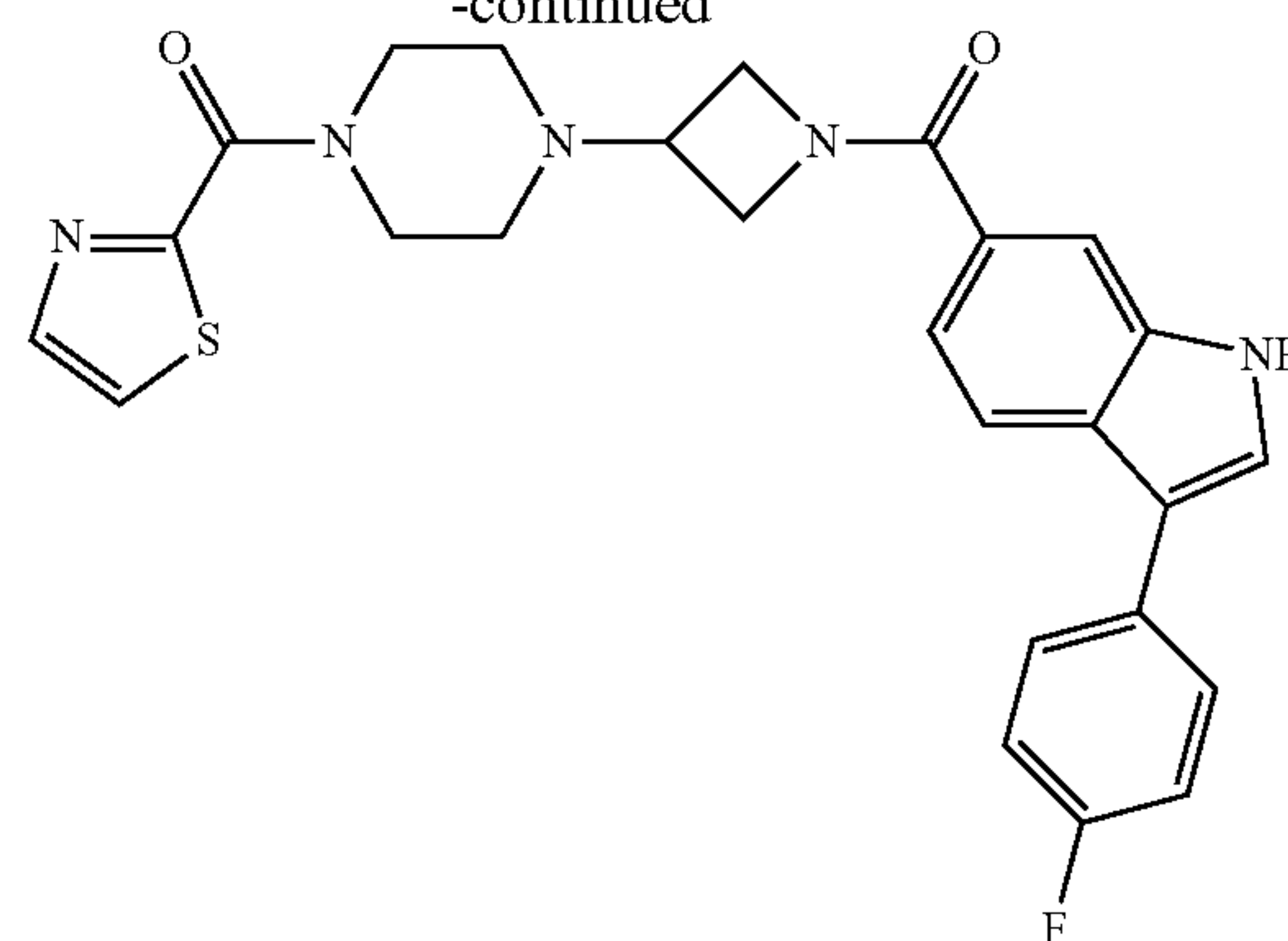
Cpd 1317
