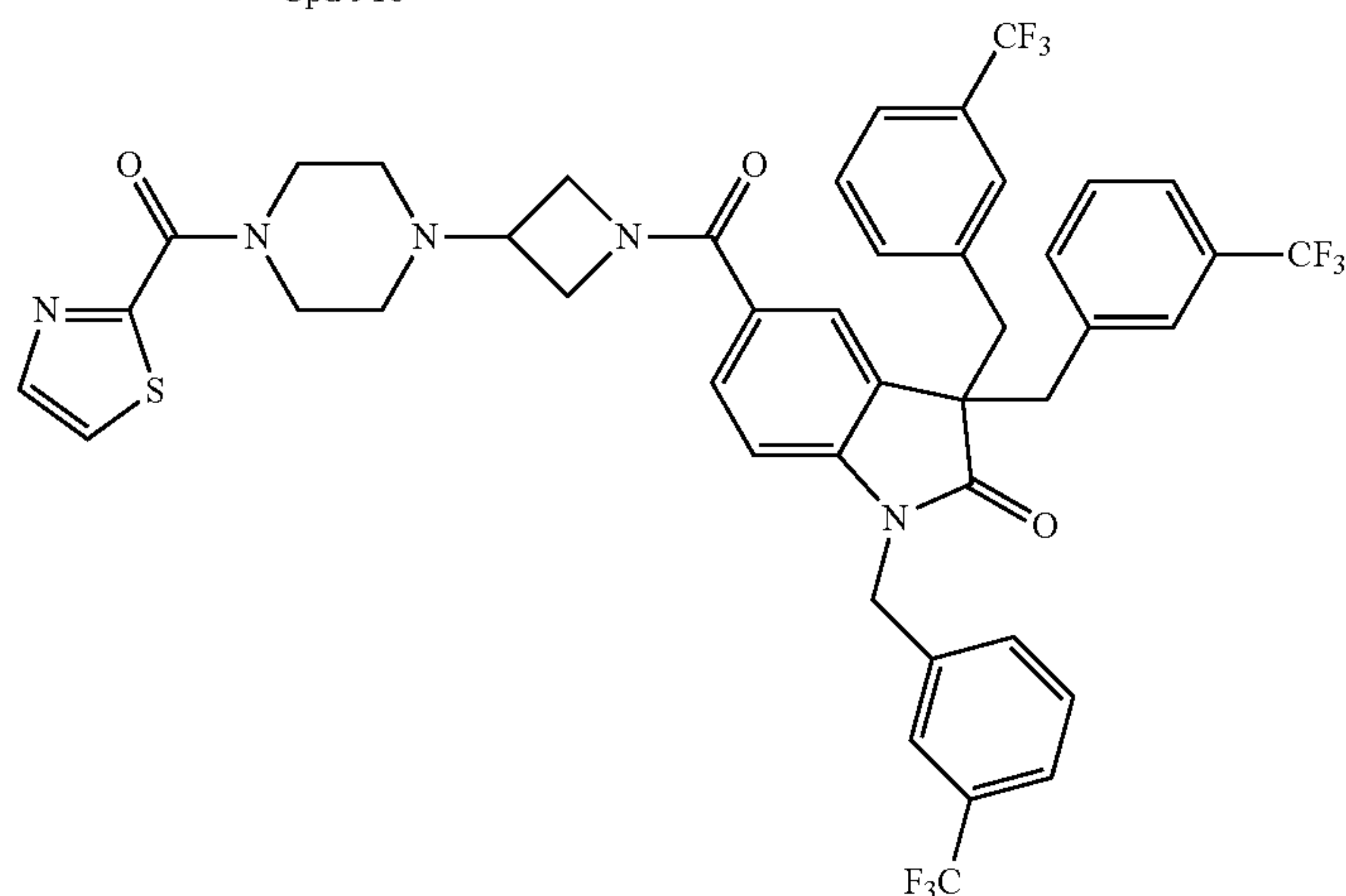
Cpd 1430
