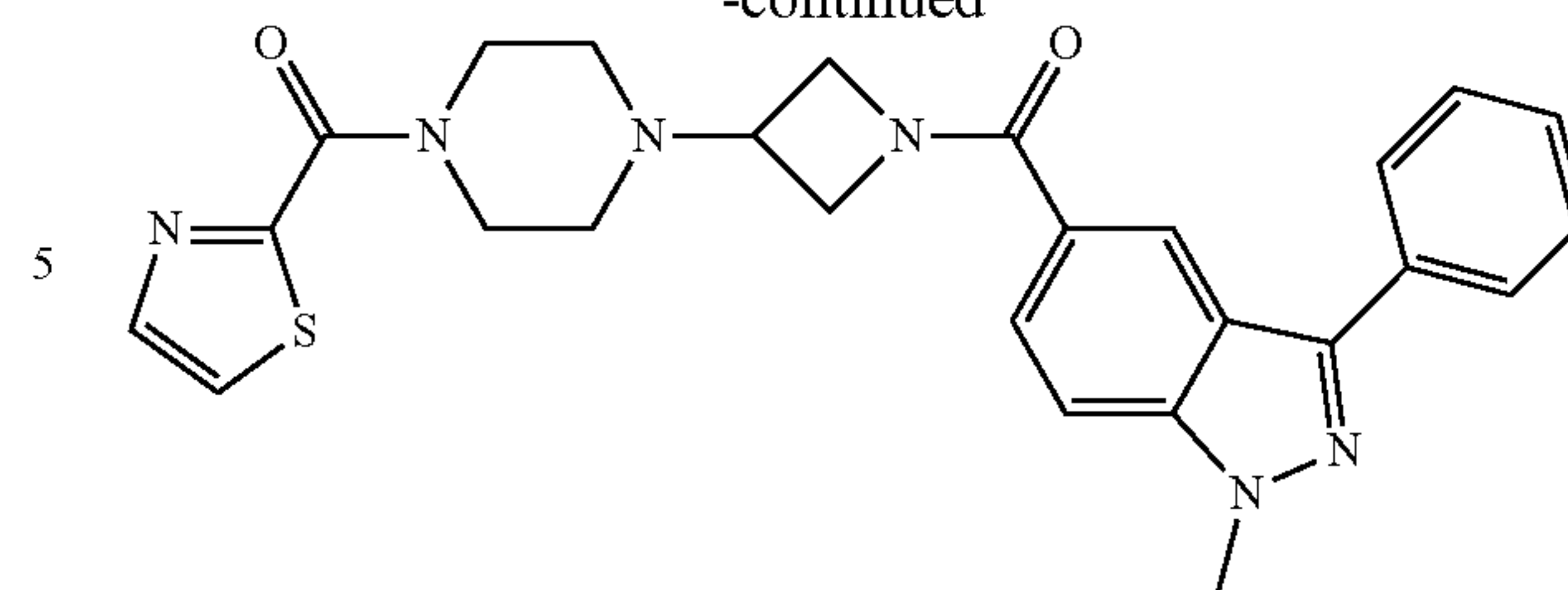
Cpd 1137
