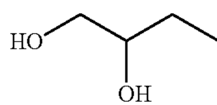
1,4-Butanediol
