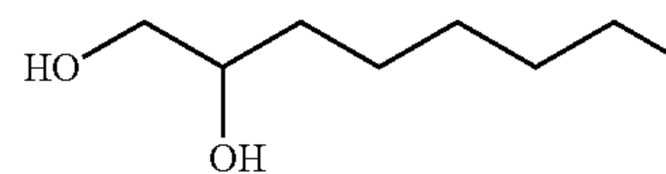
1,2-Octanediol
