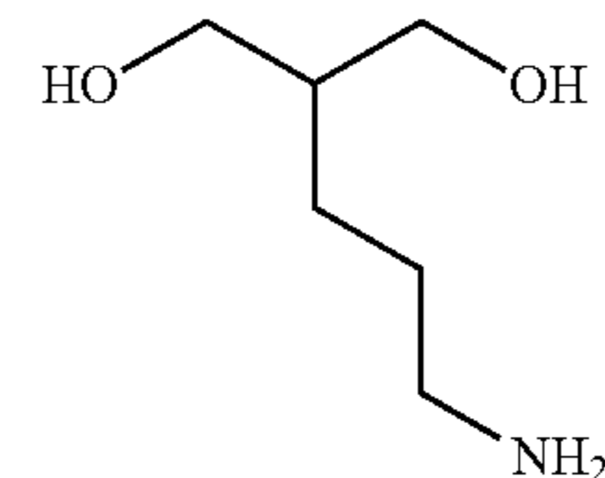
2-(1-Aminopropyl)-1,3-propanediol
