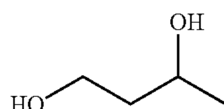
1,3-Butanediol
