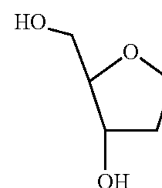
1,2-Dideoxyribose
