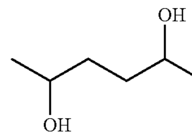
2,5-Hexanediol
