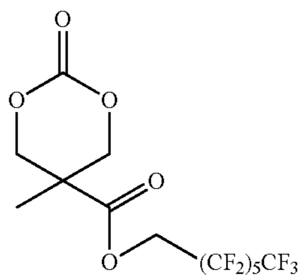
(MTCOBn)
