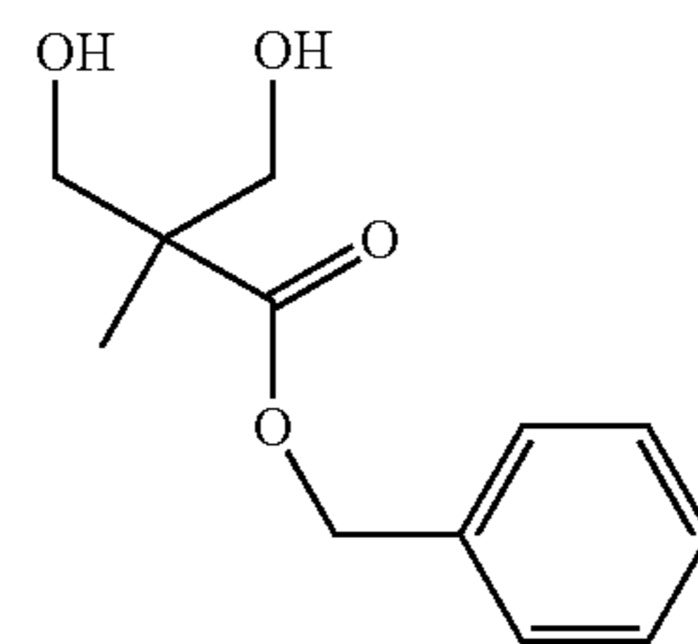
(BnMPA)
