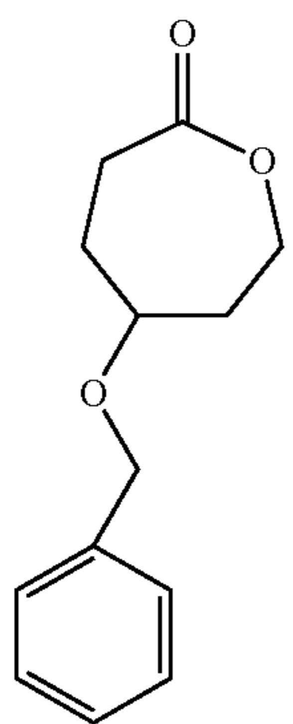
5-(Benzyloxy)oxepan-2-one (BXO)
