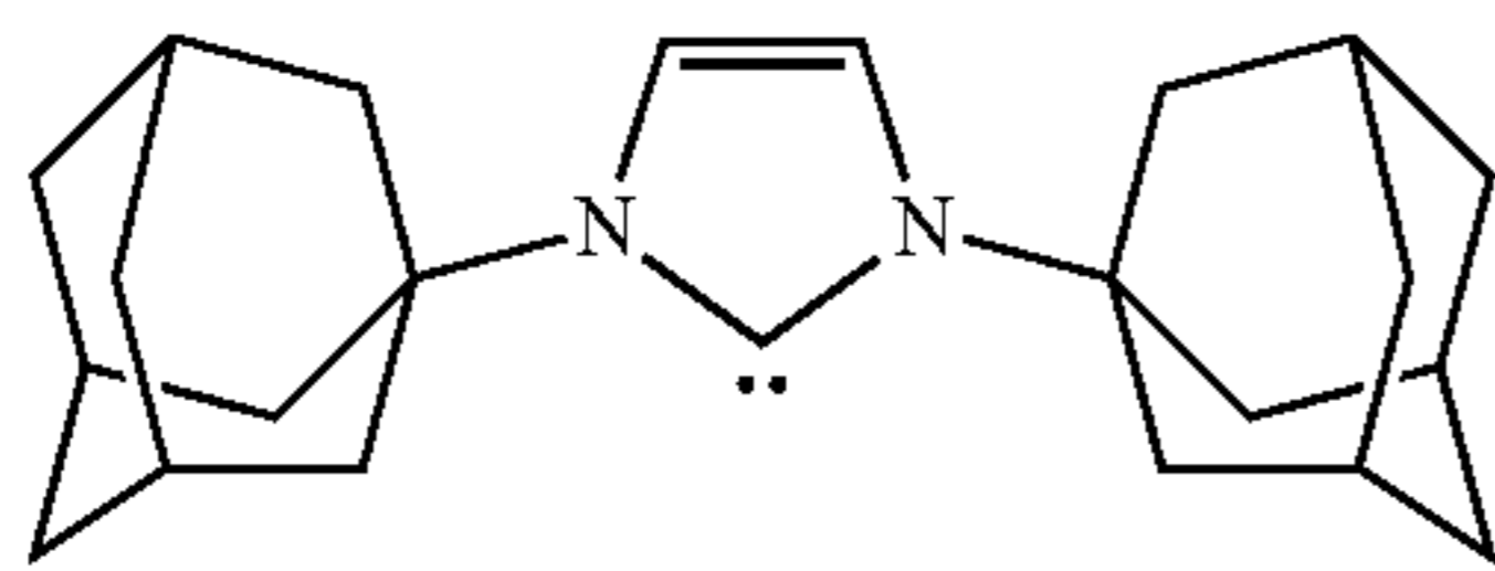
1,3-Bis(1-adamantyl)imidazol-2-ylidene (Im-4)
