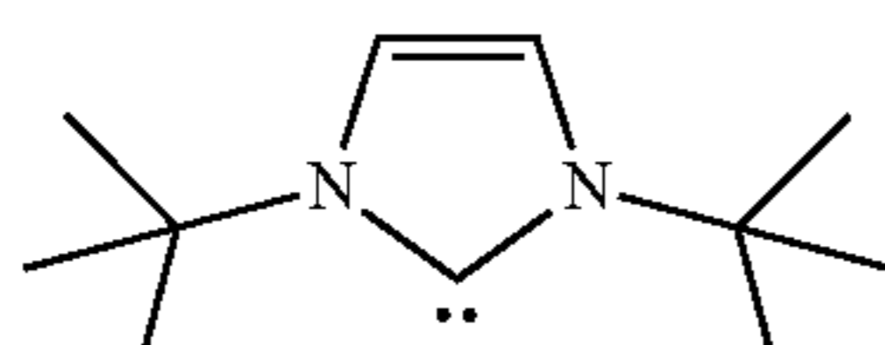
1,3-Di-t-butylimidazol-2-ylidene (Im-6)
