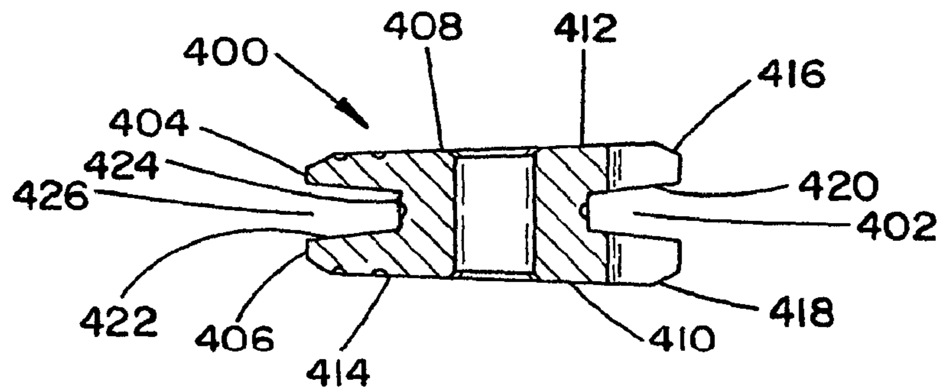
Section A-A
