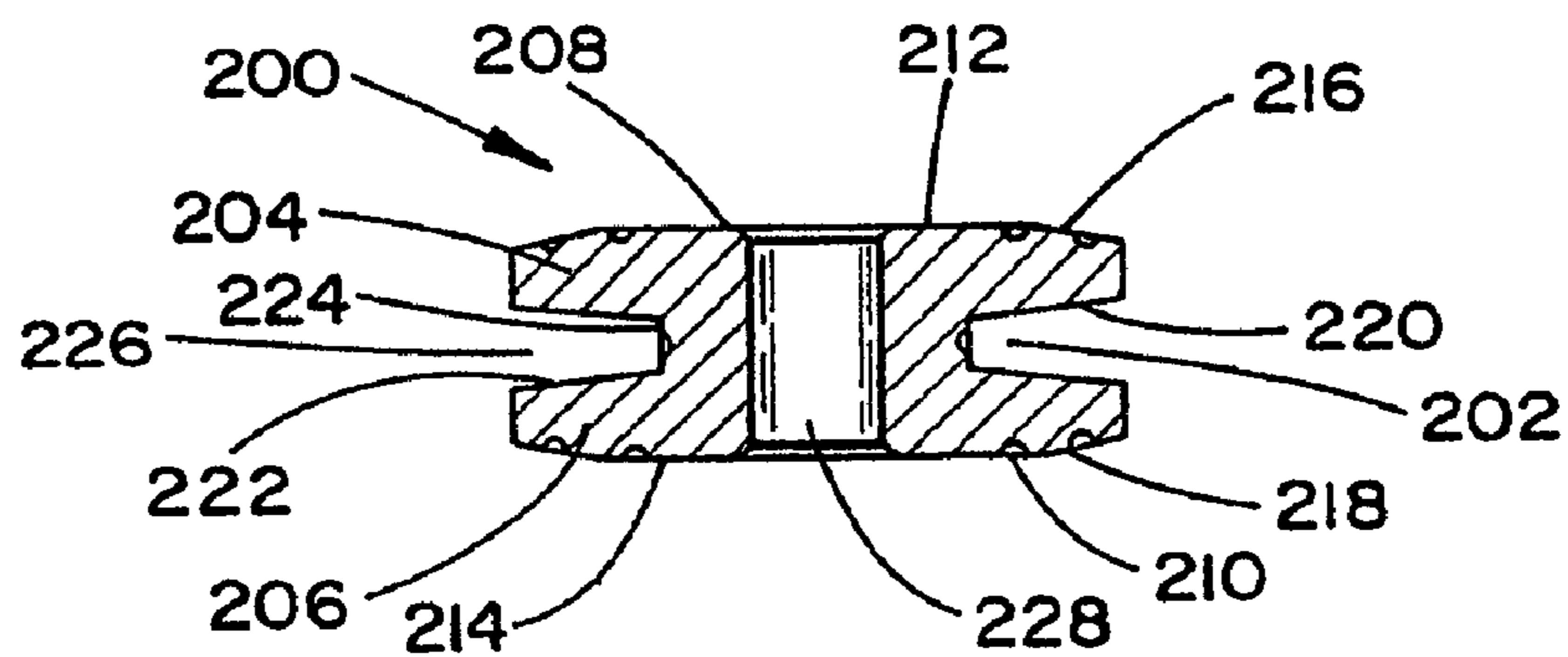
Section A-A
