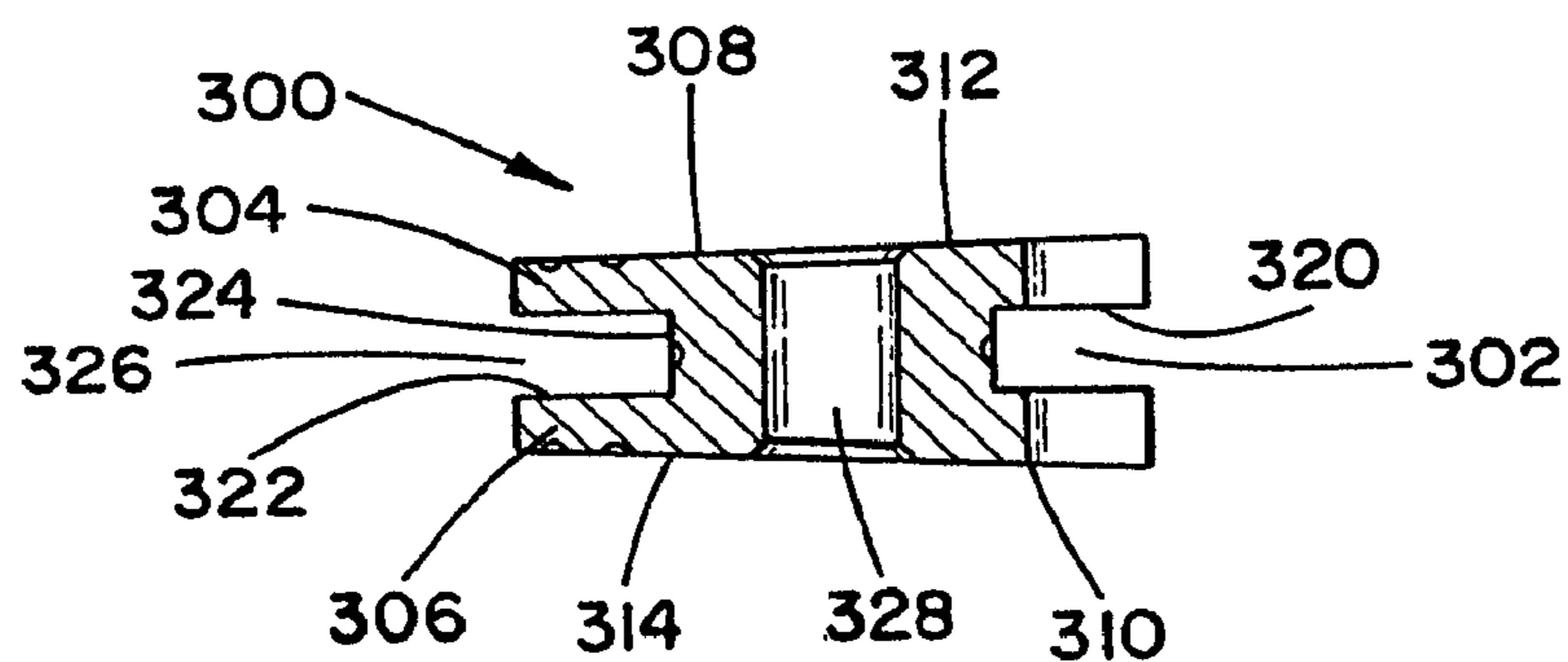
Section A-A
