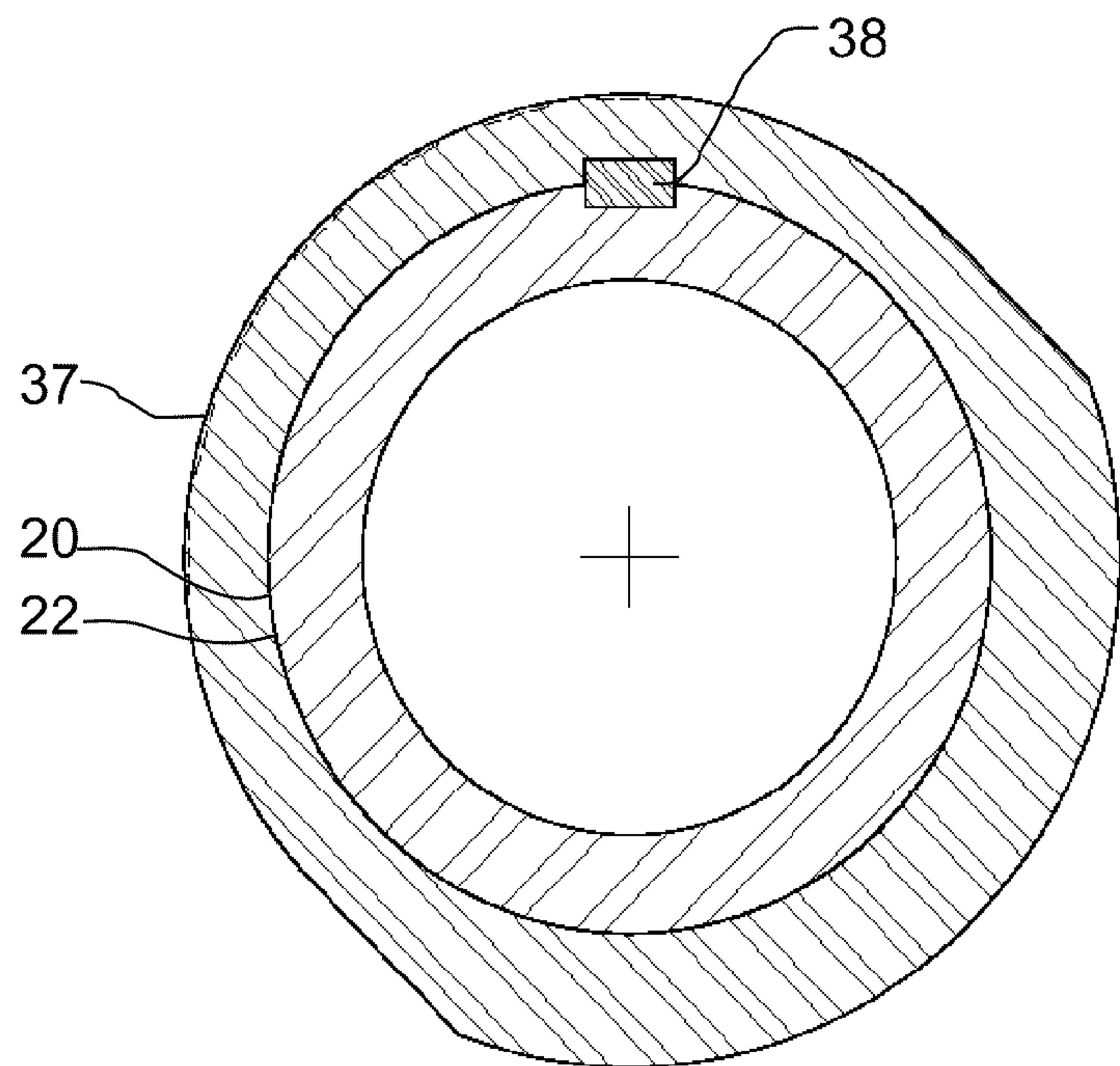
SECTION B-B FIG. 5
