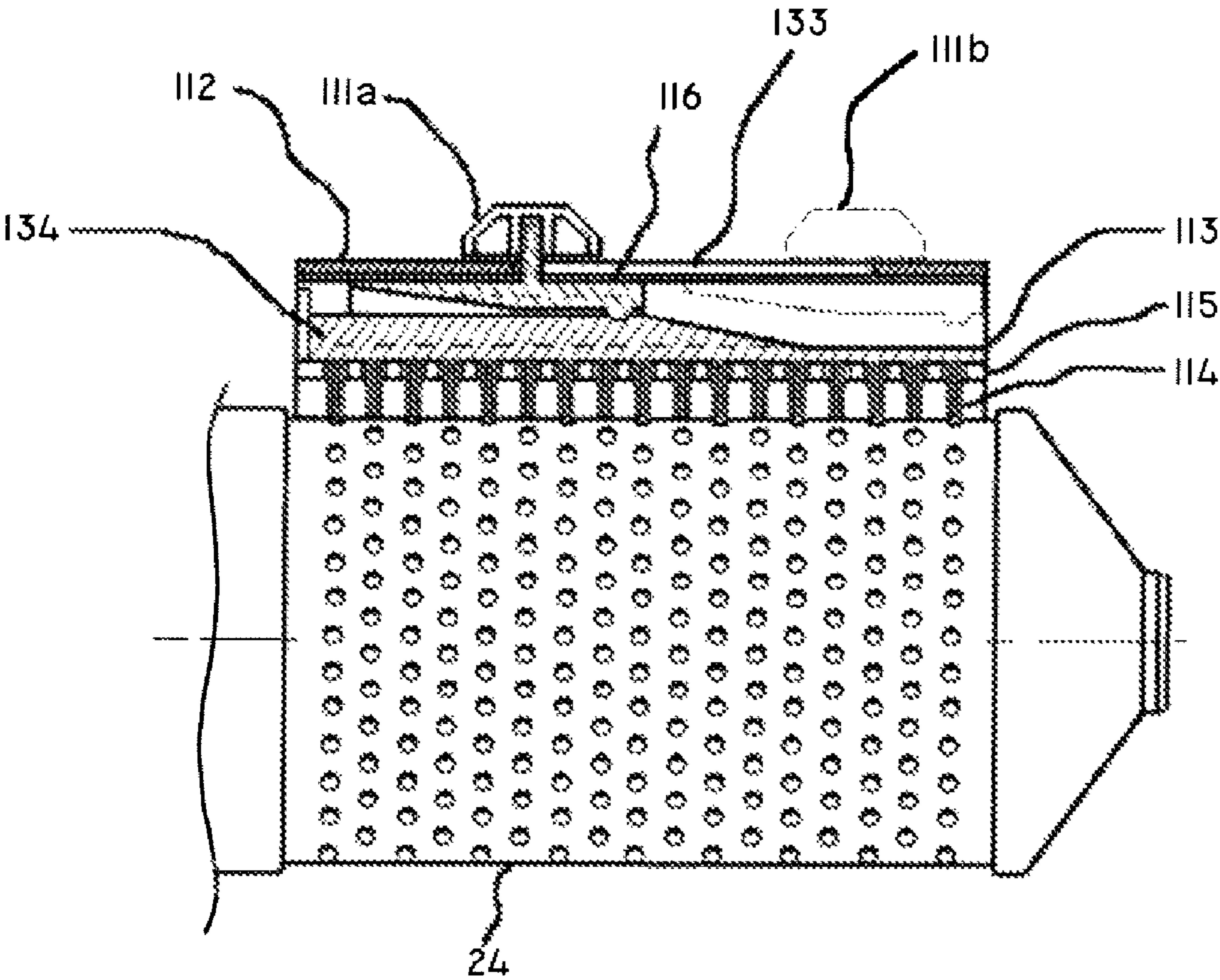
FIG. 9C
