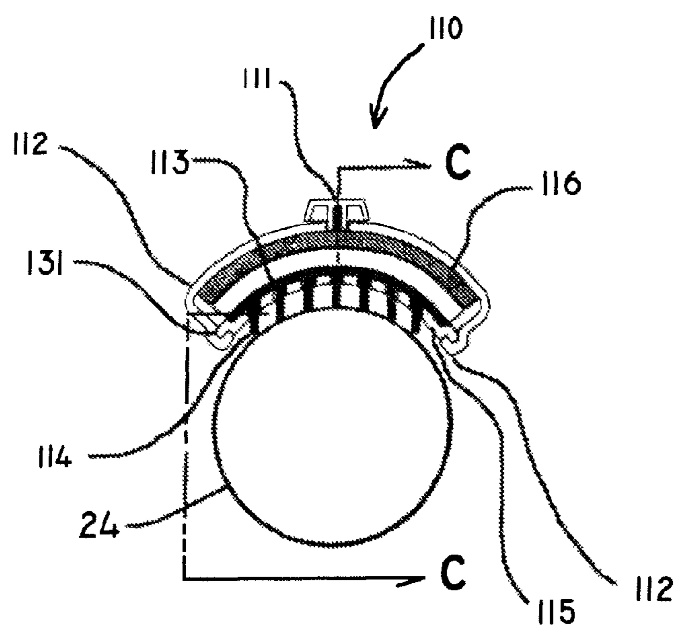
FIG. 9A
