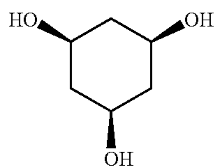
cis-1,3,5-Cyclohexanetriol
