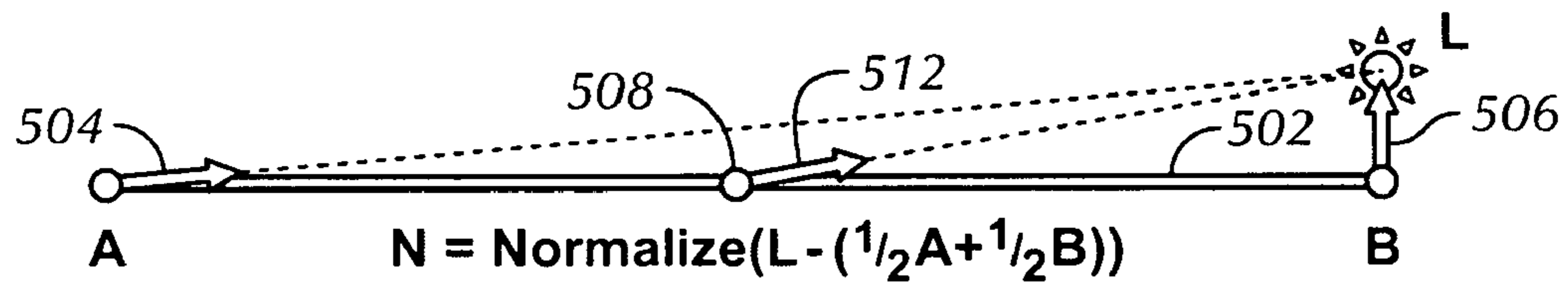
FIG. 5B
