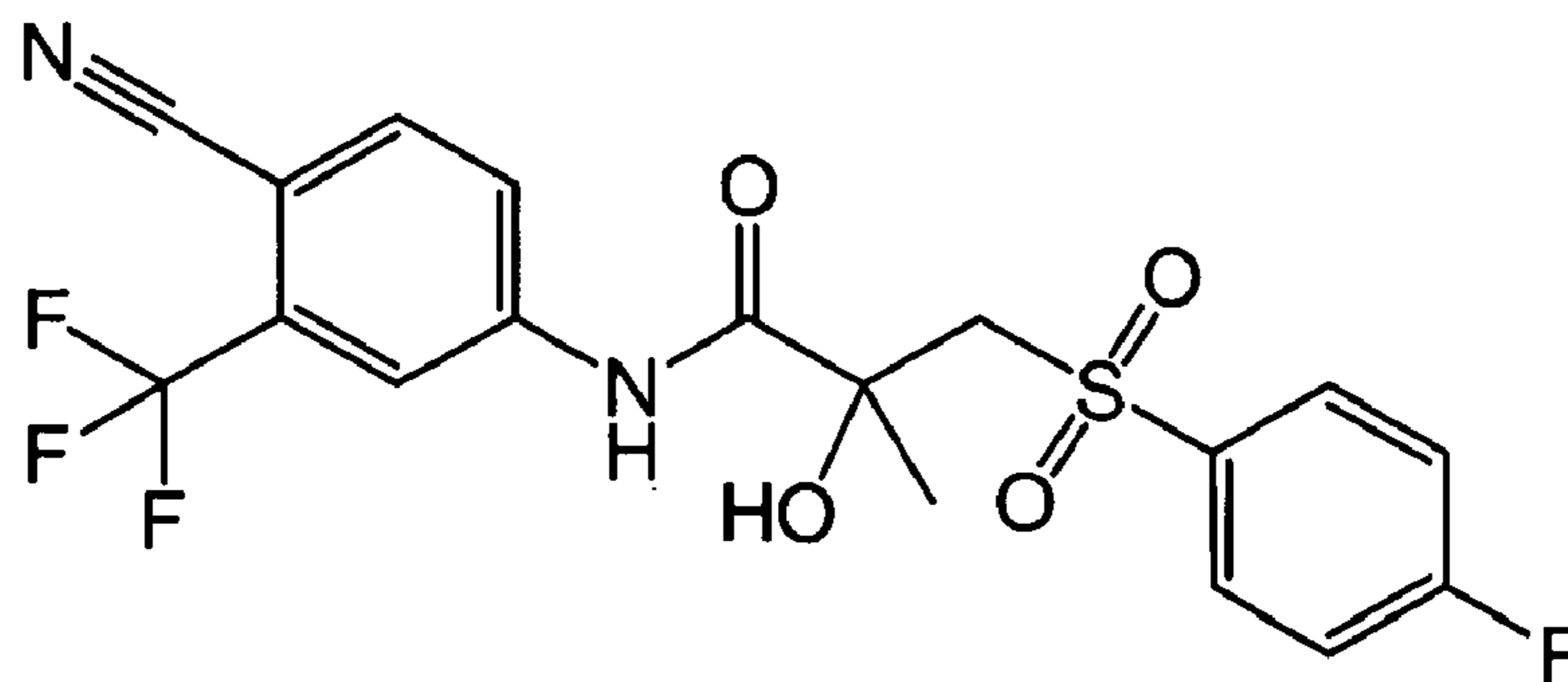
Bicalutamide (BiC)
