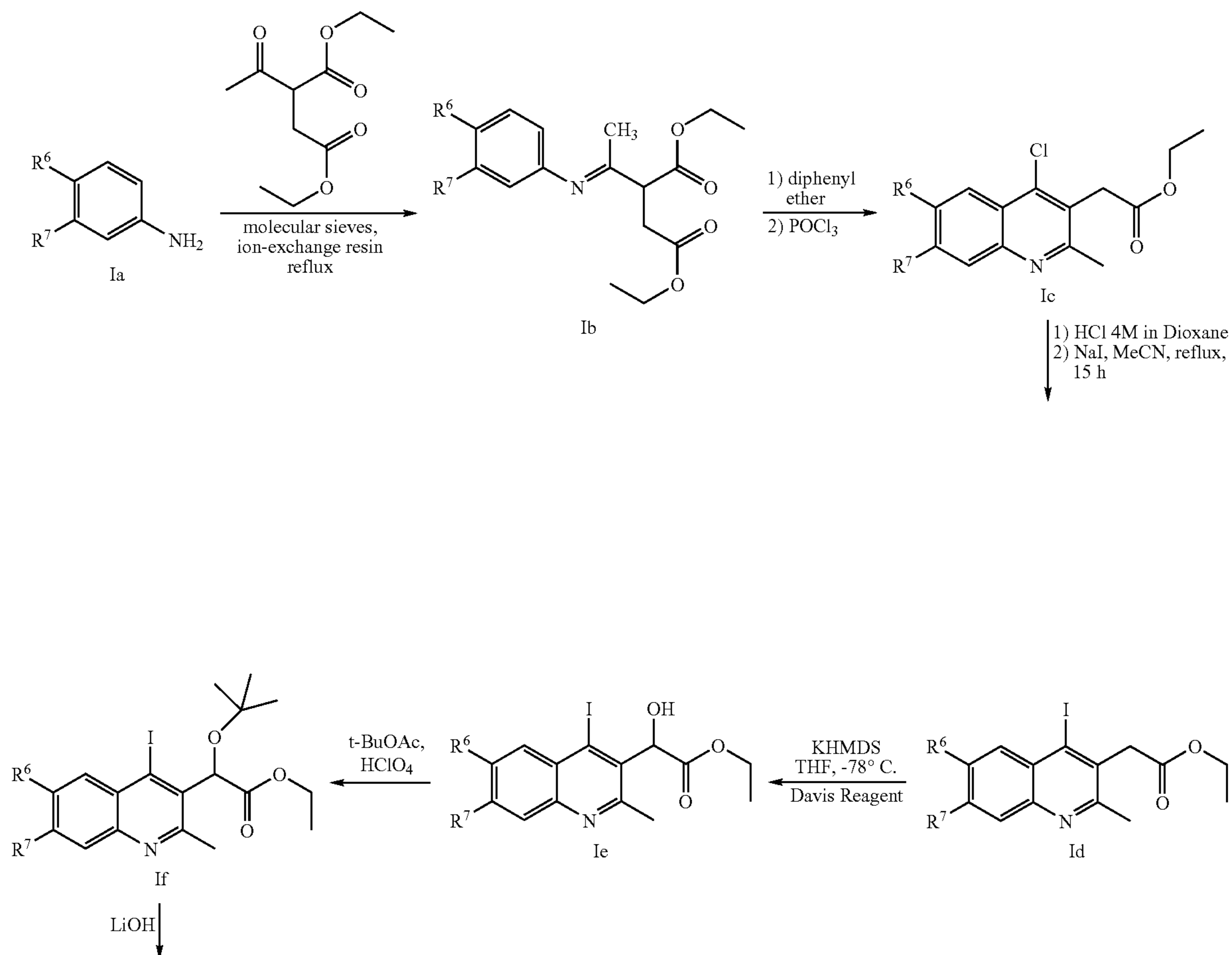
Scheme 1A
