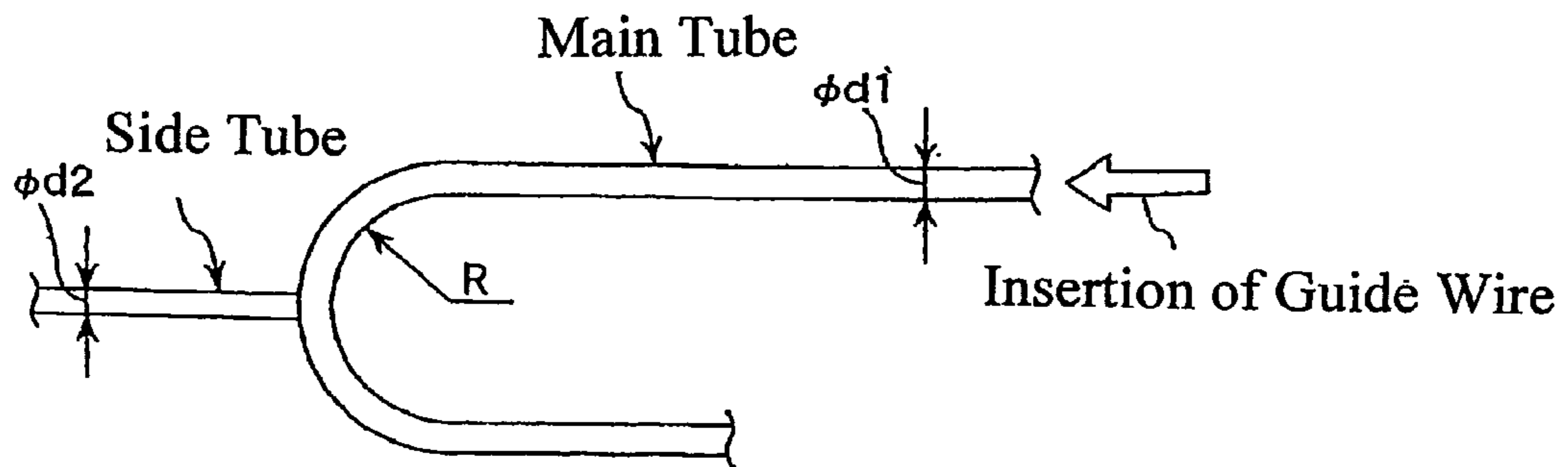
FIG. 18
