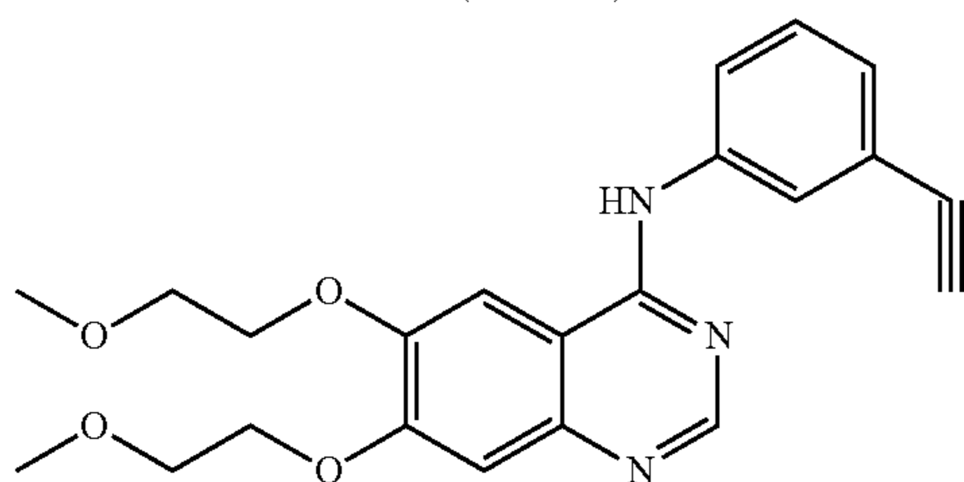
TARCEVA®
