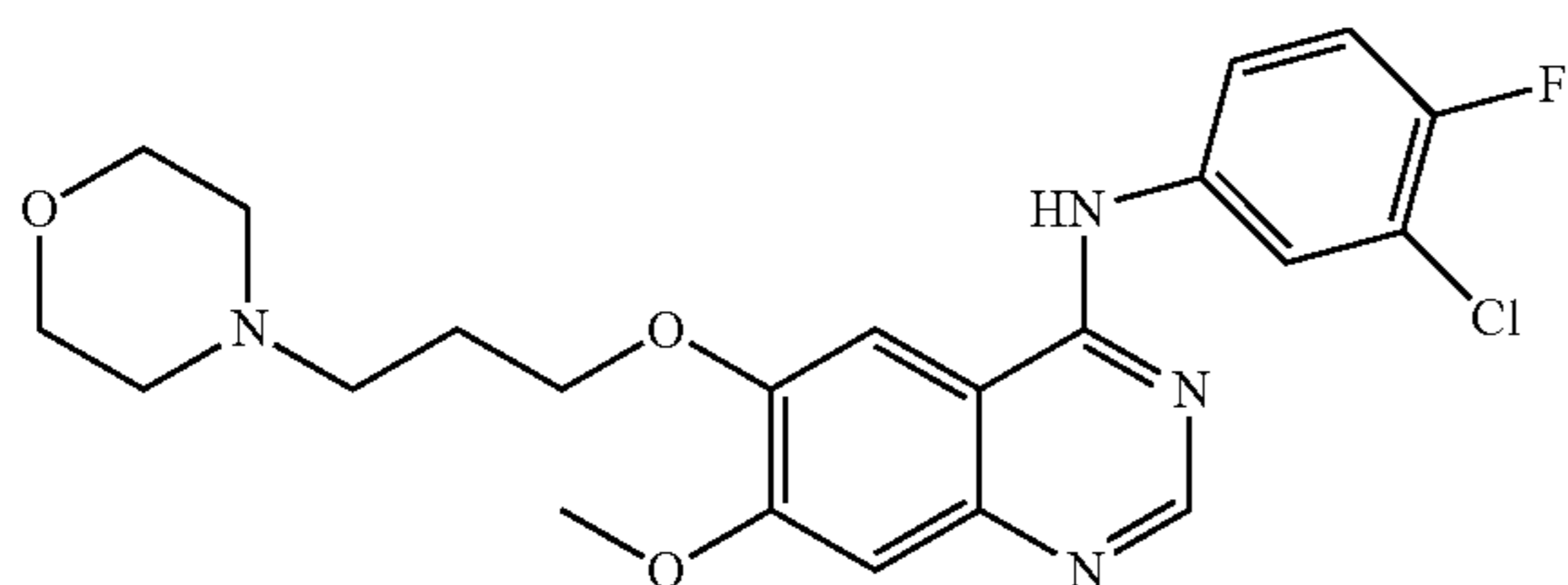
Iressa (ZD-1839)
