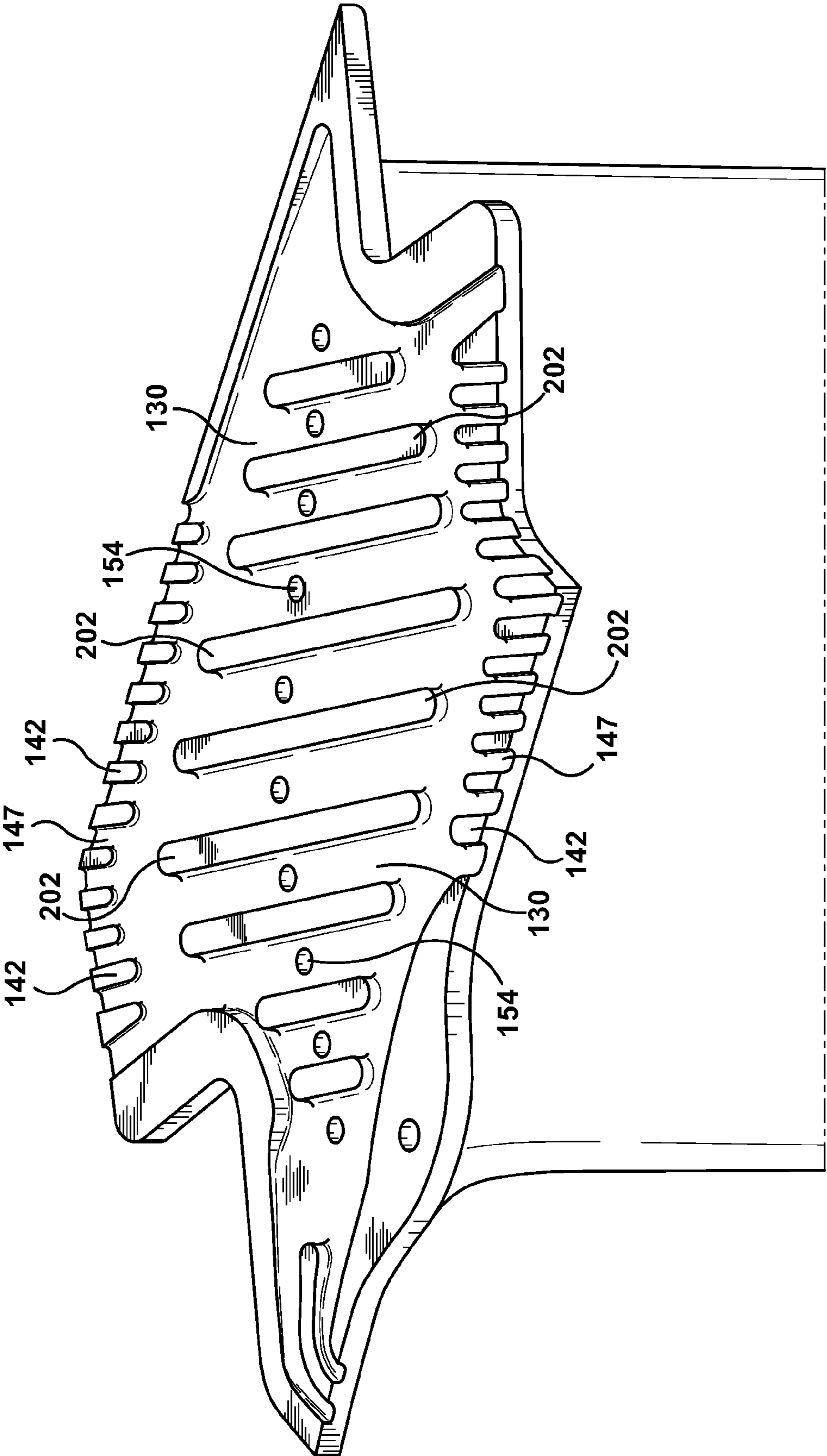
FIG. 6
