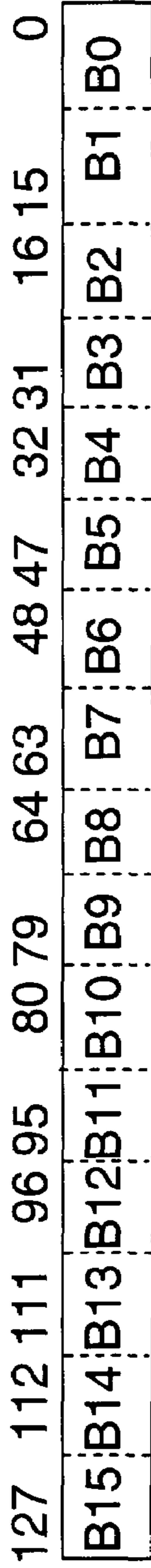
Packed Byte 421
