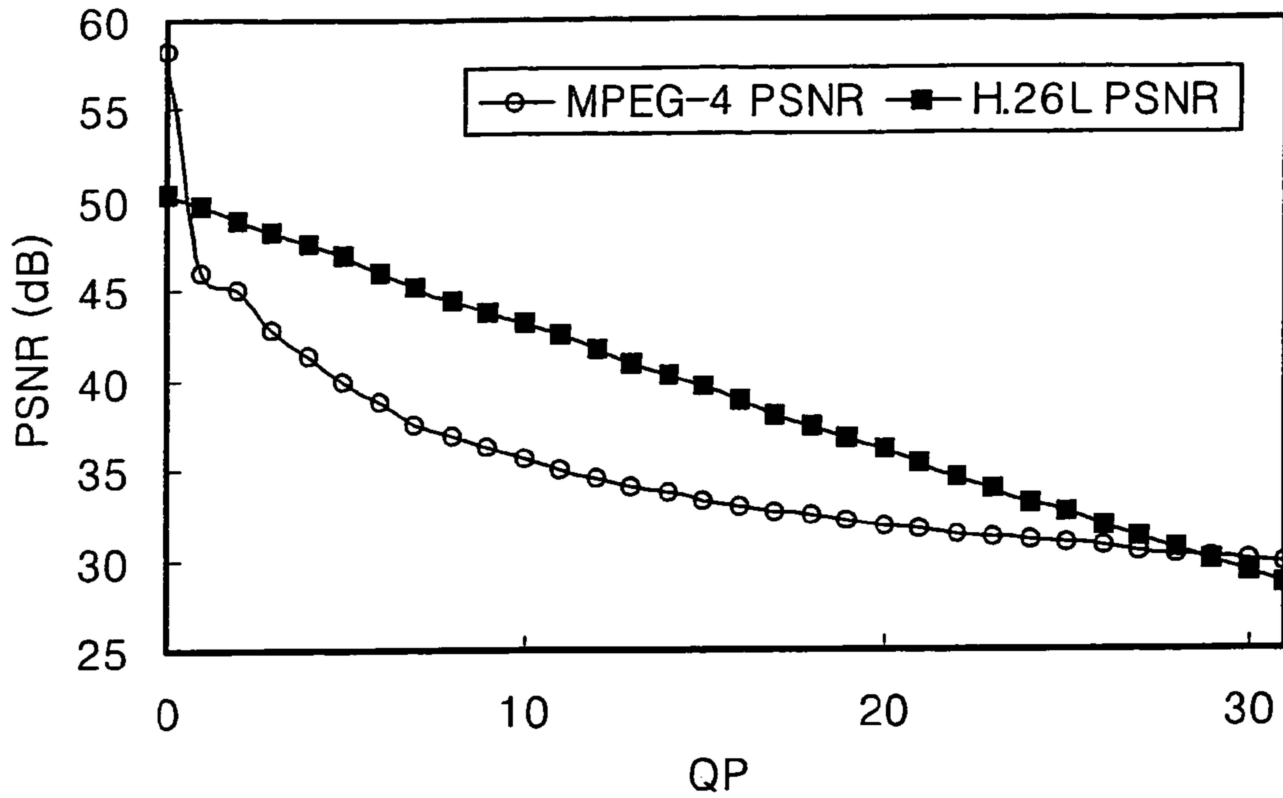
QP vs PSNR (Akiyo)
