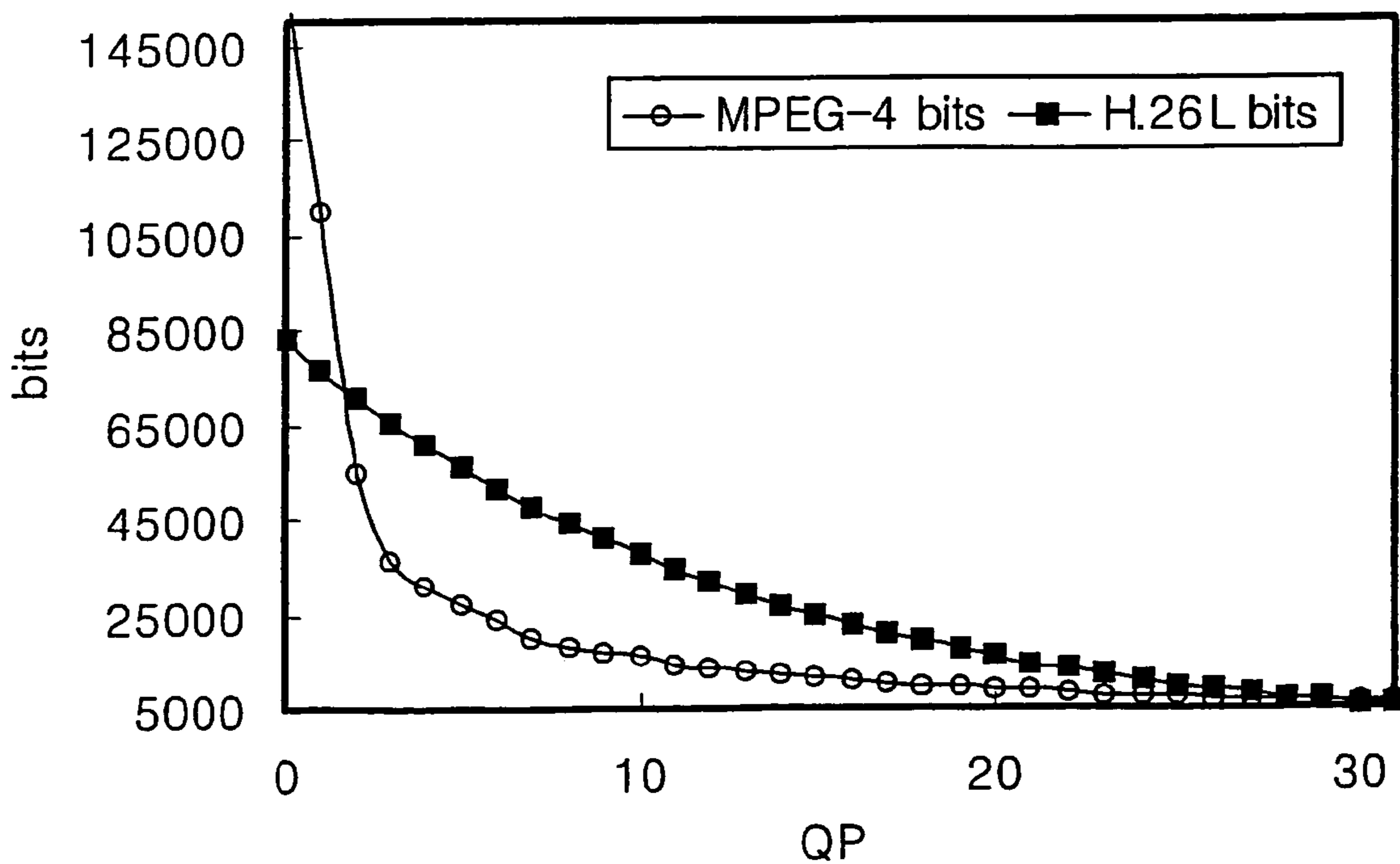
QP vs bits (Akiyo)
