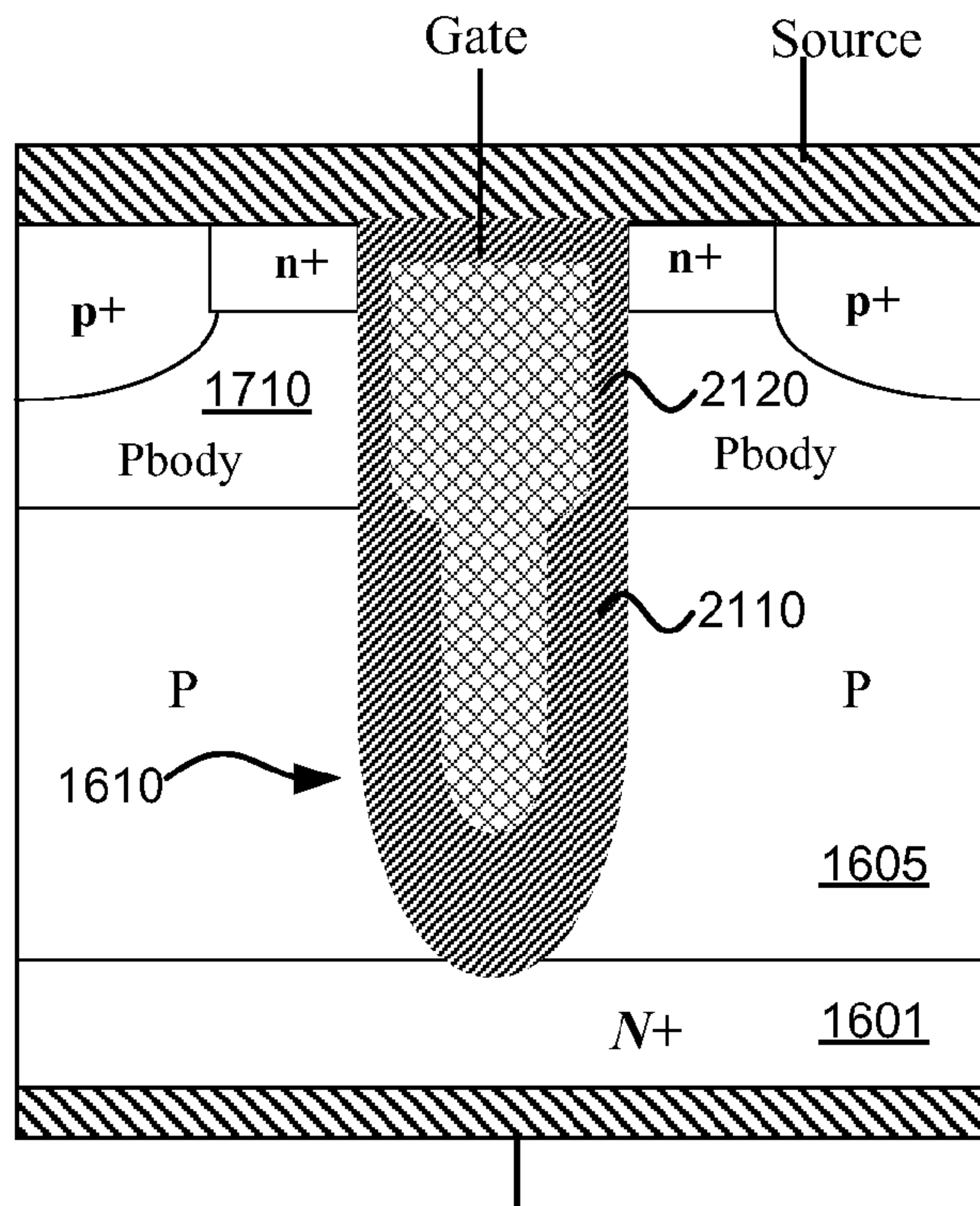
Drain FIG. 21A
