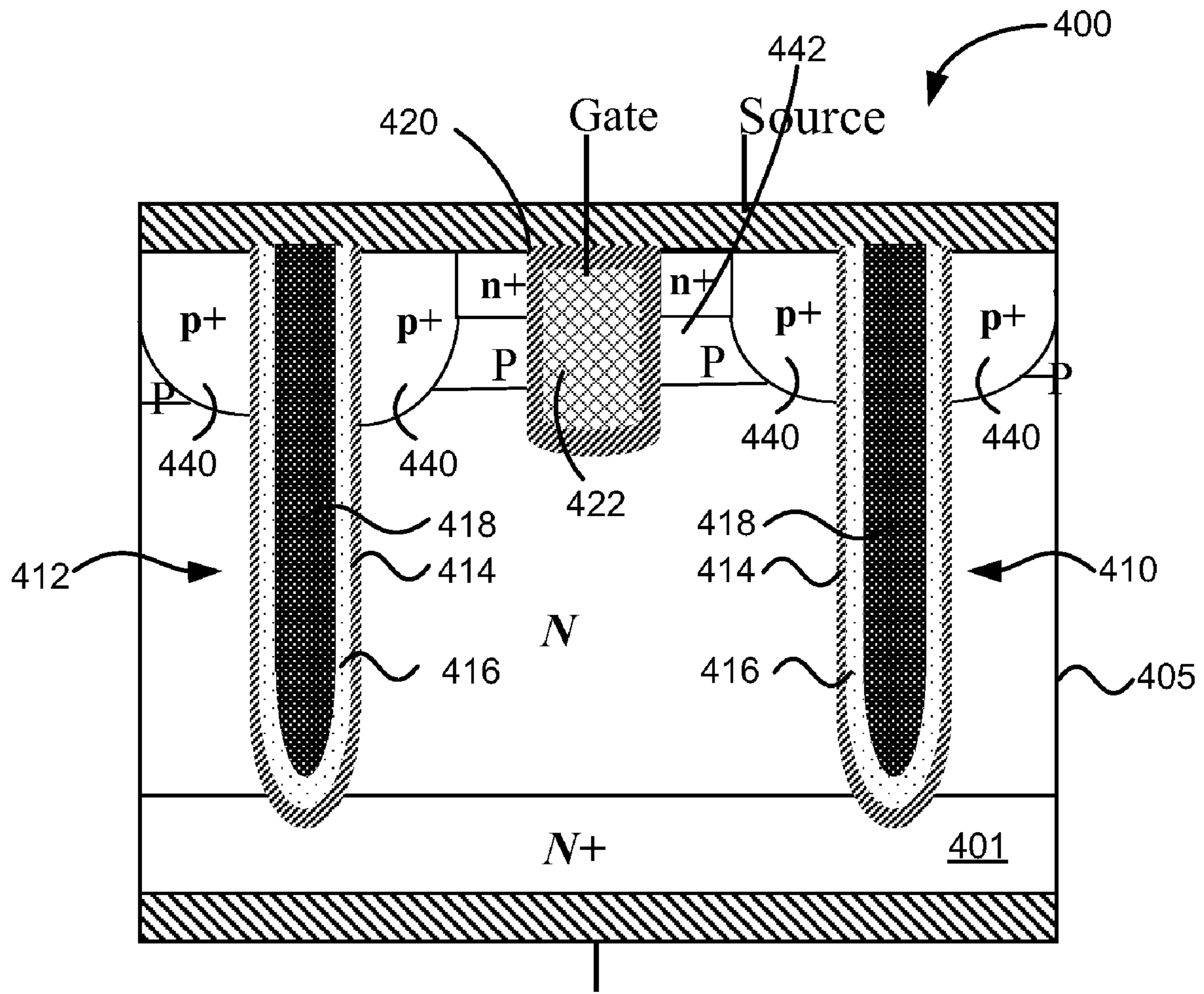
Drain FIG. 4
