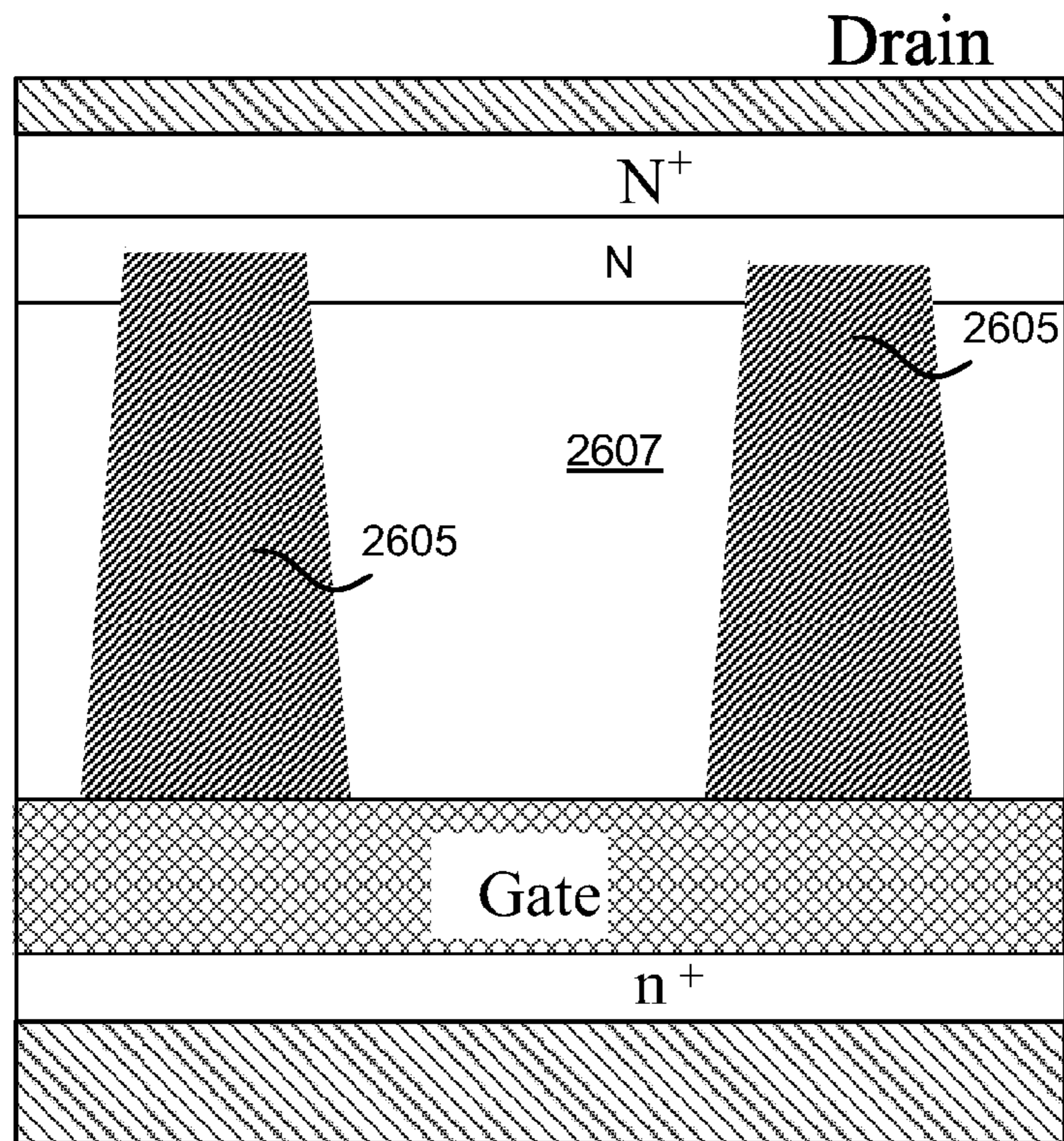
FIG. 26H Source
