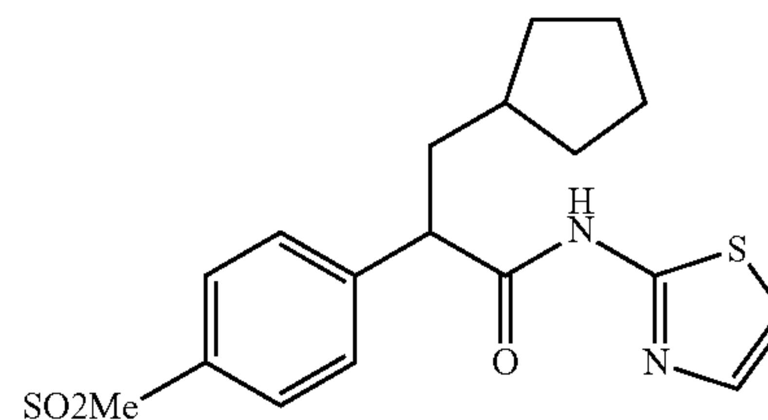
Ro-28-1675
