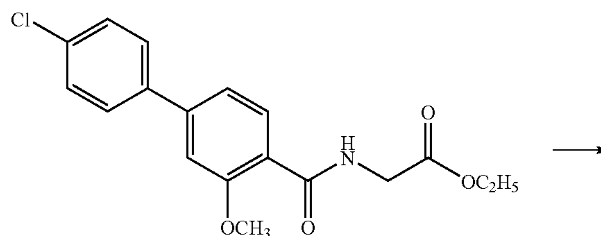
Scheme VI
