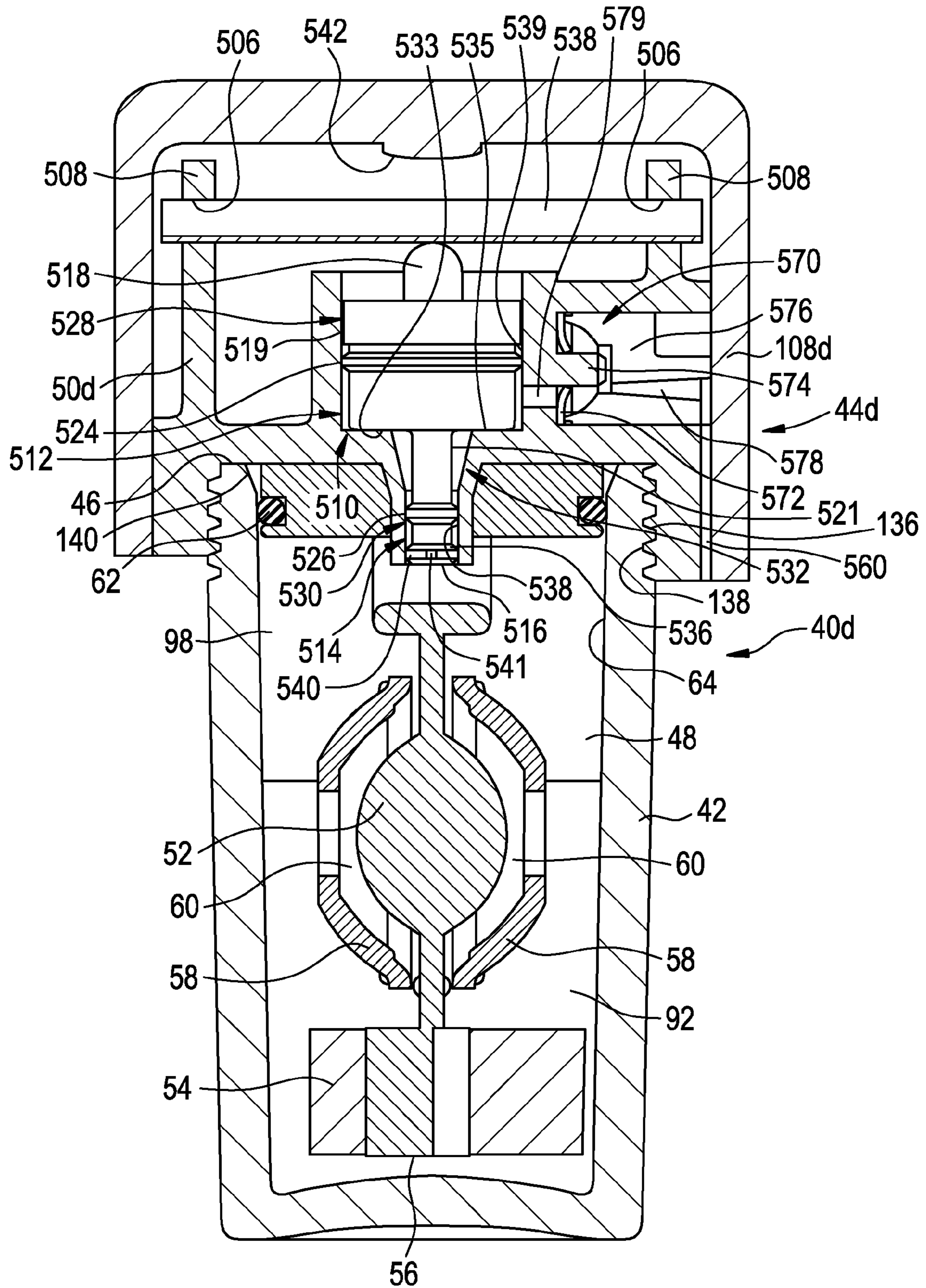
FIG. 22
