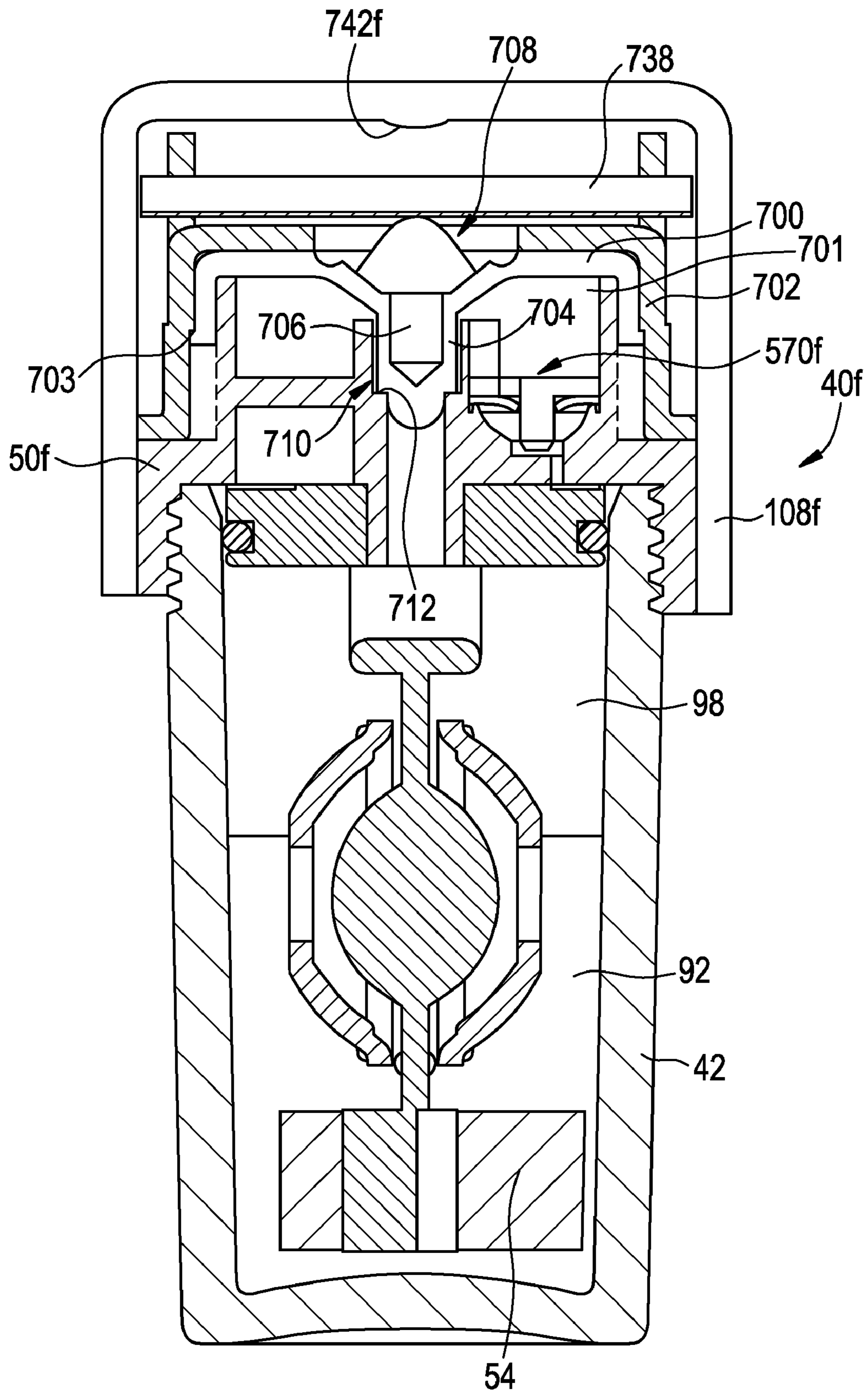
FIG. 27
