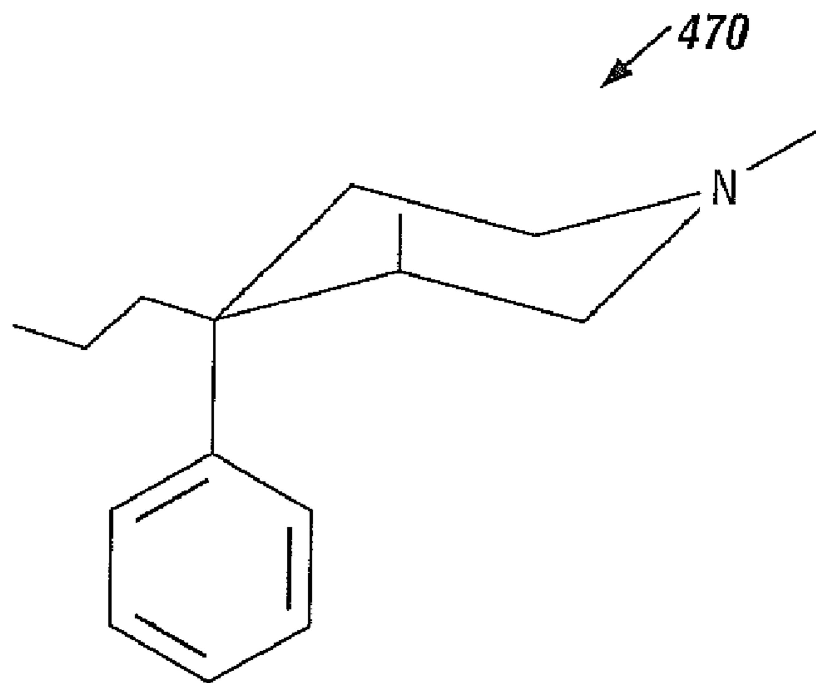
Picenadol (-) Isomer
