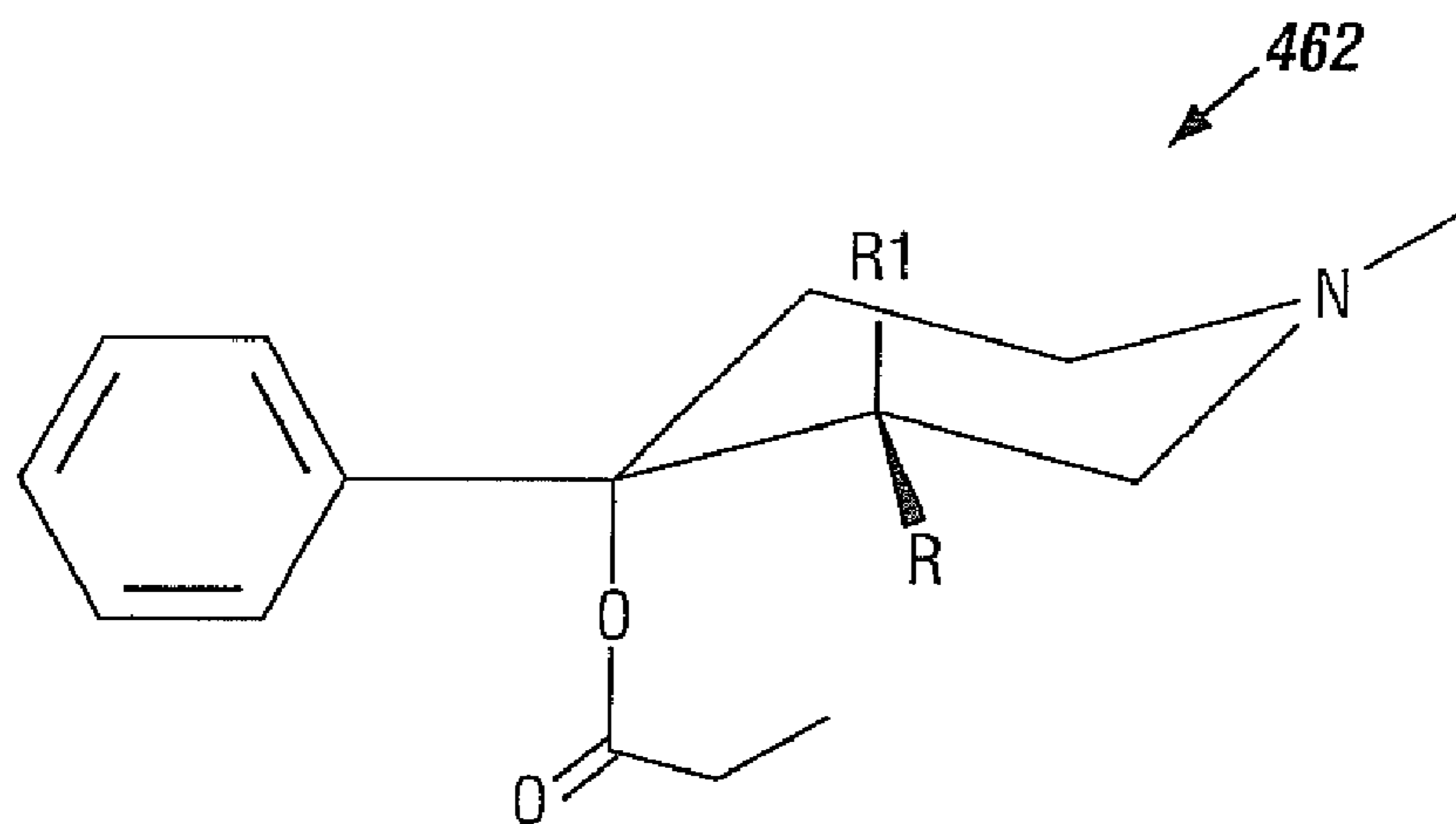
Prodine (-) Isomer
