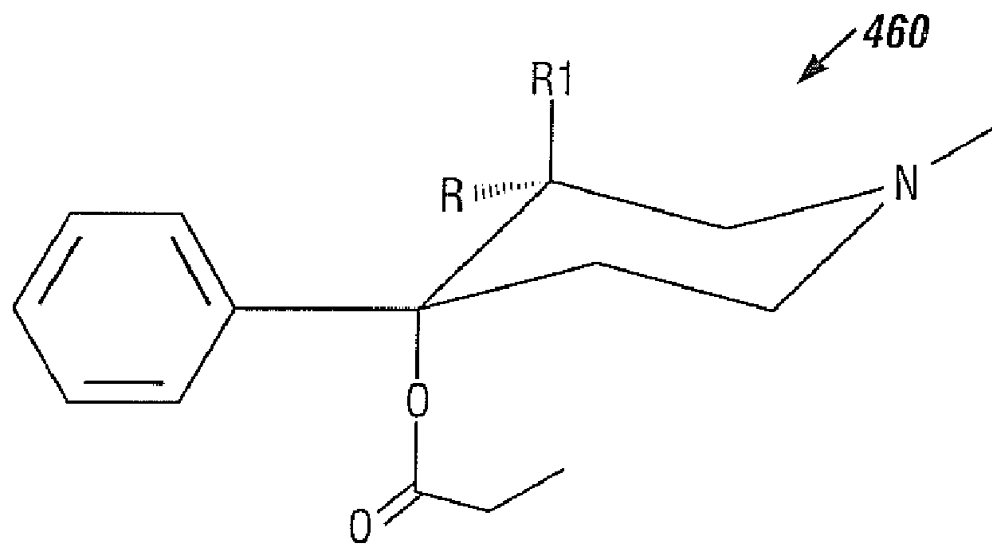
Prodine (+) Isomer
