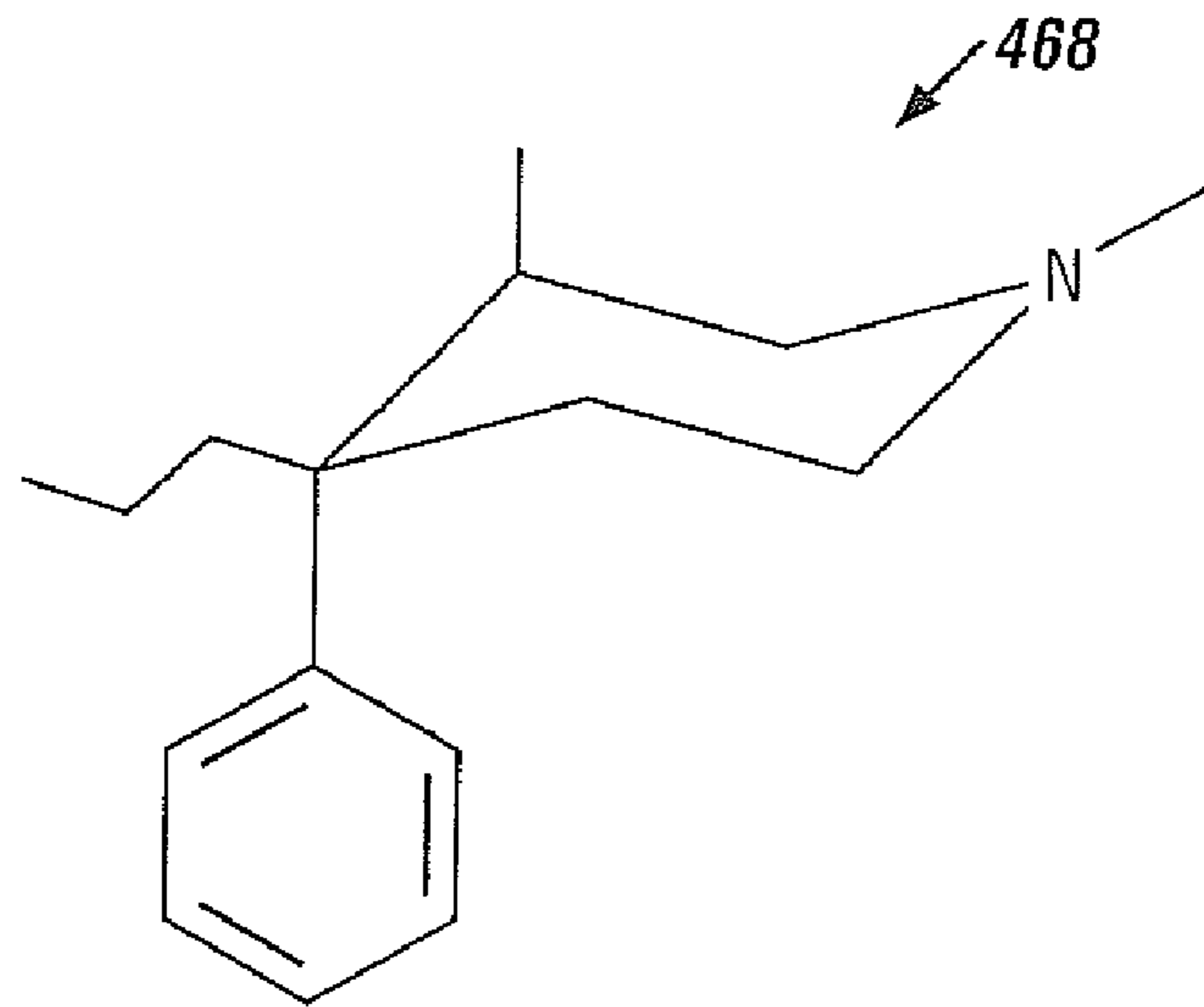
Picenadol (+) Isomer
