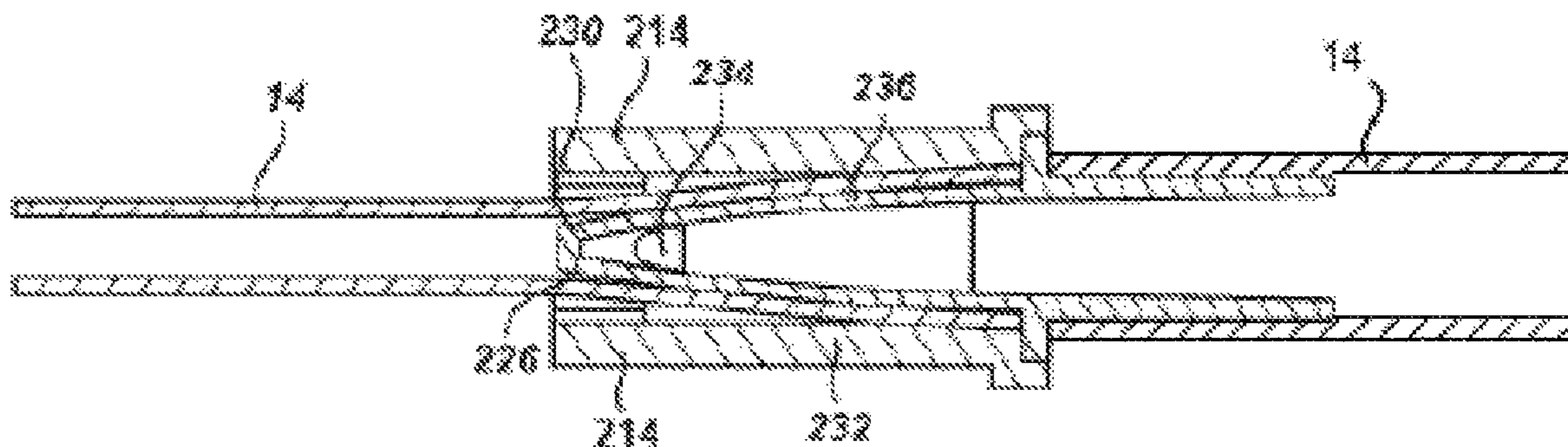
SECTION A-A
