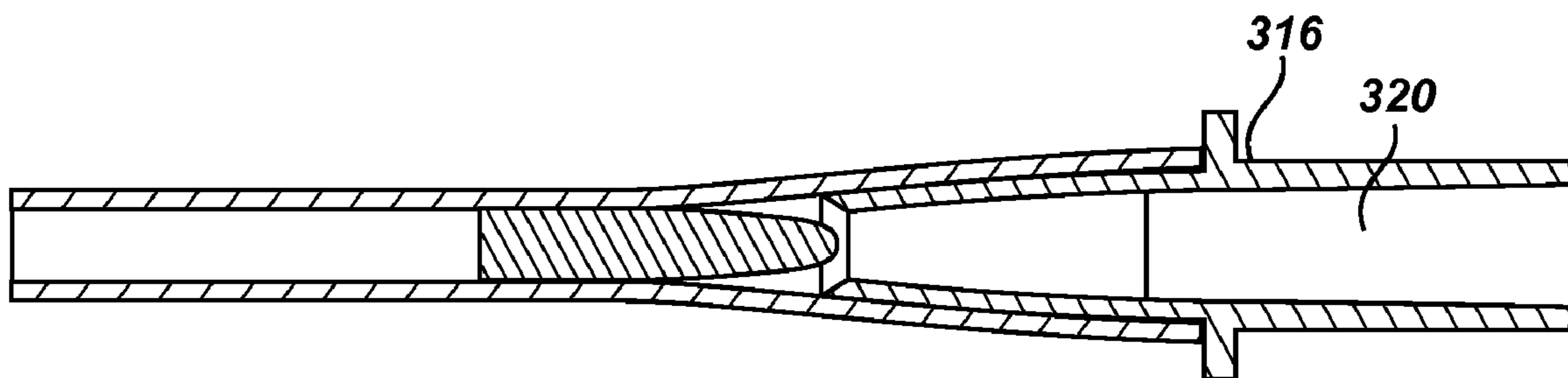
SECTION A-A
