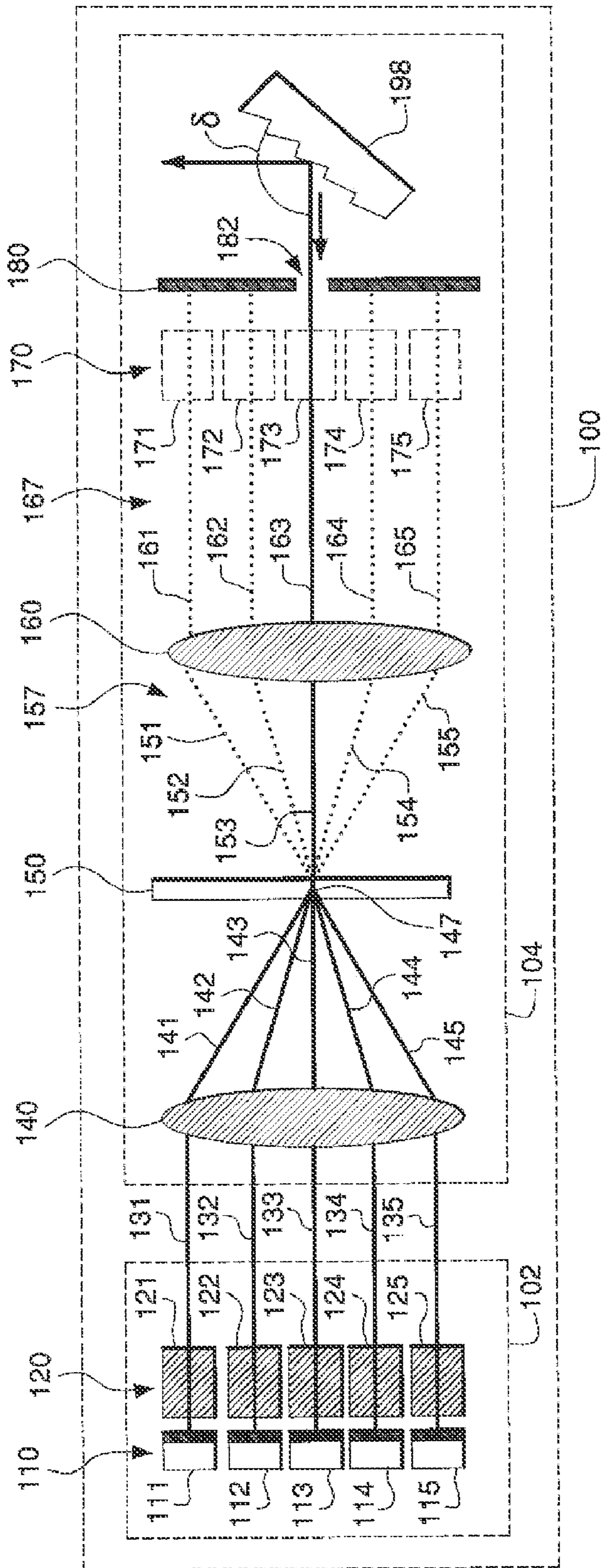
FIG. 3B
