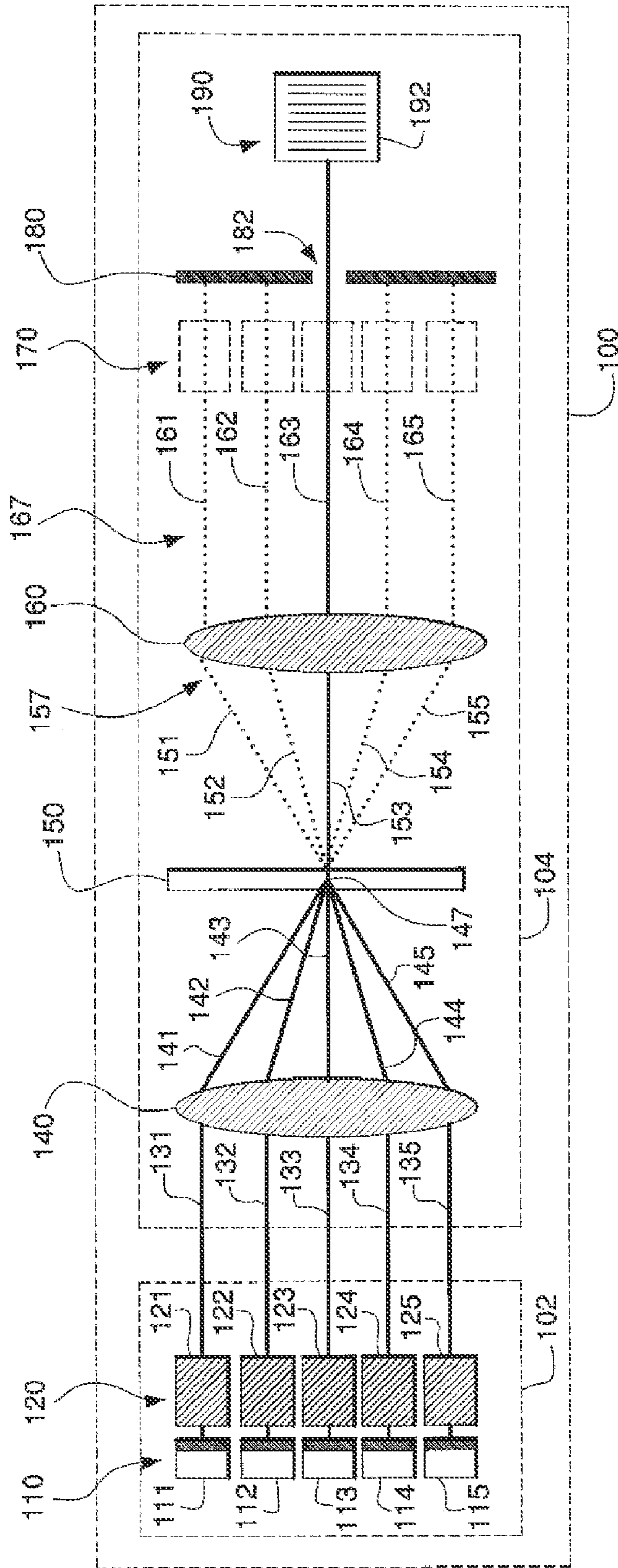
FIG. 1A
