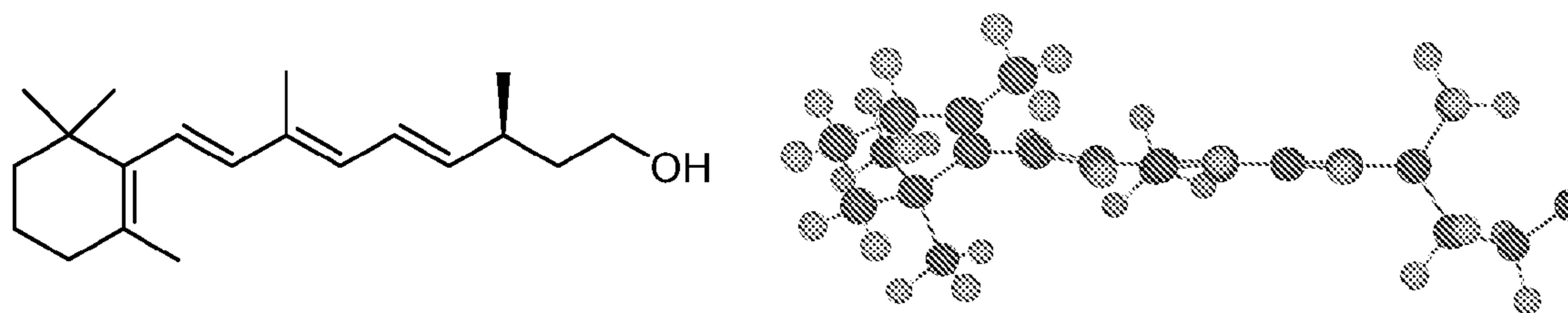
(13 S )-all-trans-13,14-dihydroretinol
