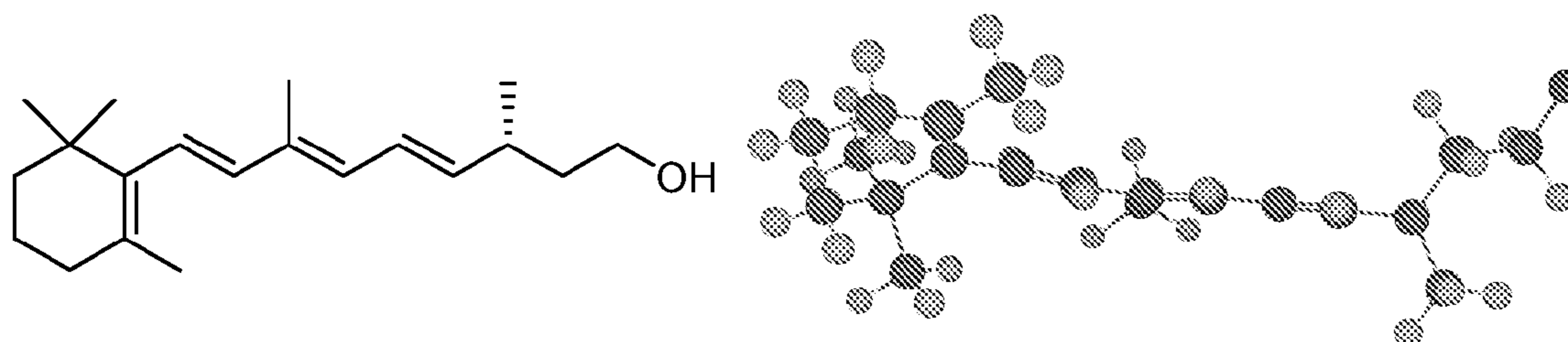
(13 R )-all-trans-13,14-dihydroretinol
