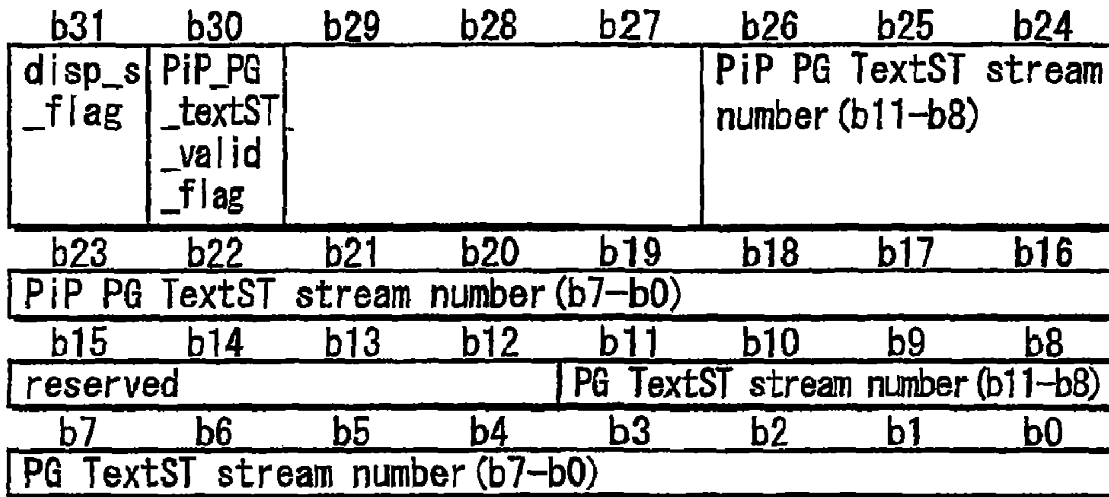
FIG. 48B
