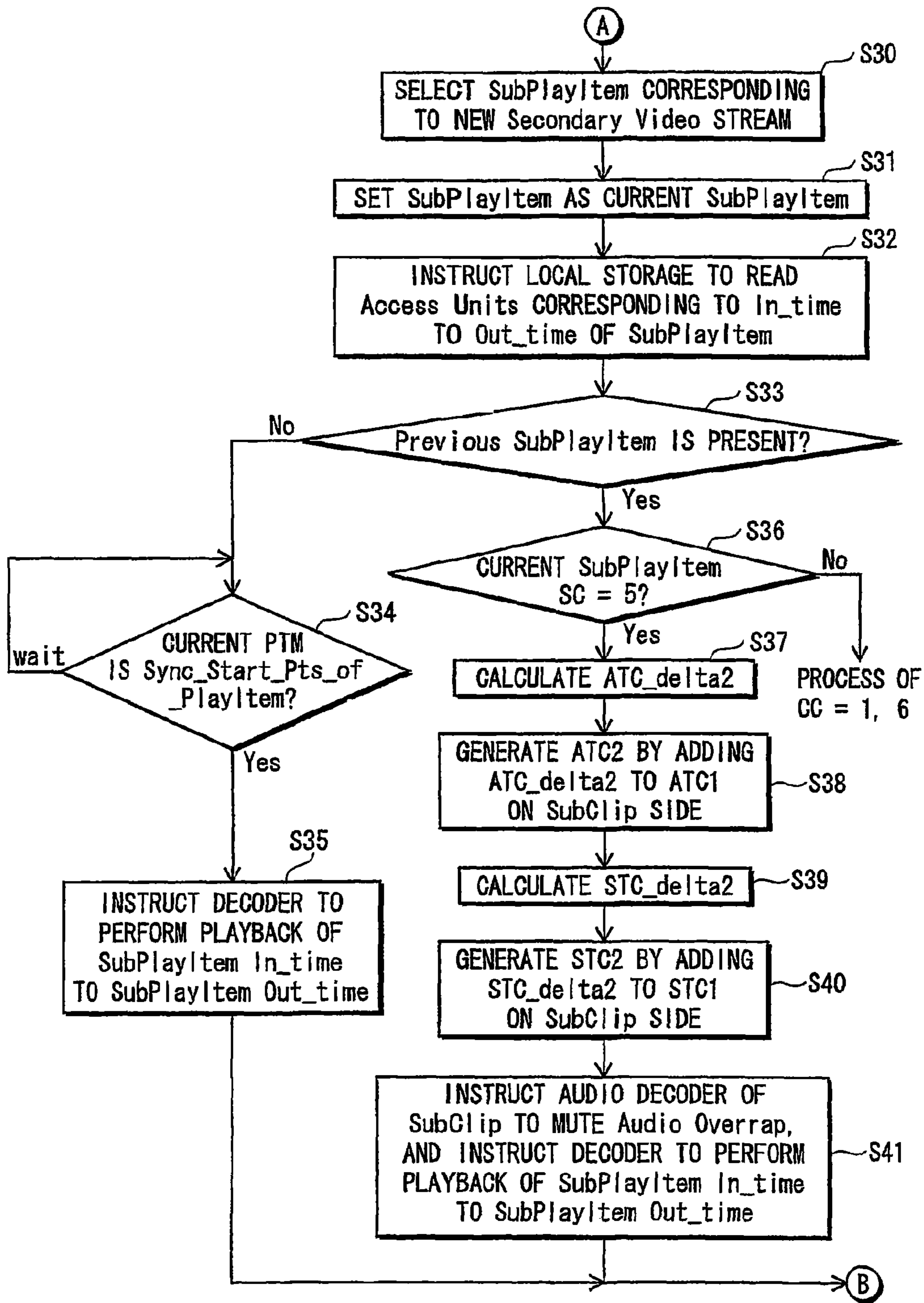
FIG. 39
