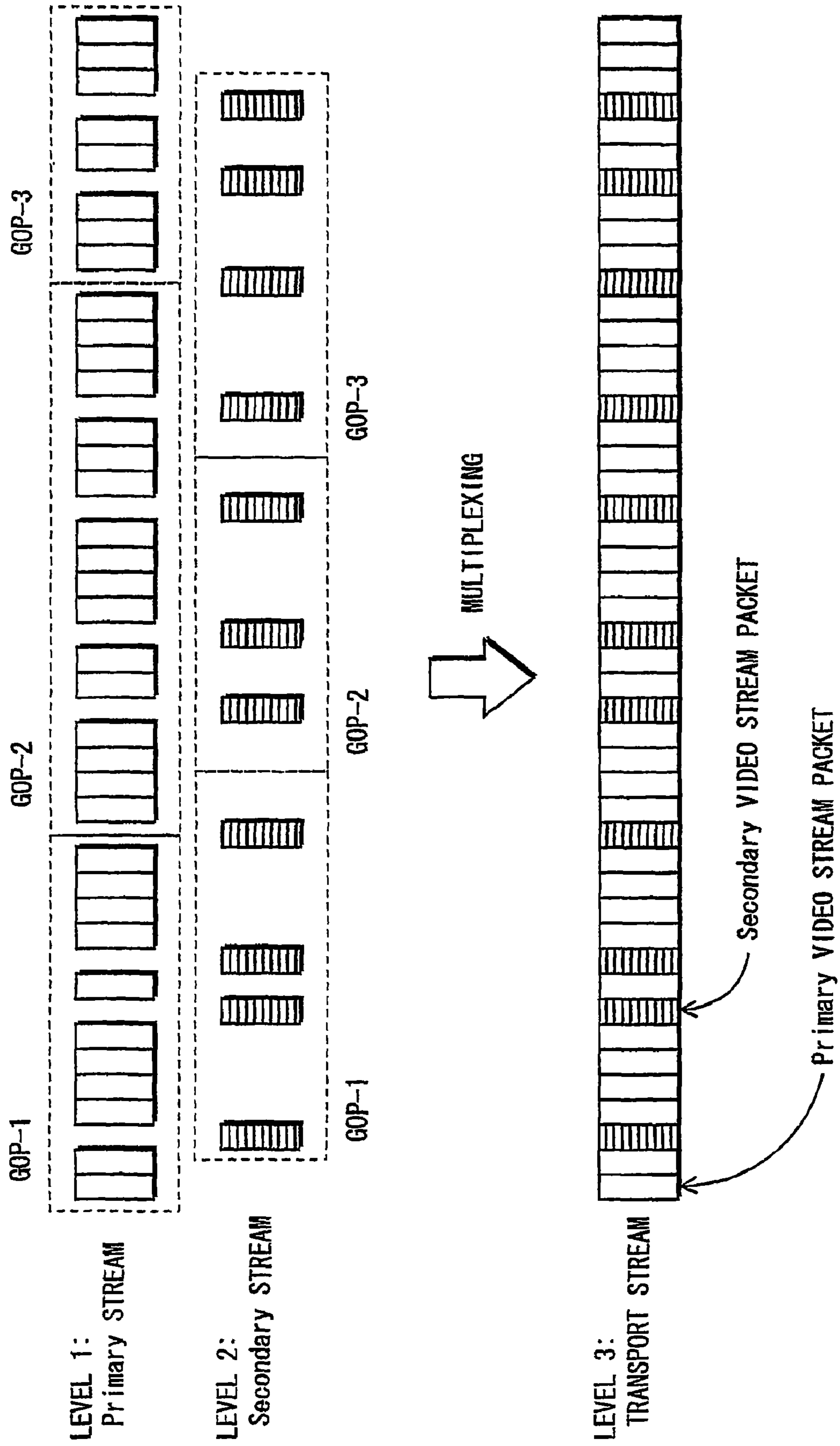
FIG. 55
