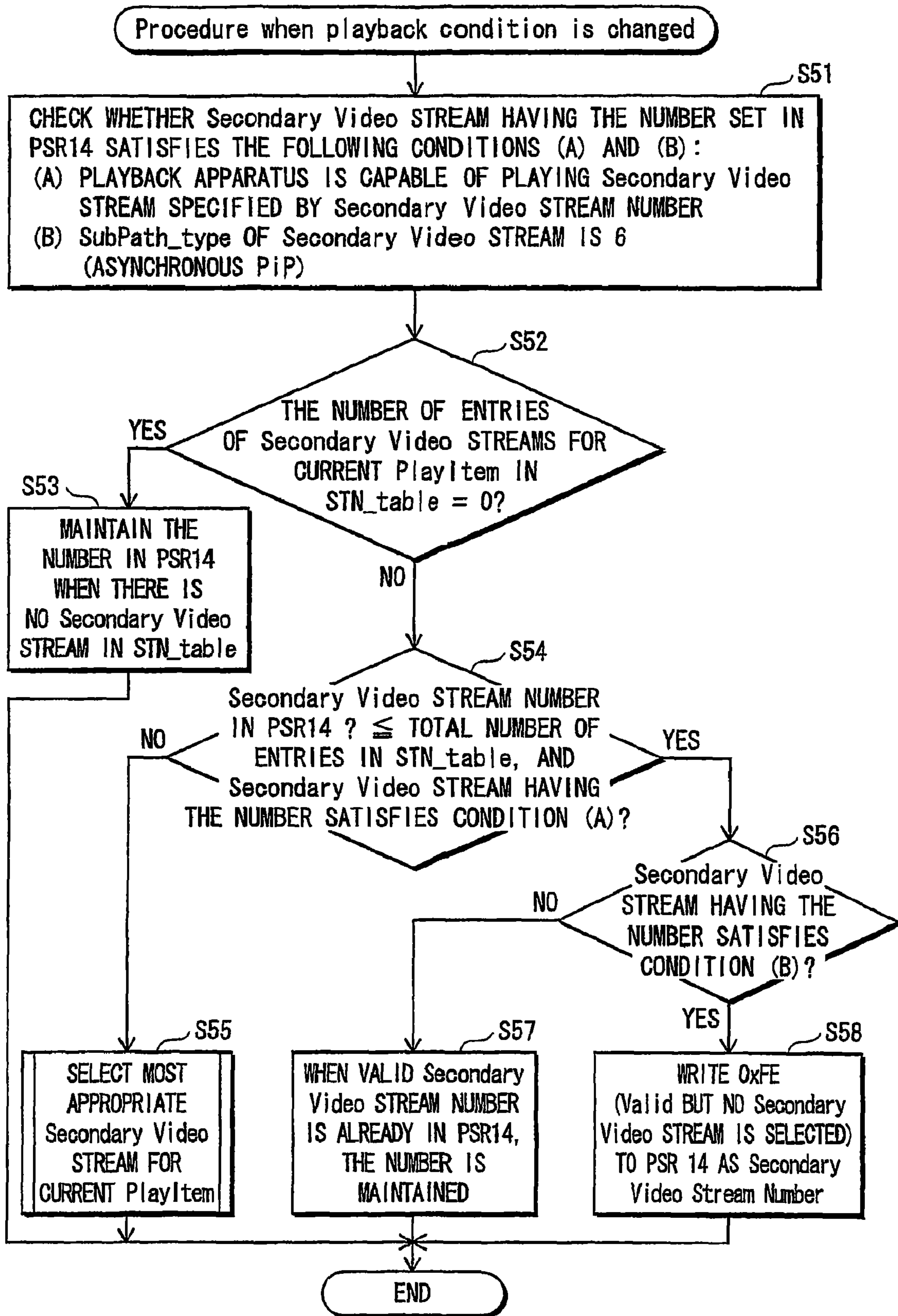
FIG. 27
