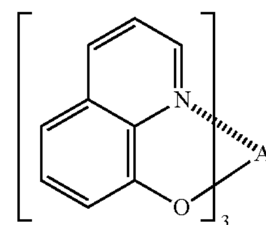
Alq 3
