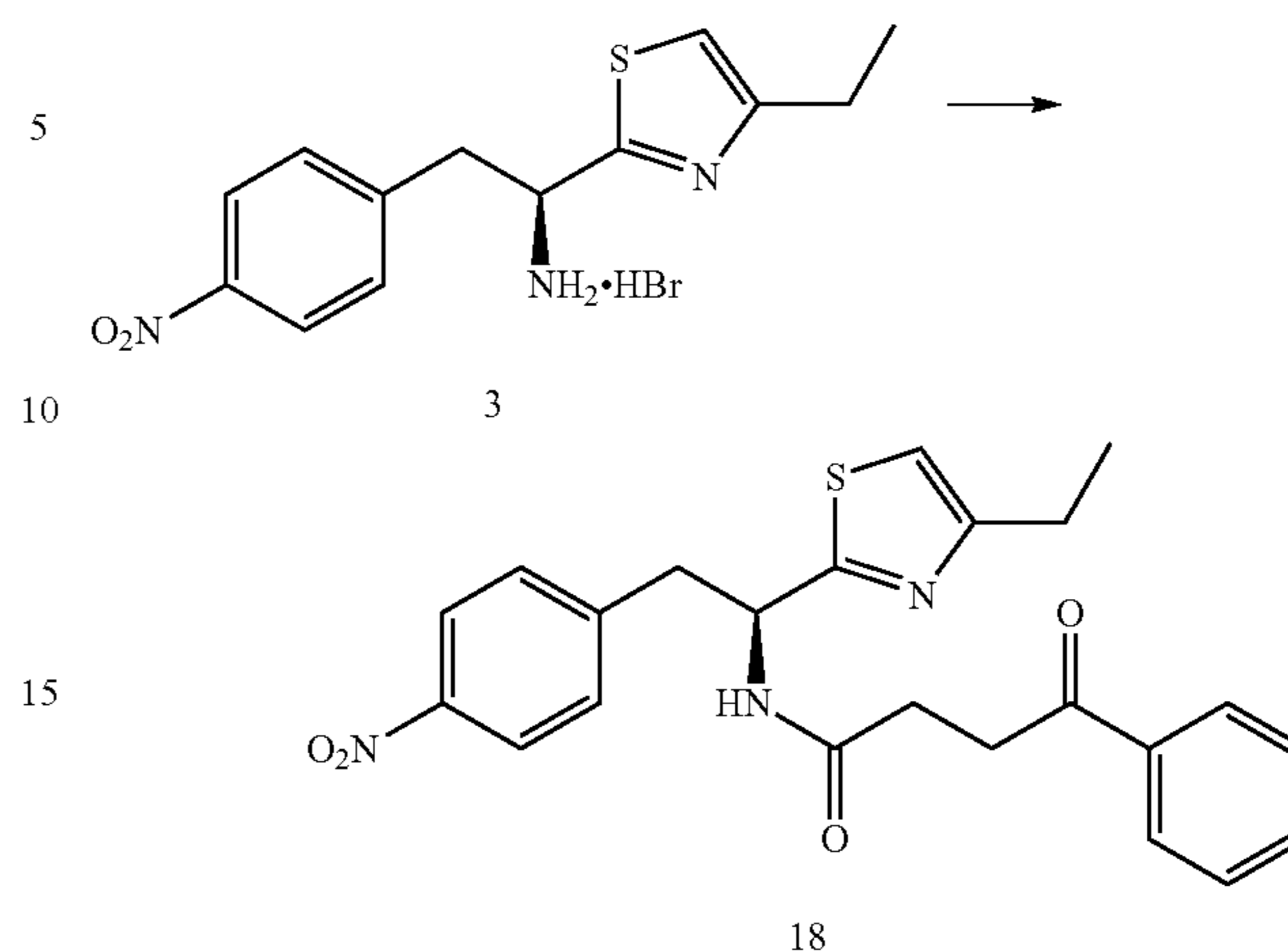
Scheme VI
