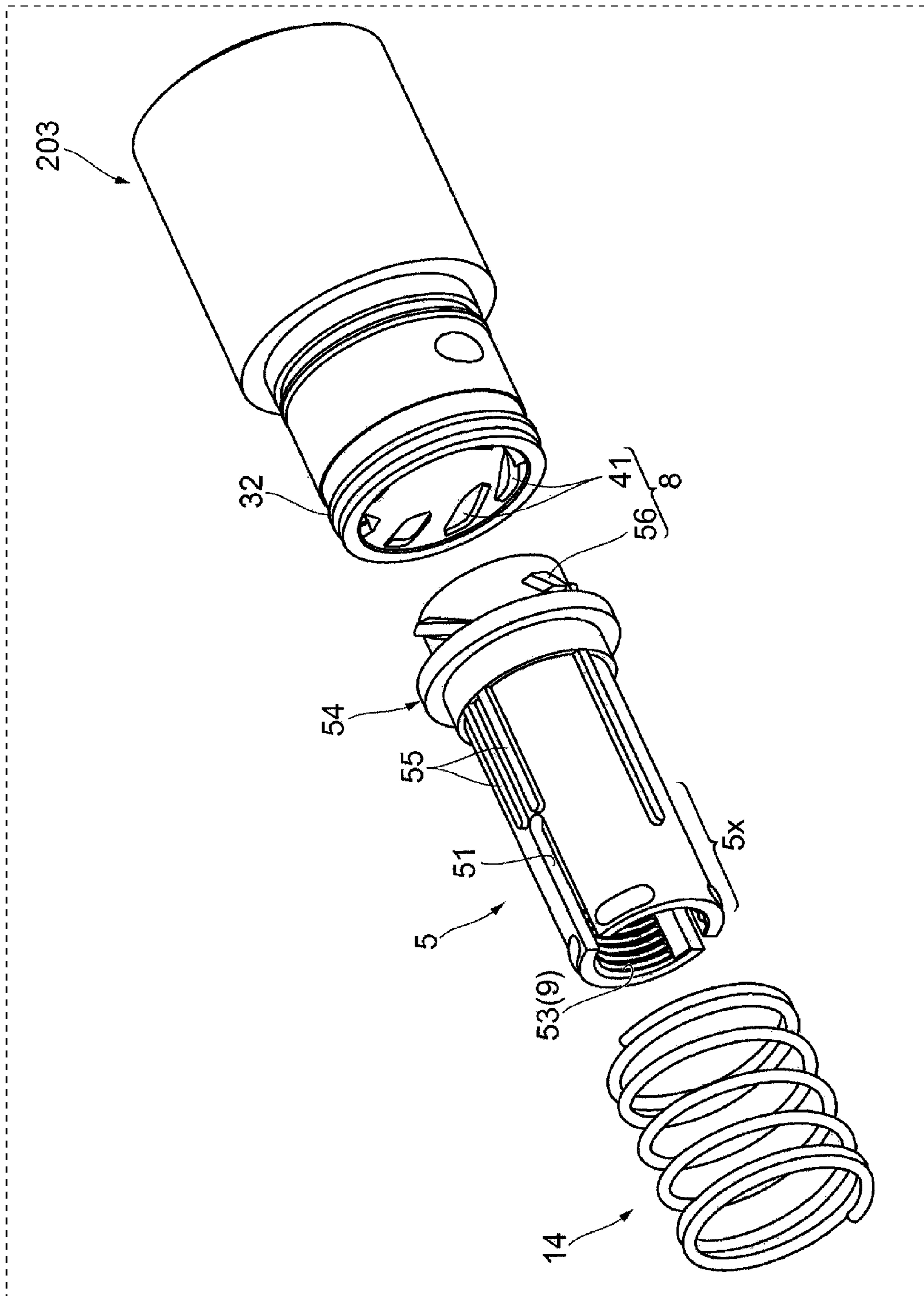
FIG.16
