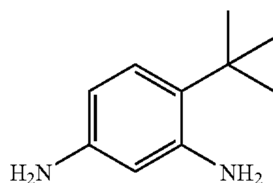
D-9; 4-tert-Butylbenzene-1,3-diamine
