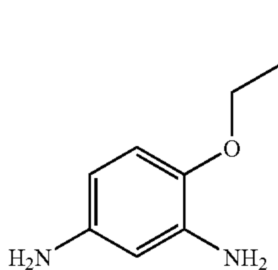
D-5; 4-Propoxybenzene-1,3-diamine
