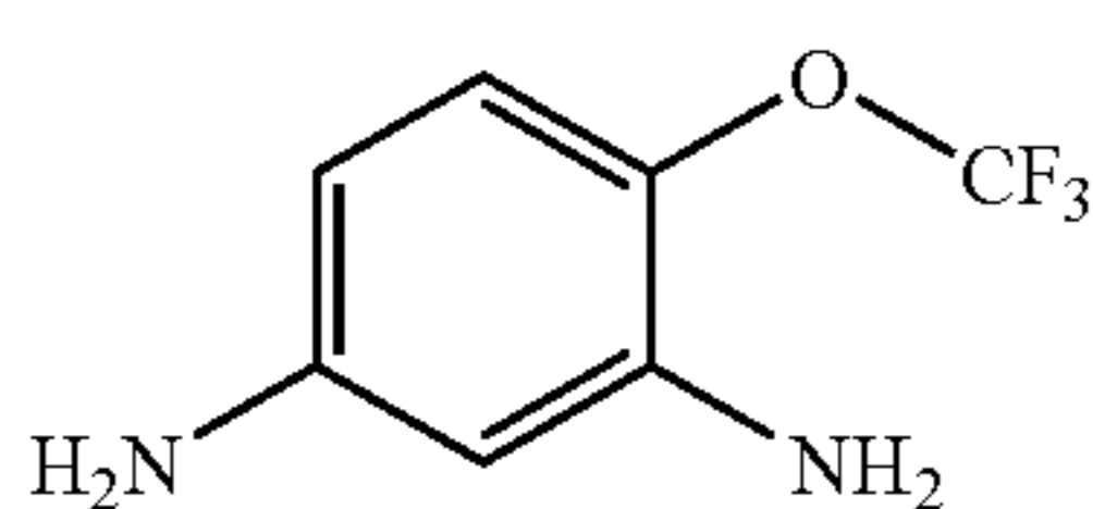
D-4; 4-Trifluoromethoxy-benzene-1,3-diamine
