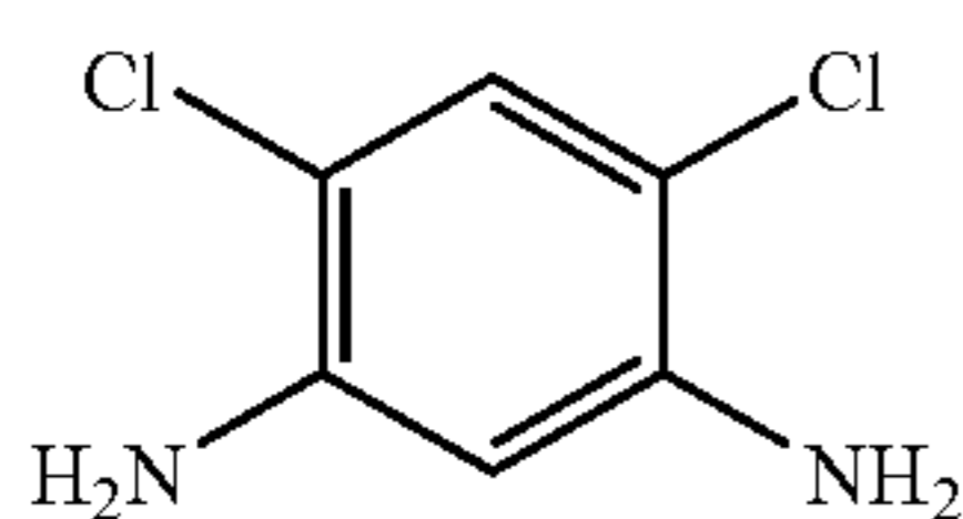
D-2; 4,6-Dichloro-benzene-1,3-diamine
