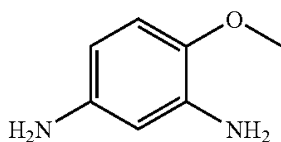
D-3; 4-Methoxy-benzene-1,3-diamine
