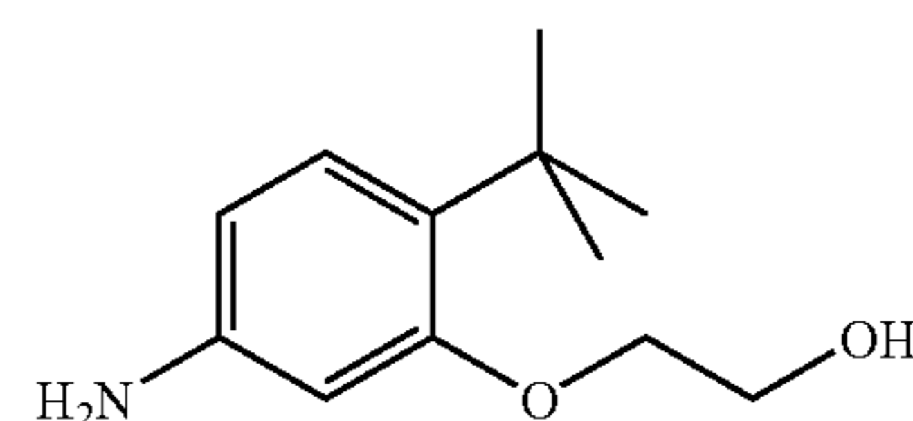
C-4; 2-(2-tert-Butyl-5-aminophenoxy)ethanol
