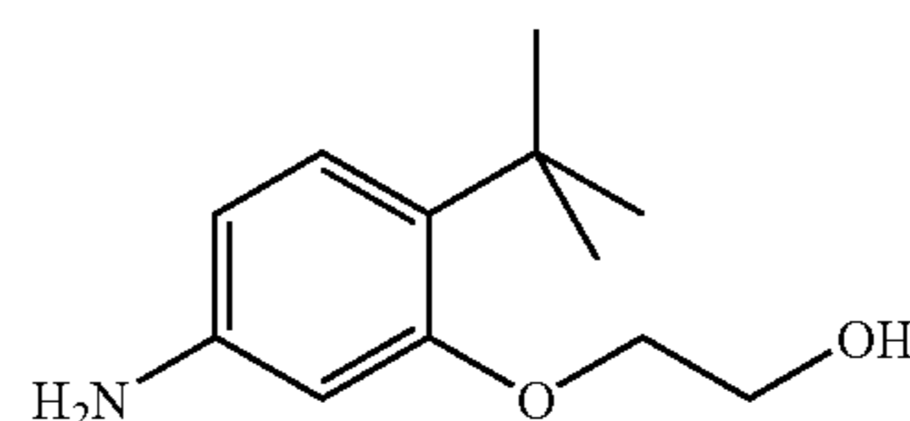
C-4; 2-(2-tert-Butyl-5-aminophenoxy)ethanol
