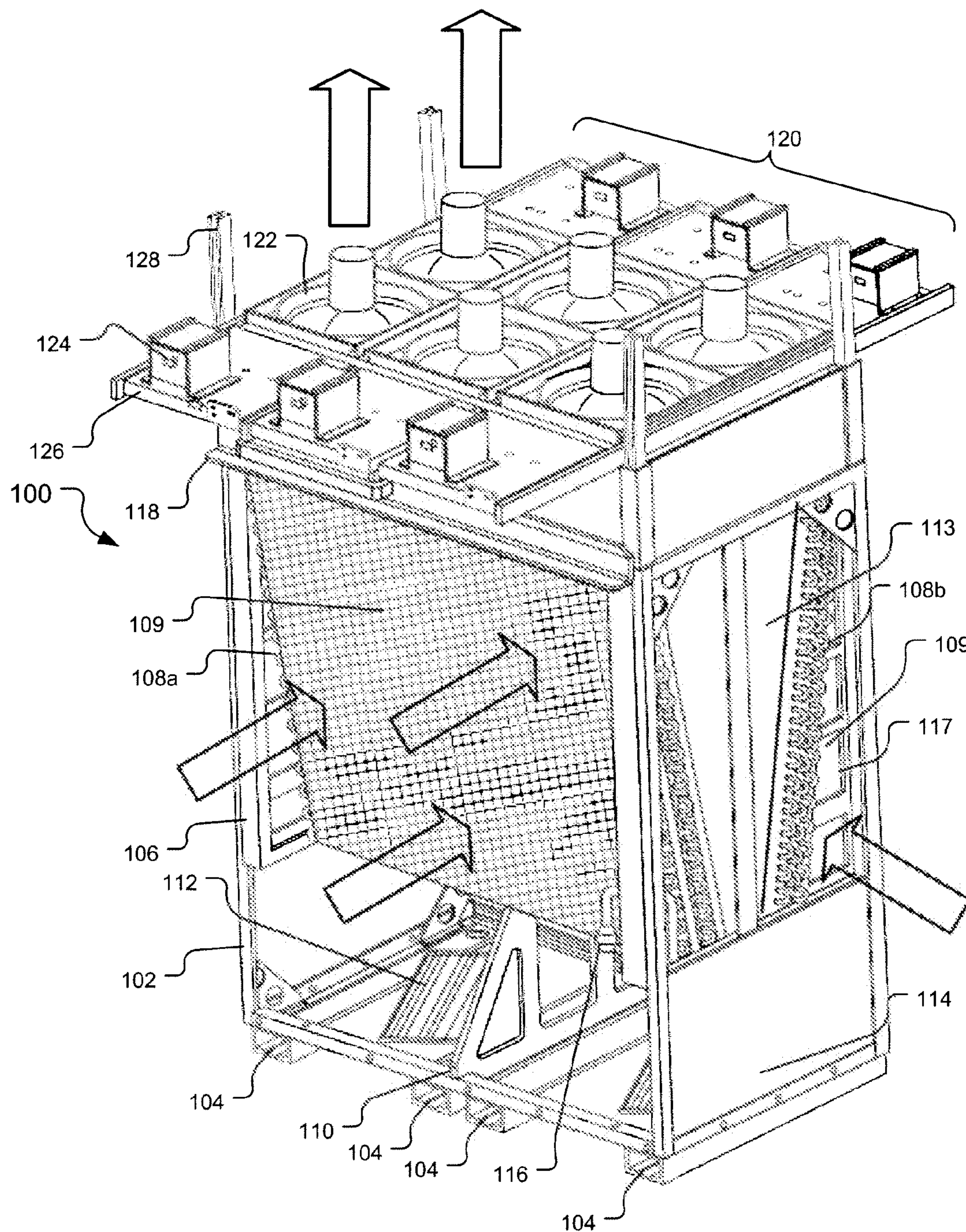
FIG. 1A
