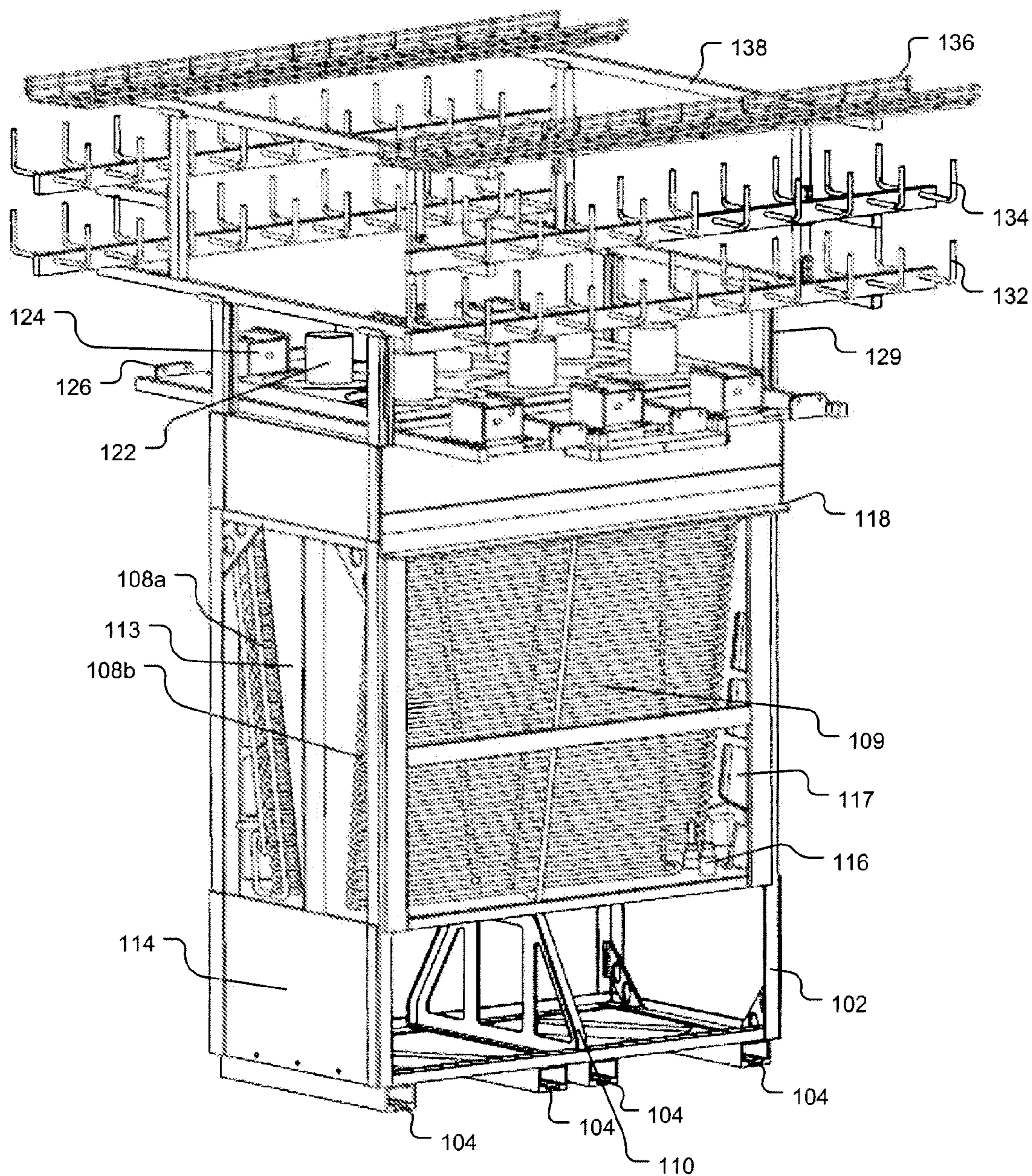
FIG. 1C
