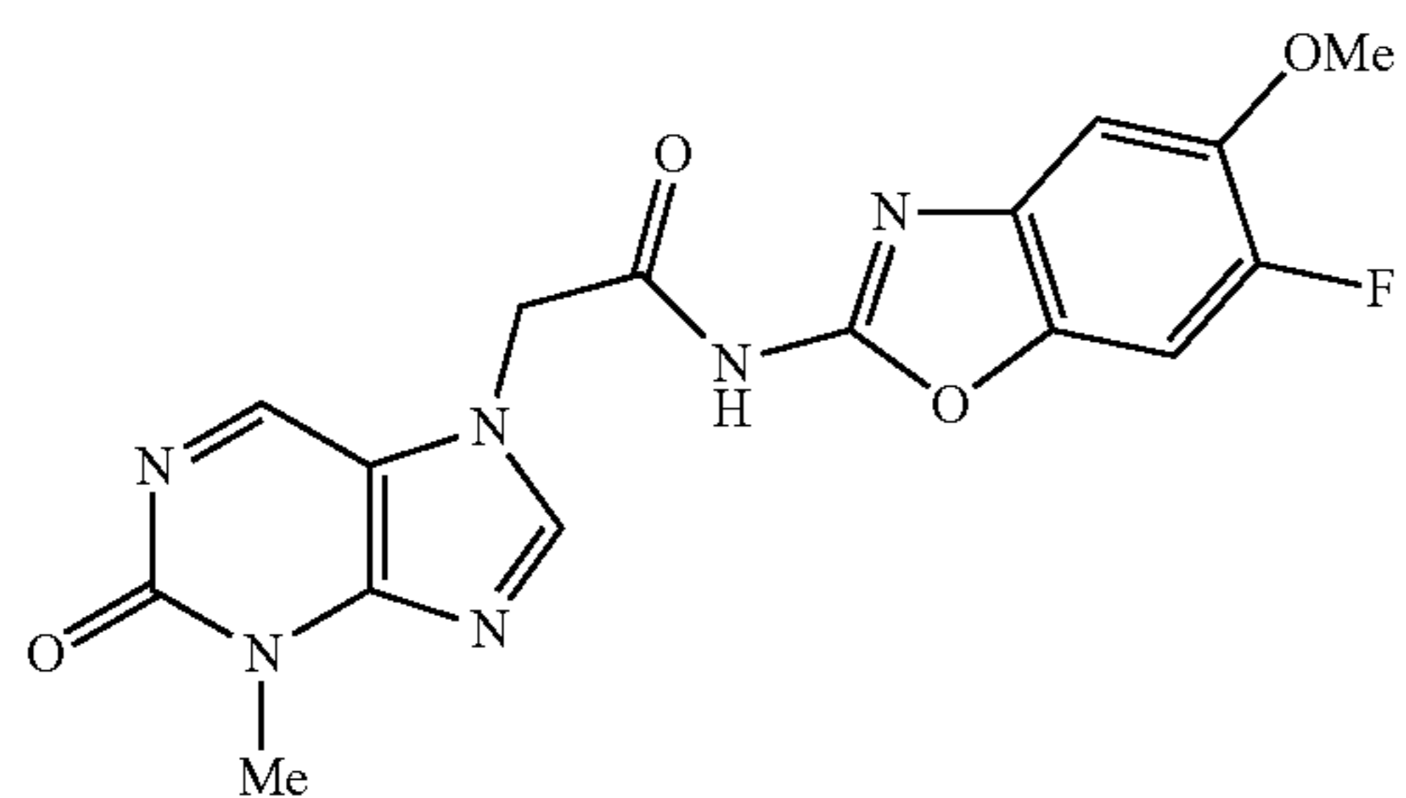
N-(6-fluoro-5-methoxybenzo[d]oxazol-2-yl)-2-(3-methyl-2-oxo-2,3-dihydropurin-7-yl)acetamide
