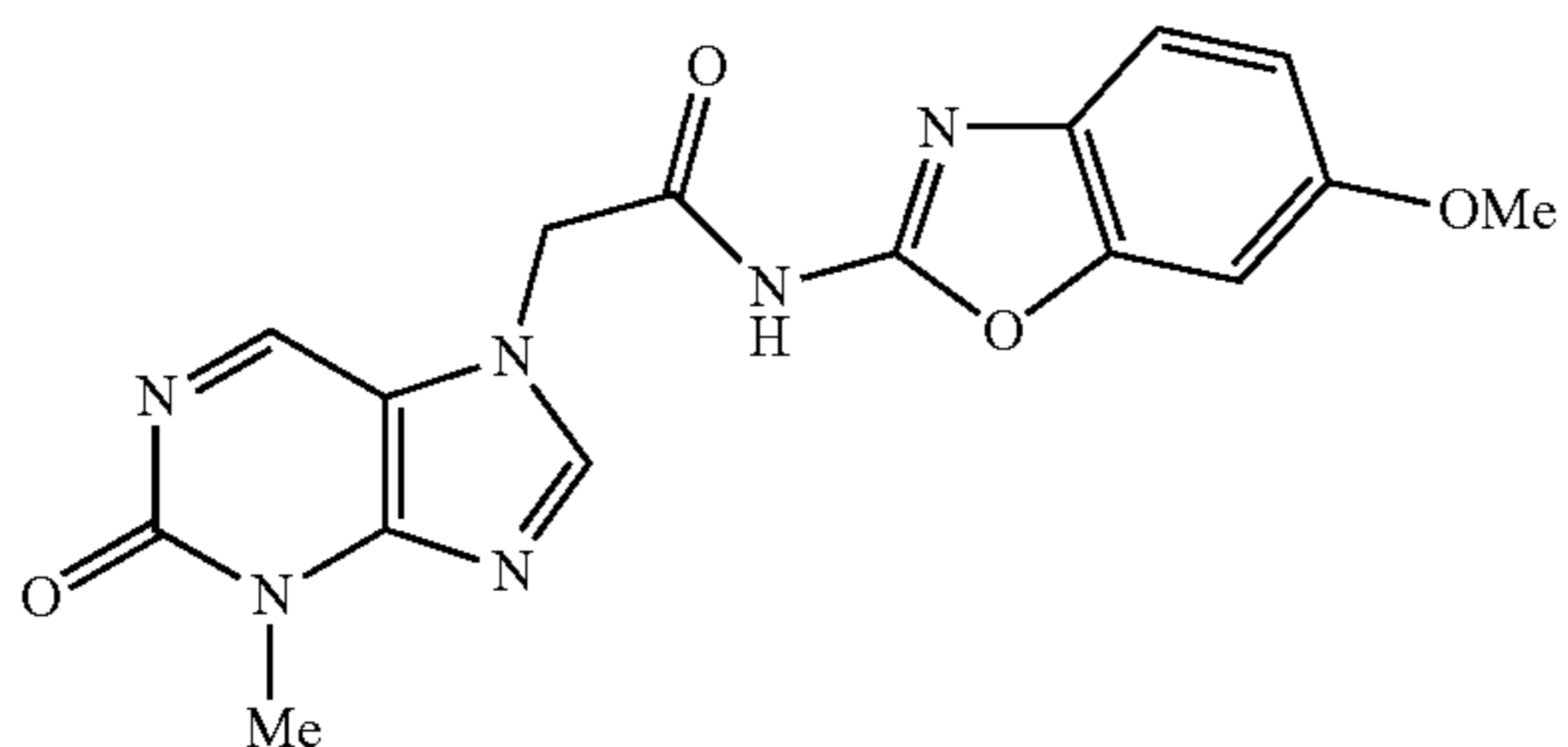
N-(6-methoxybenzo[d]oxazol-2-yl)-2-(3-methyl-2-oxo-2,3-dihydropurin-7-yl)acetamide
