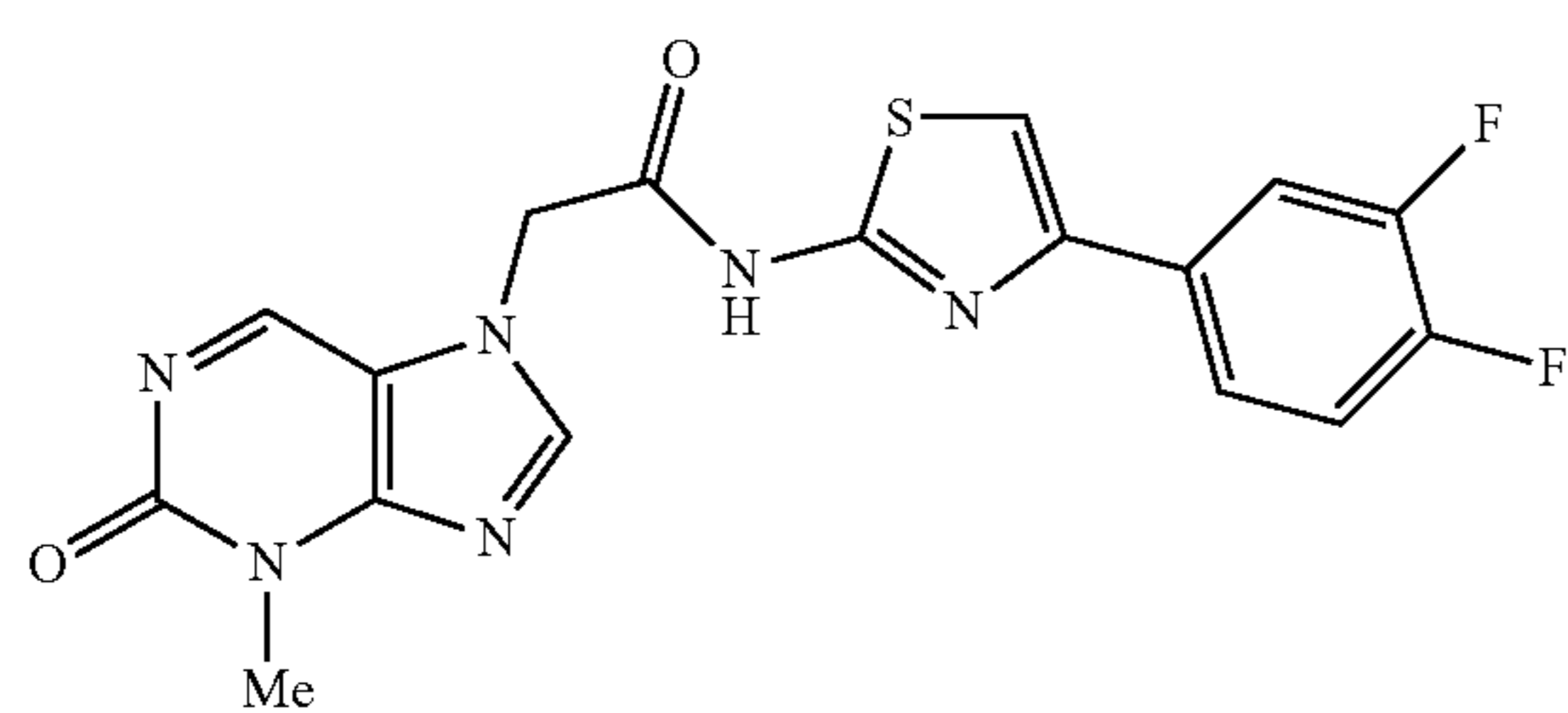
N-(4-(3,4-difluorophenyl)thiazol-2-yl)-2-(3-methyl-2-oxo-2,3-dihydropurin-7-yl)acetamide
