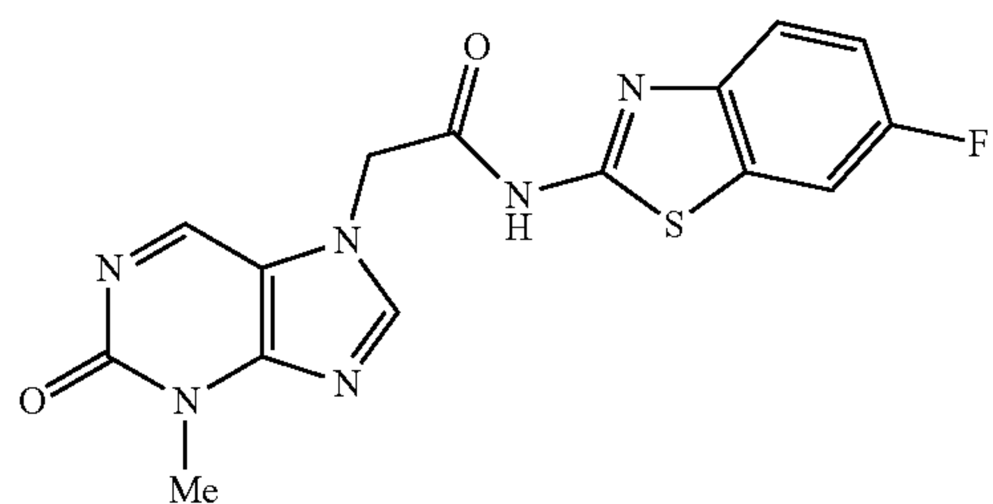
N-(6-fluorobenzo[d]thiazol-2-yl)-2-(3-methyl-2-oxo-2,3-dihydropurin-7-yl)acetamide
