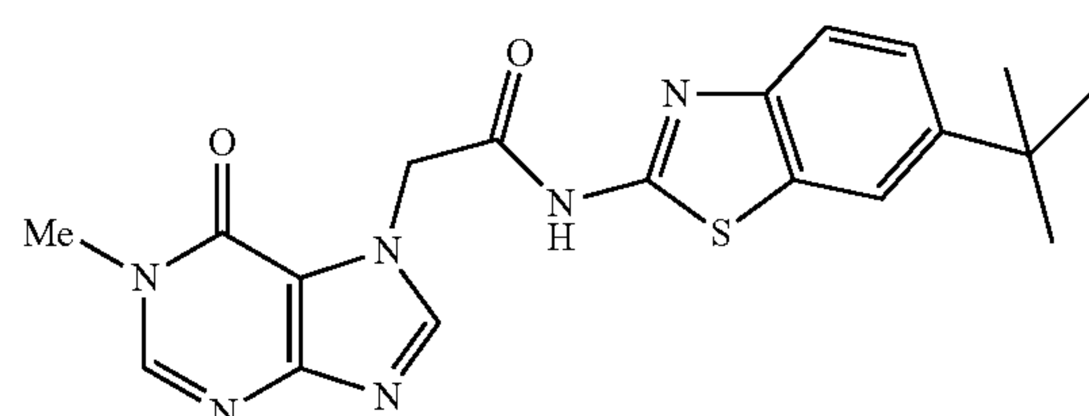
N-(6-tert-butylbenzo[d]thiazol-2-yl)-2-(1-methyl-6-oxo-1H-purin-7(6H)-yl)acetamide
