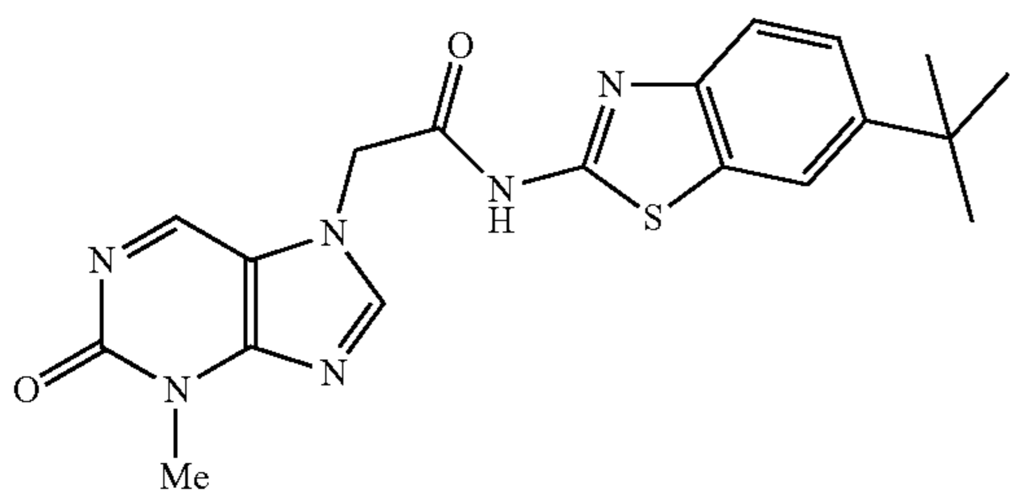
N-(6-tert-butylbenzo[d]thiazol-2-yl)-2-(3-methyl-2-oxo-2,3-dihydropurin-7-yl)acetamide
