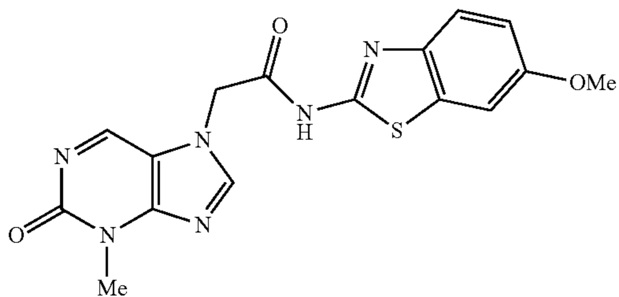
N-(6-methoxybenzo[d]thiazol-2-yl)-2-(3-methyl-2-oxo-2,3-dihydropurin-7-yl)acetamide
