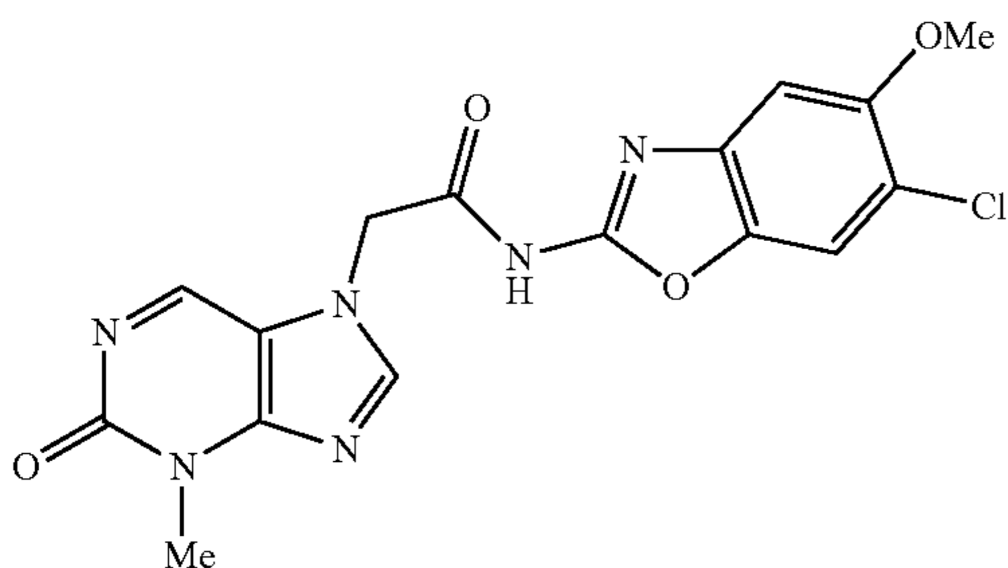
N-(6-chloro-5-methoxybenzo[d]oxazol-2-yl)-2-(3-methyl-2-oxo-2,3-dihydropurin-7-yl)acetamide
