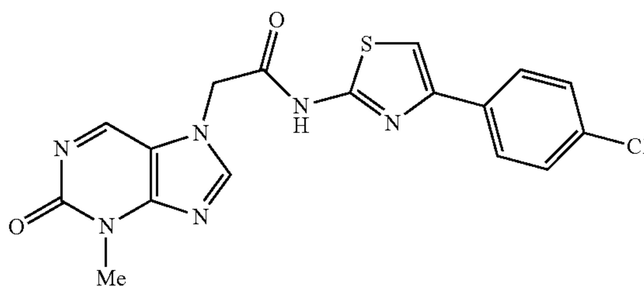
N-(4-(4-chlorophenyl)thiazol-2-yl)-2-(3-methyl-2-oxo-2,3-dihydropurin-7-yl)acetamide
