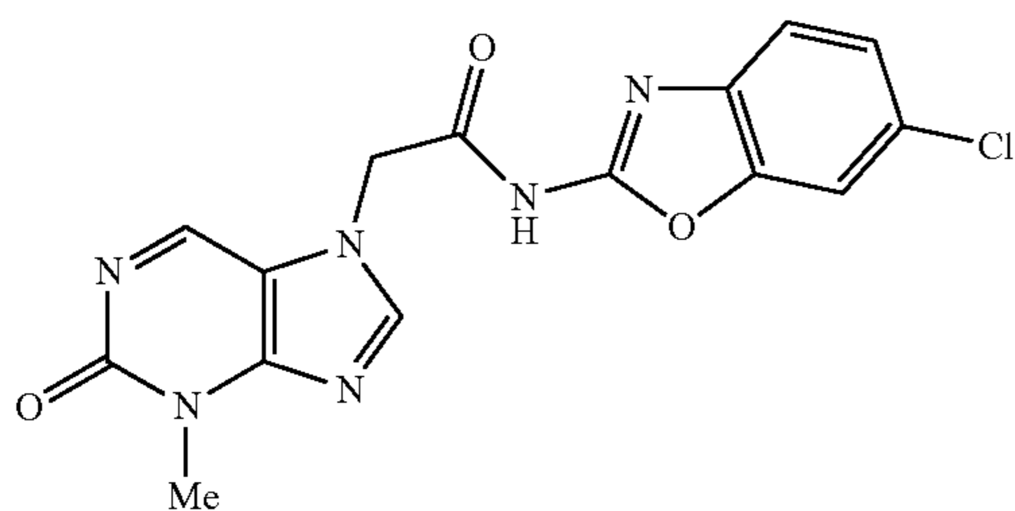
N-(6-chlorobenzo[d]oxazol-2-yl)-2-(3-methyl-2-oxo-2,3-dihydropurin-7-yl)acetamide
