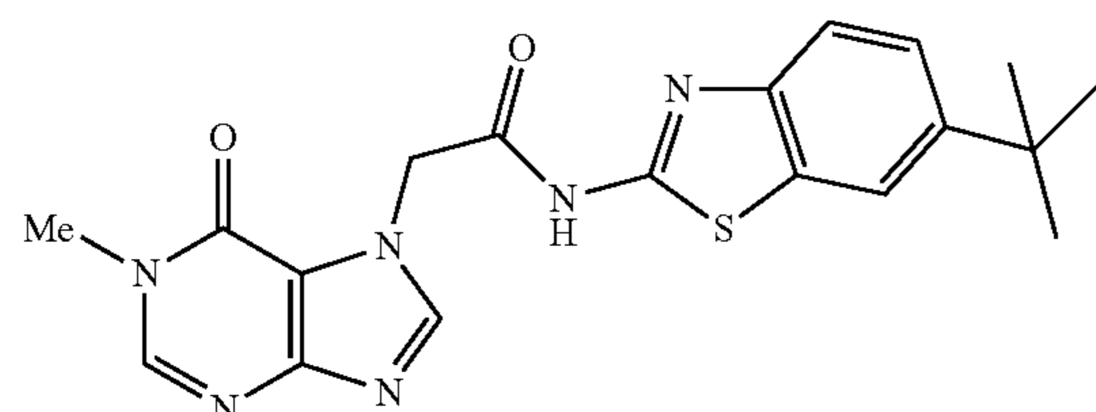
N-(6-tert-butylbenzo[d]thiazol-2-yl)-2-(1-methyl-6-oxo-1H-purin-7(6H)-yl)acetamide
