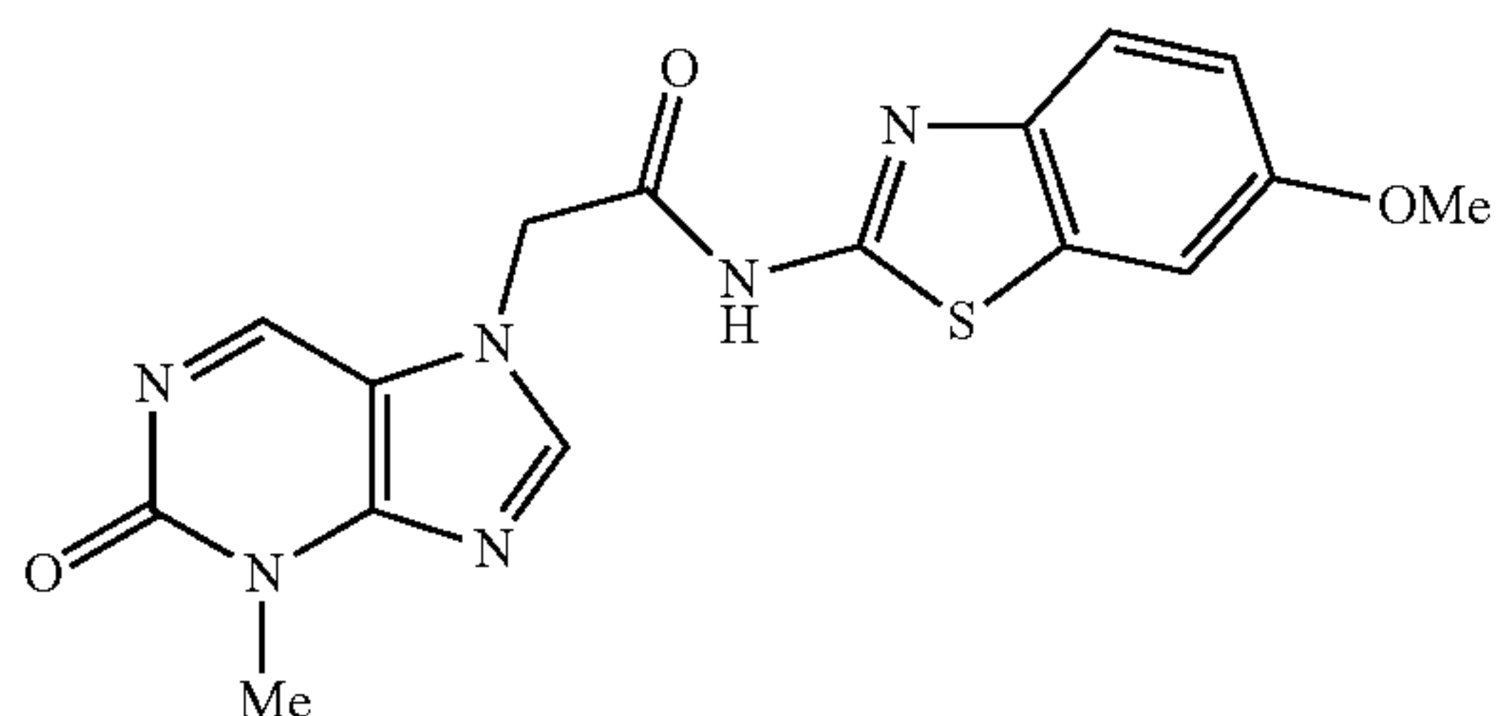
N-(6-methoxybenzo[d]thiazol-2-yl)-2-(3-methyl-2-oxo-2,3-dihydropurin-7-yl)acetamide
