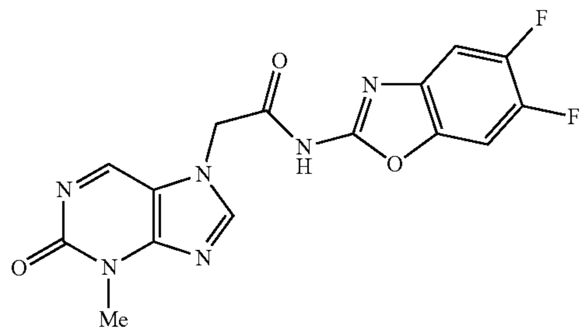
N-(5,6-difluorobenzo[d]oxazol-2-yl)-2-(3-methyl-2-oxo-2,3-dihydropurin-7-yl)acetamide
