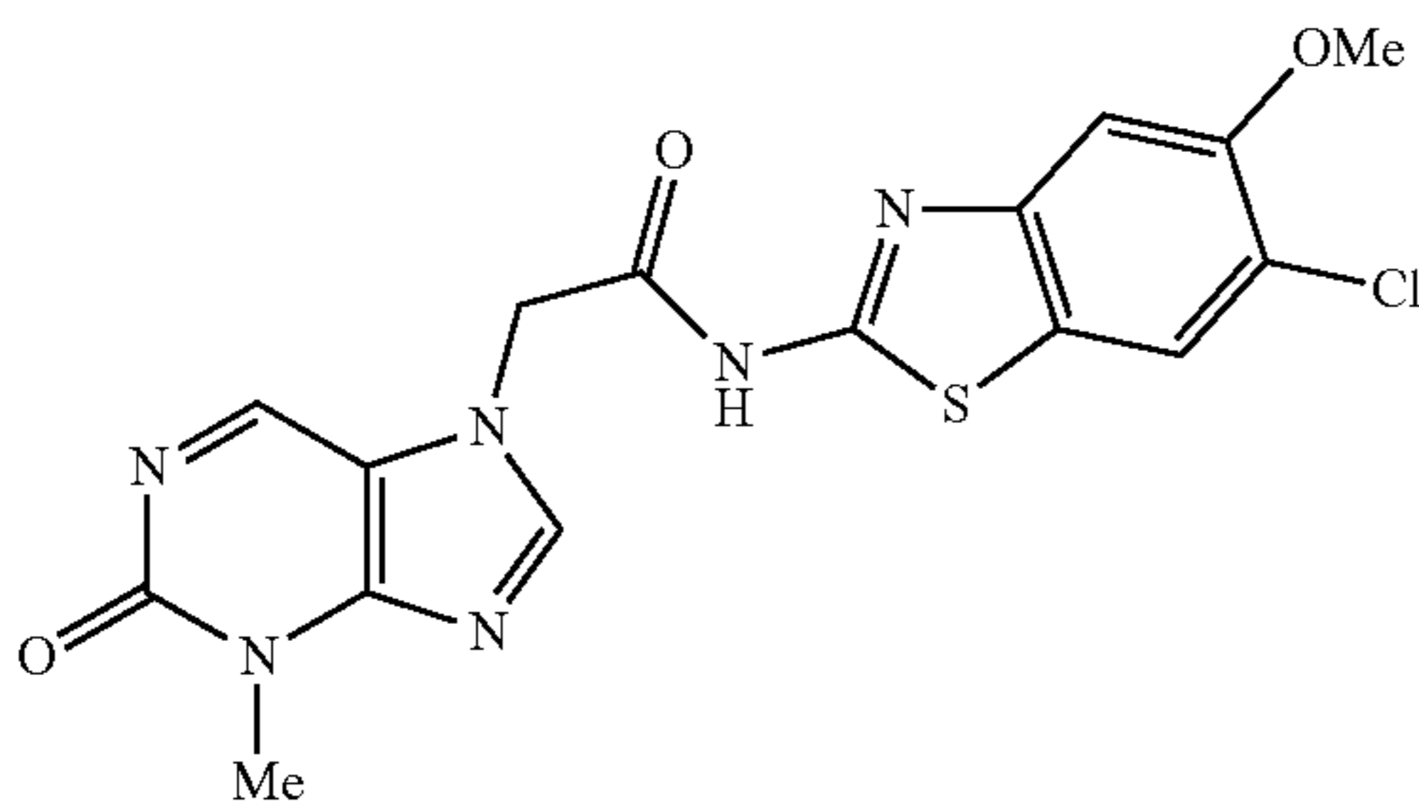
N-(6-chloro-5-methoxybenzo[d]thiazol-2-yl)-2-(3-methyl-2-oxo-2,3-dihydropurin-7-yl)acetamide
