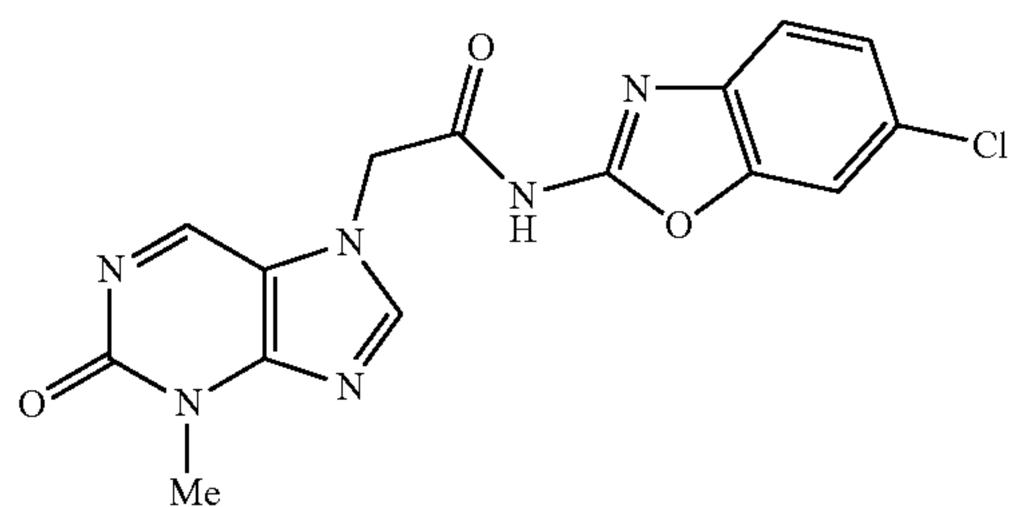
N-(6-chlorobenzo[d]oxazol-2-yl)-2-(3-methyl-2-oxo-2,3-dihydropurin-7-yl)acetamide
