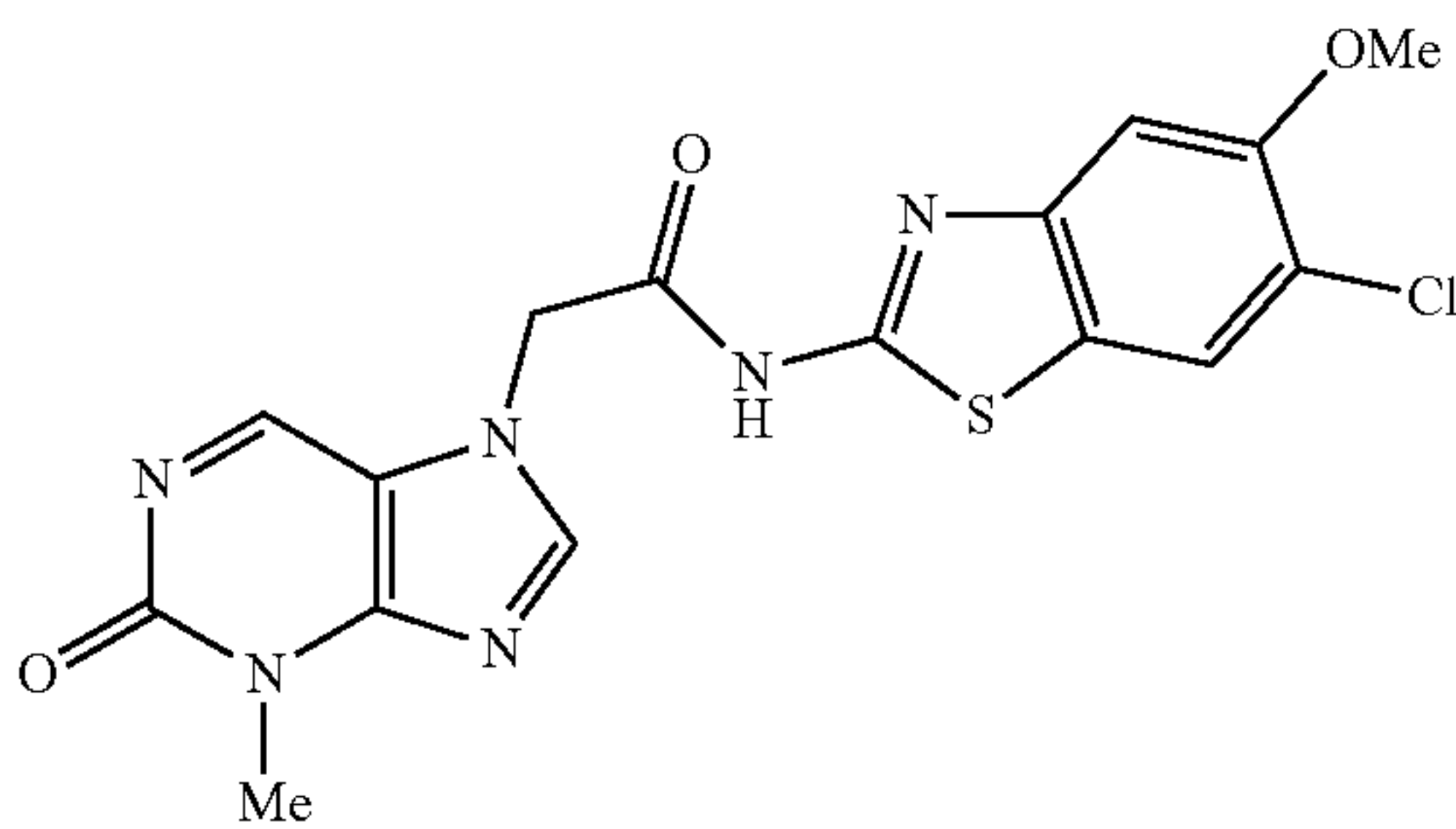
N-(6-chloro-5-methoxybenzo[d]thiazol-2-yl)-2-(3-methyl-2-oxo-2,3-dihydropurin-7-yl)acetamide
