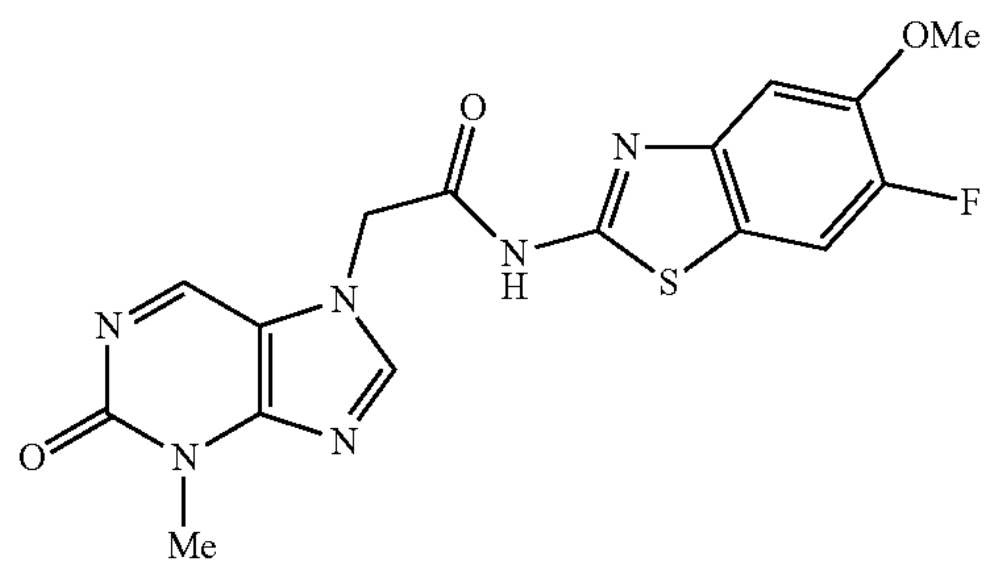
N-(6-fluoro-5-methoxybenzo[d]thiazol-2-yl)-2-(3-methyl-2-oxo-2,3-dihydropurin-7-yl)acetamide
