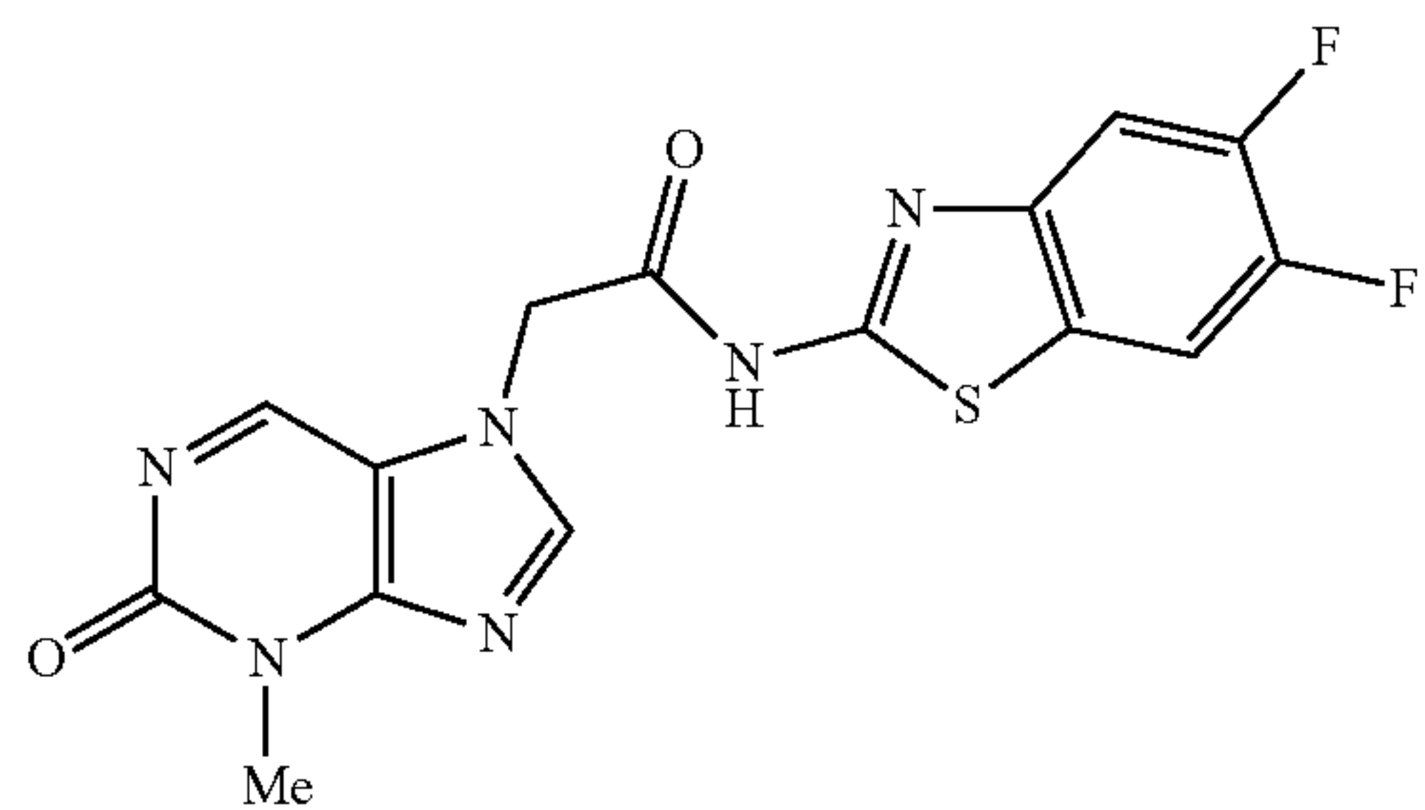
N-(5,6-difluorobenzo[d]thiazol-2-yl)-2-(3-methyl-2-oxo-2,3-dihydropurin-7-yl)acetamide
