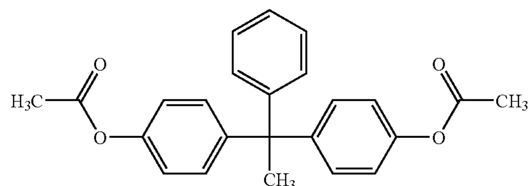
1,1-Bis-(4-acetoxyphenyl)-1-phenyl-ethane (I-10)
