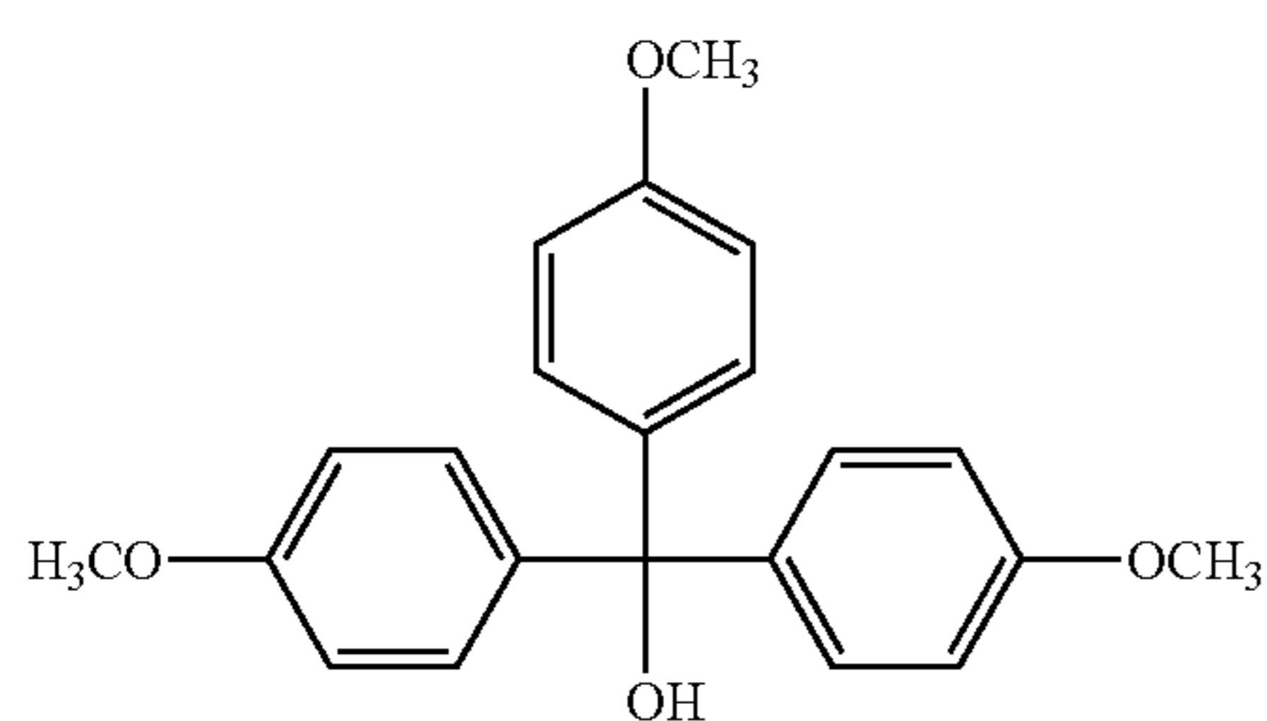
1,1,1-Tris-(4-methoxyphenyl)methanol (I-6)
