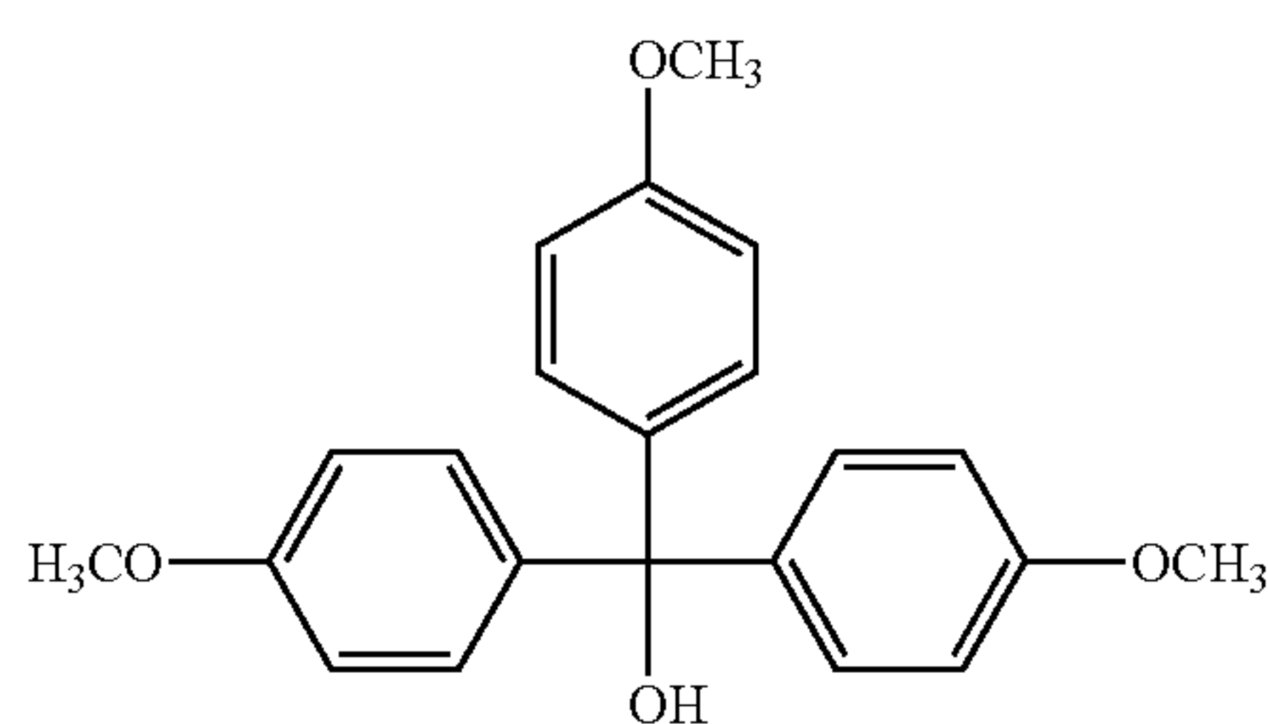
1,1,1-Tris-(4-methoxyphenyl)methanol (I-6)
