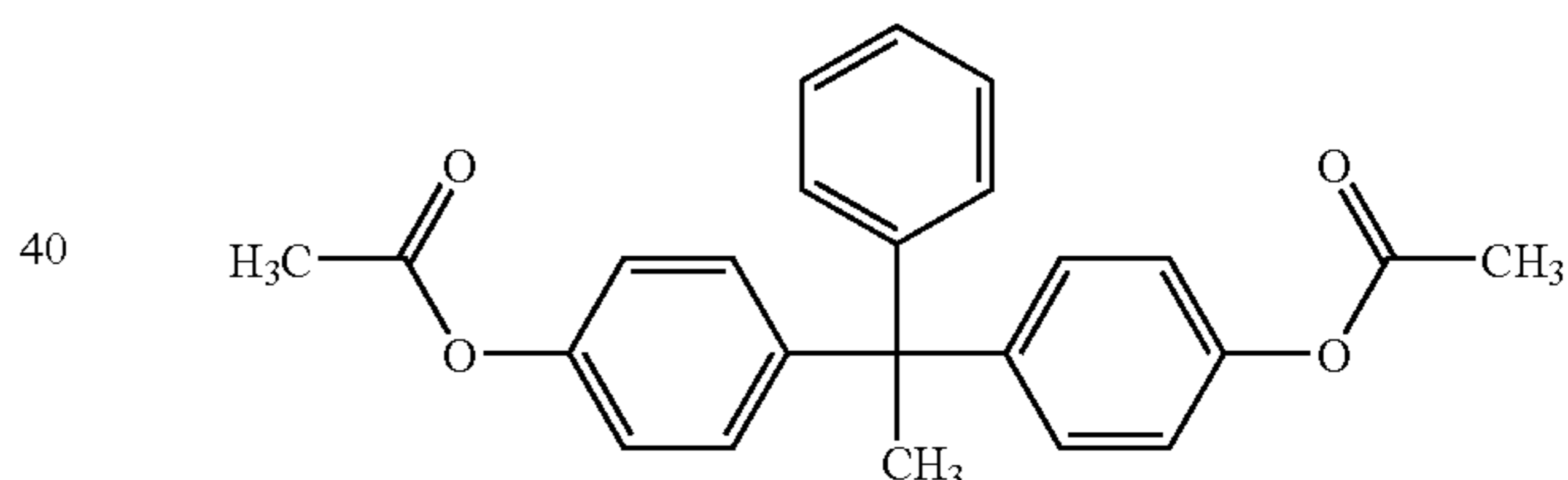
1,1-Bis-(4-acetoxyphenyl)-1-phenyl-ethane (I-10)
