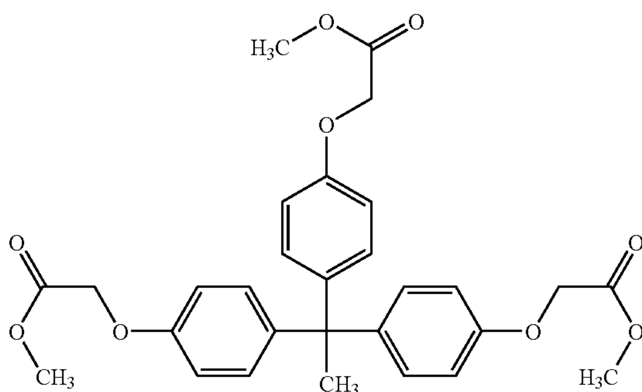
1,1,1-Tris-(4-methoxycarbonylmethoxyphenyl)ethane (I-4)
