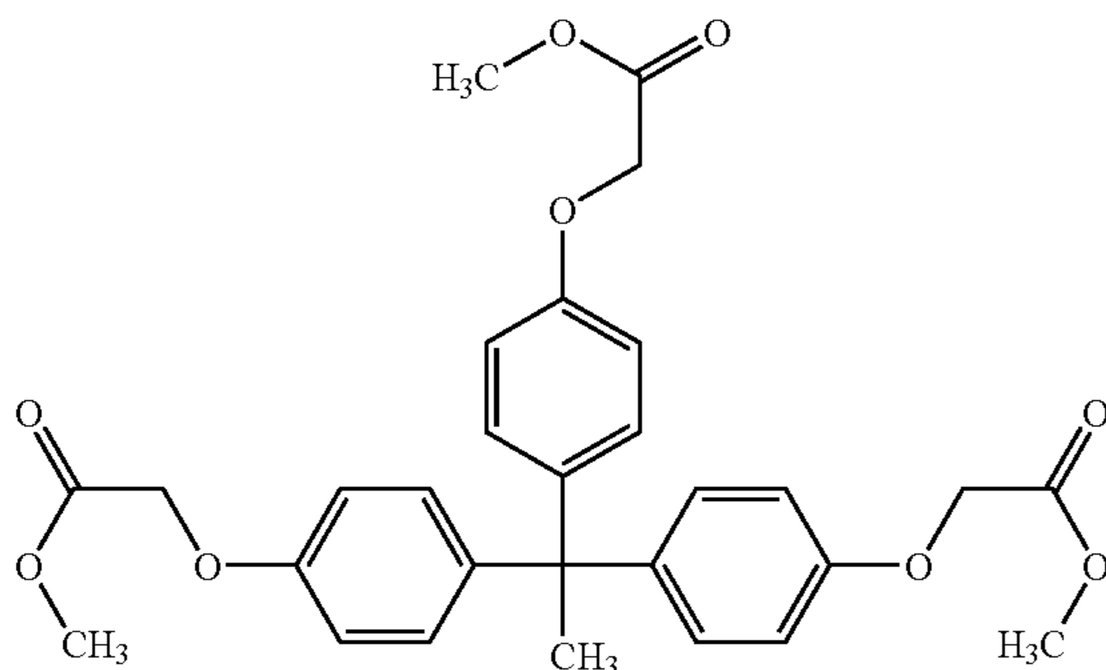
1,1,1-Tris-(4-methoxycarbonylmethoxyphenyl)ethane (I-4)
