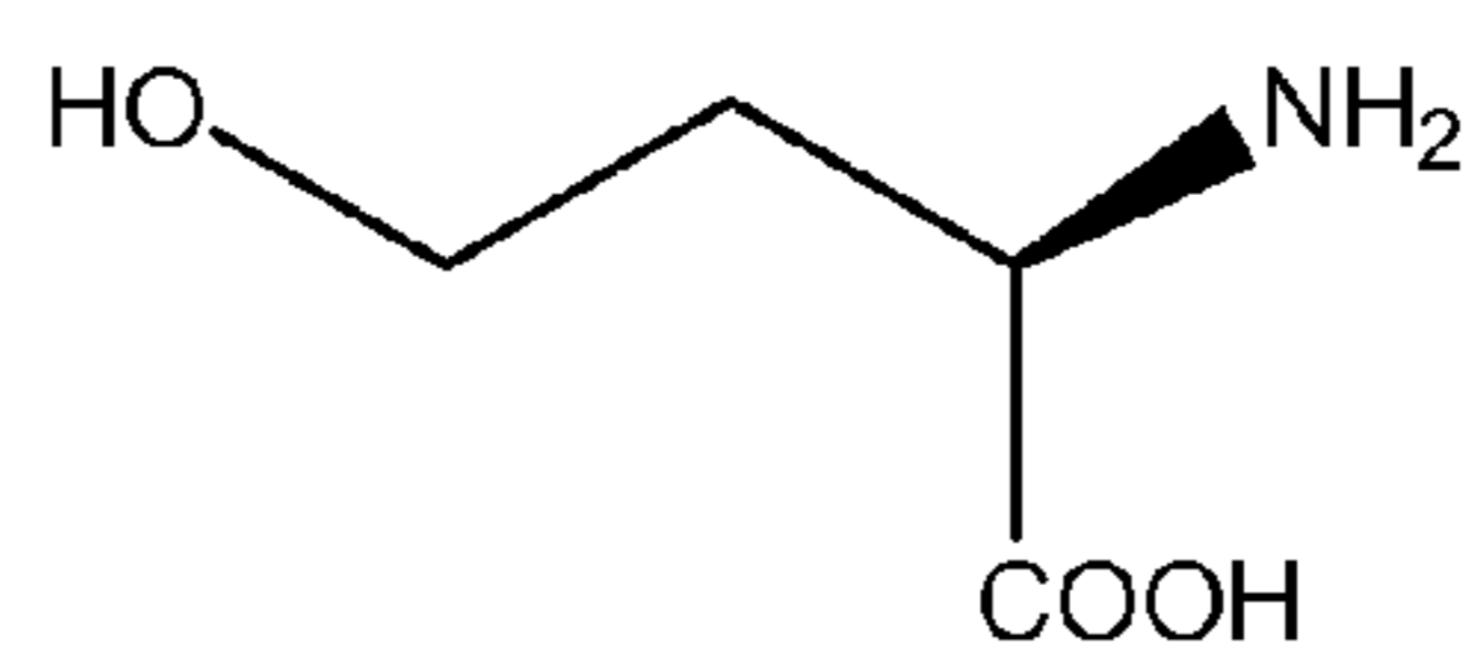
D-homoserine
