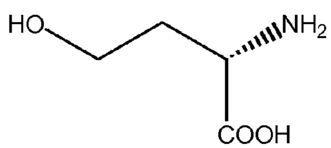
L-homoserine
