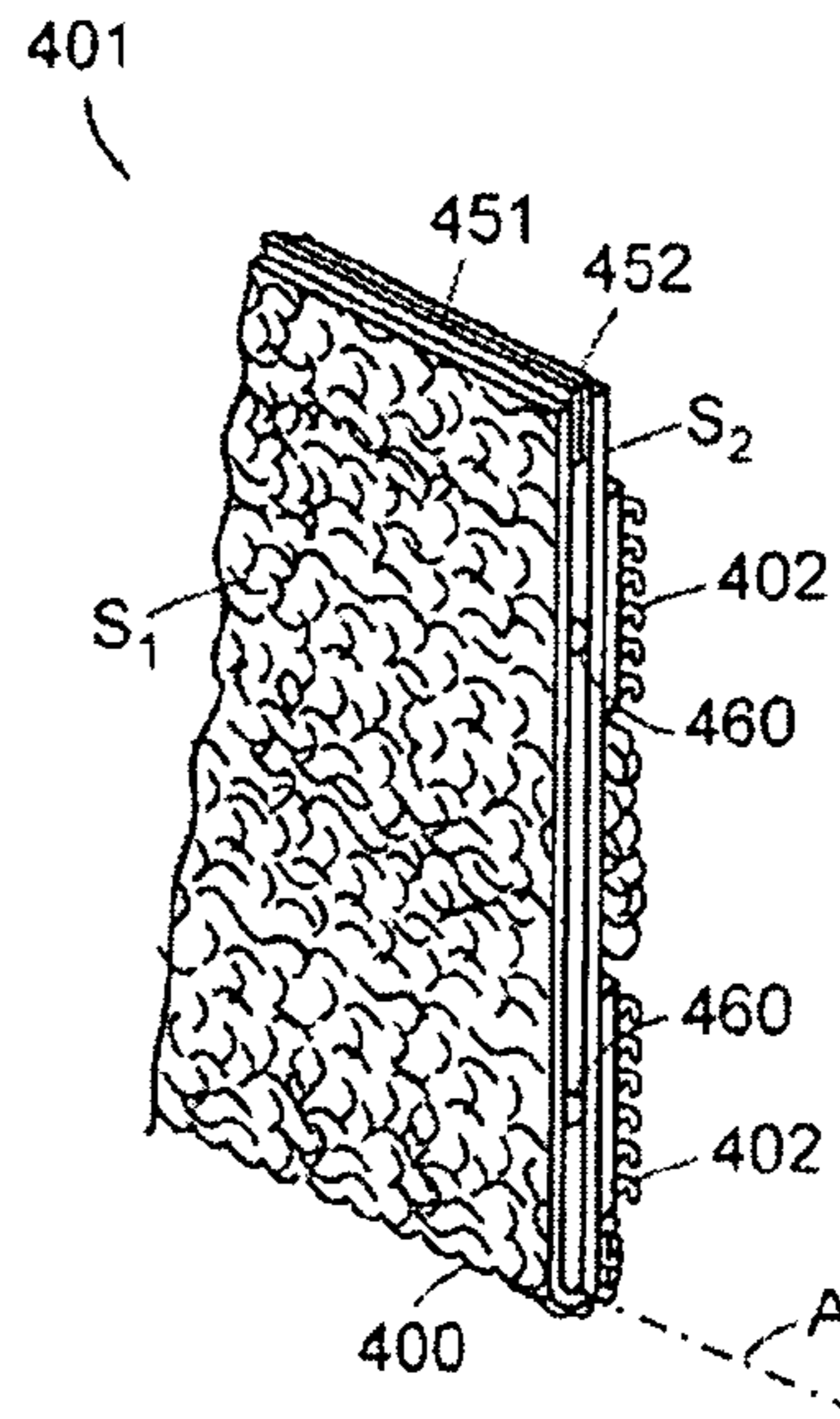
FIG. 15A
