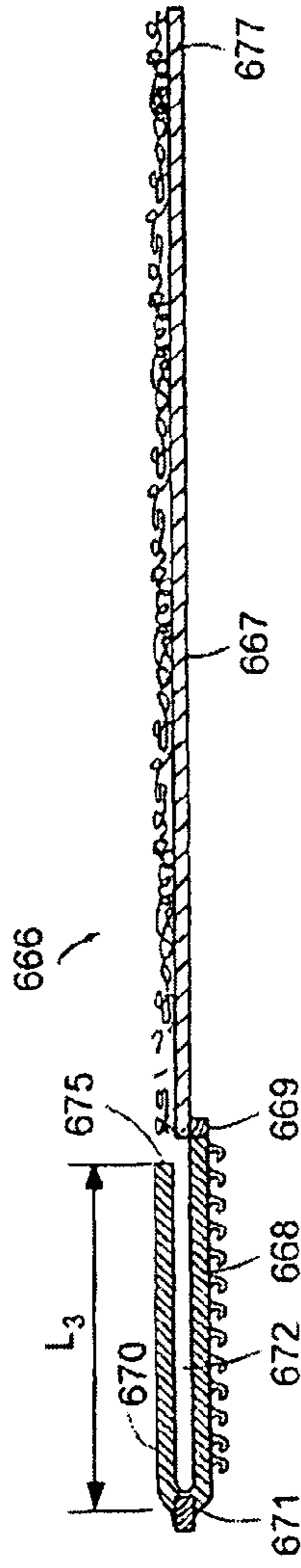
FIG. 20A
