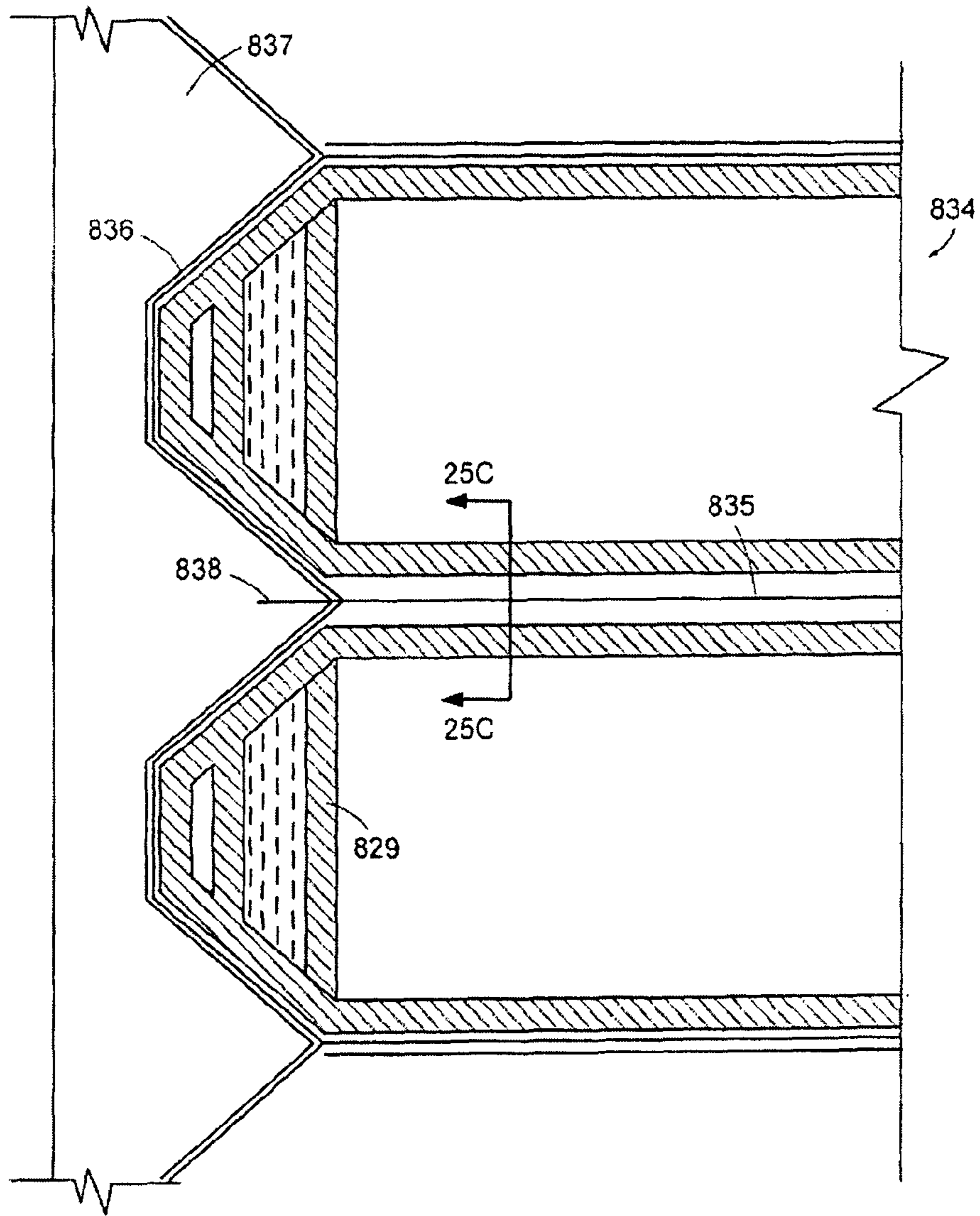
FIG. 25B
