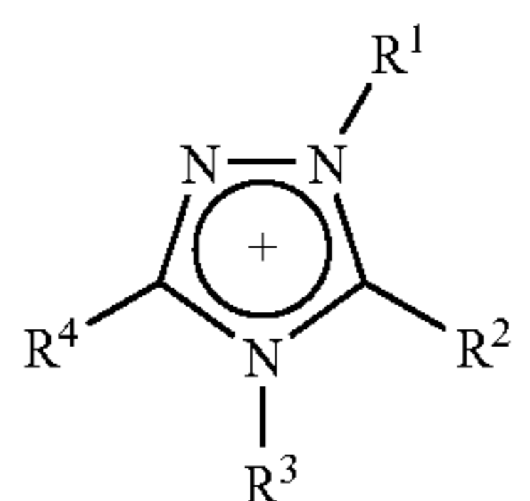
Triazolium
