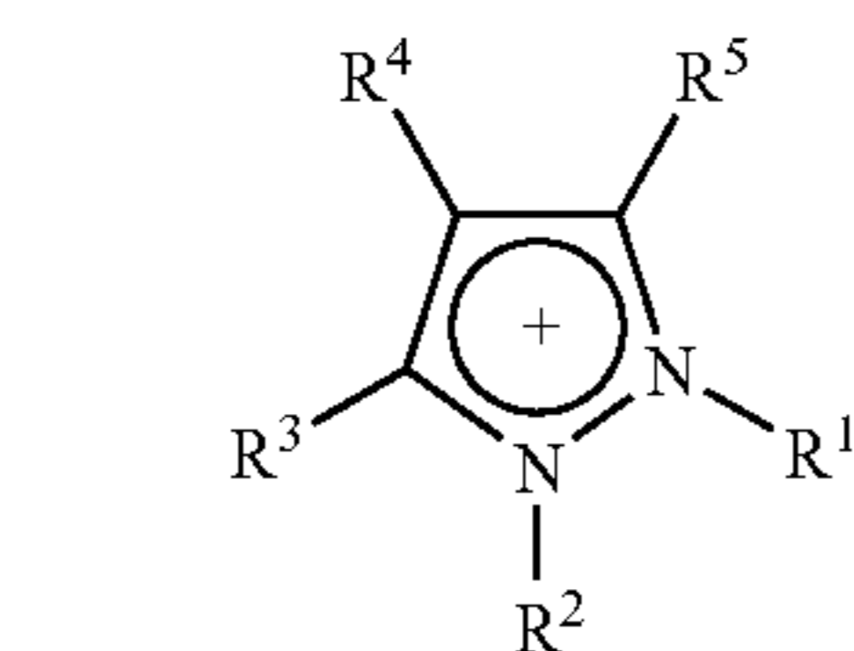
Imidazolium
