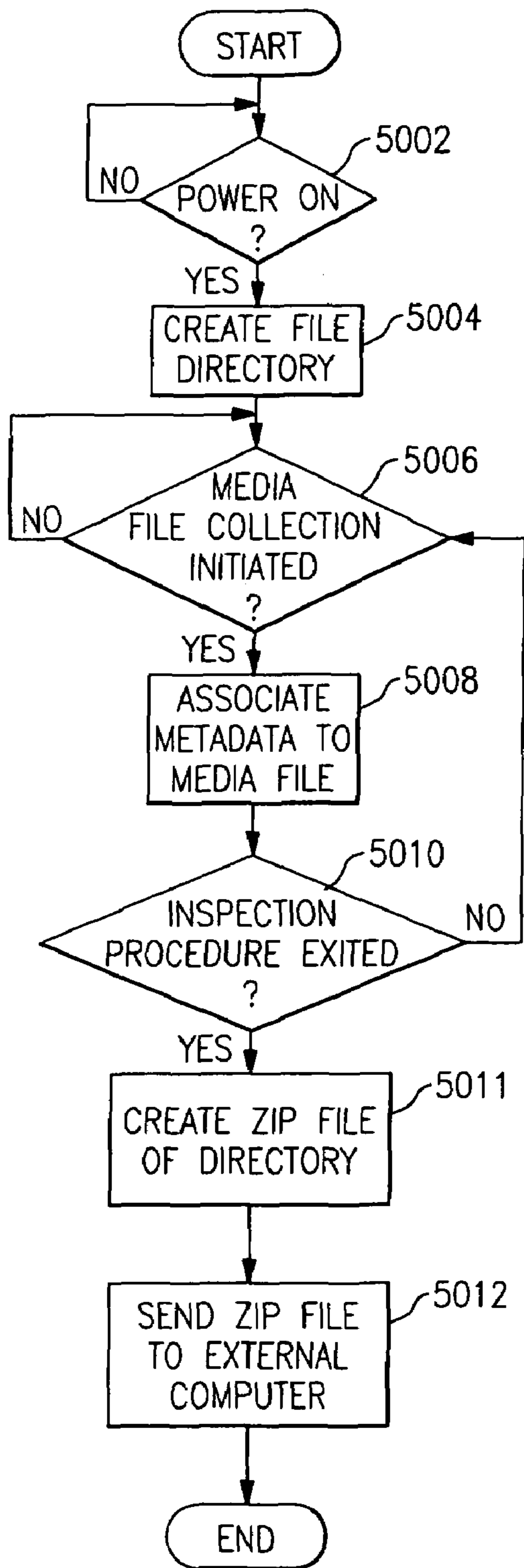
FIG. 5A
