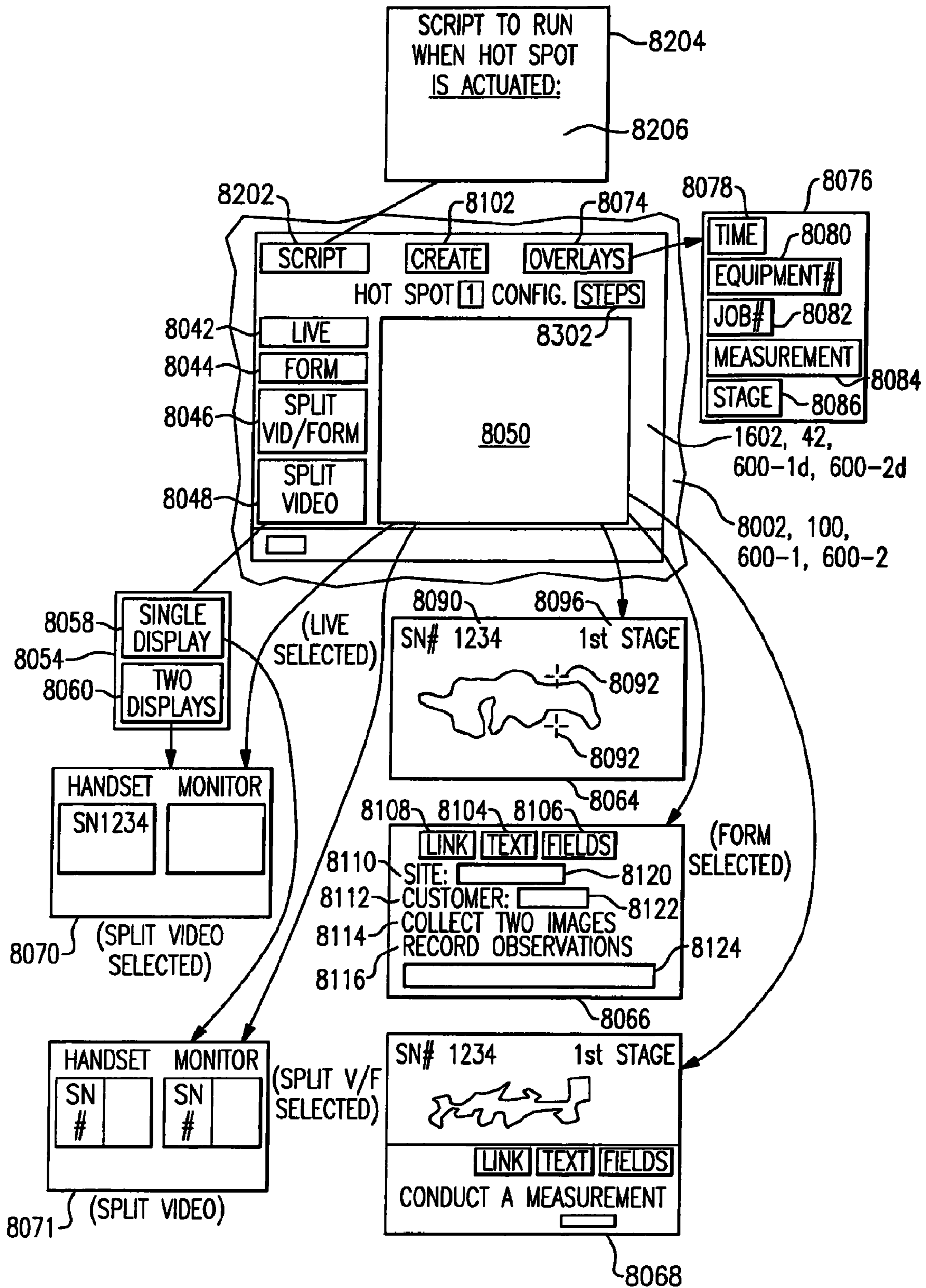
FIG. 10C
