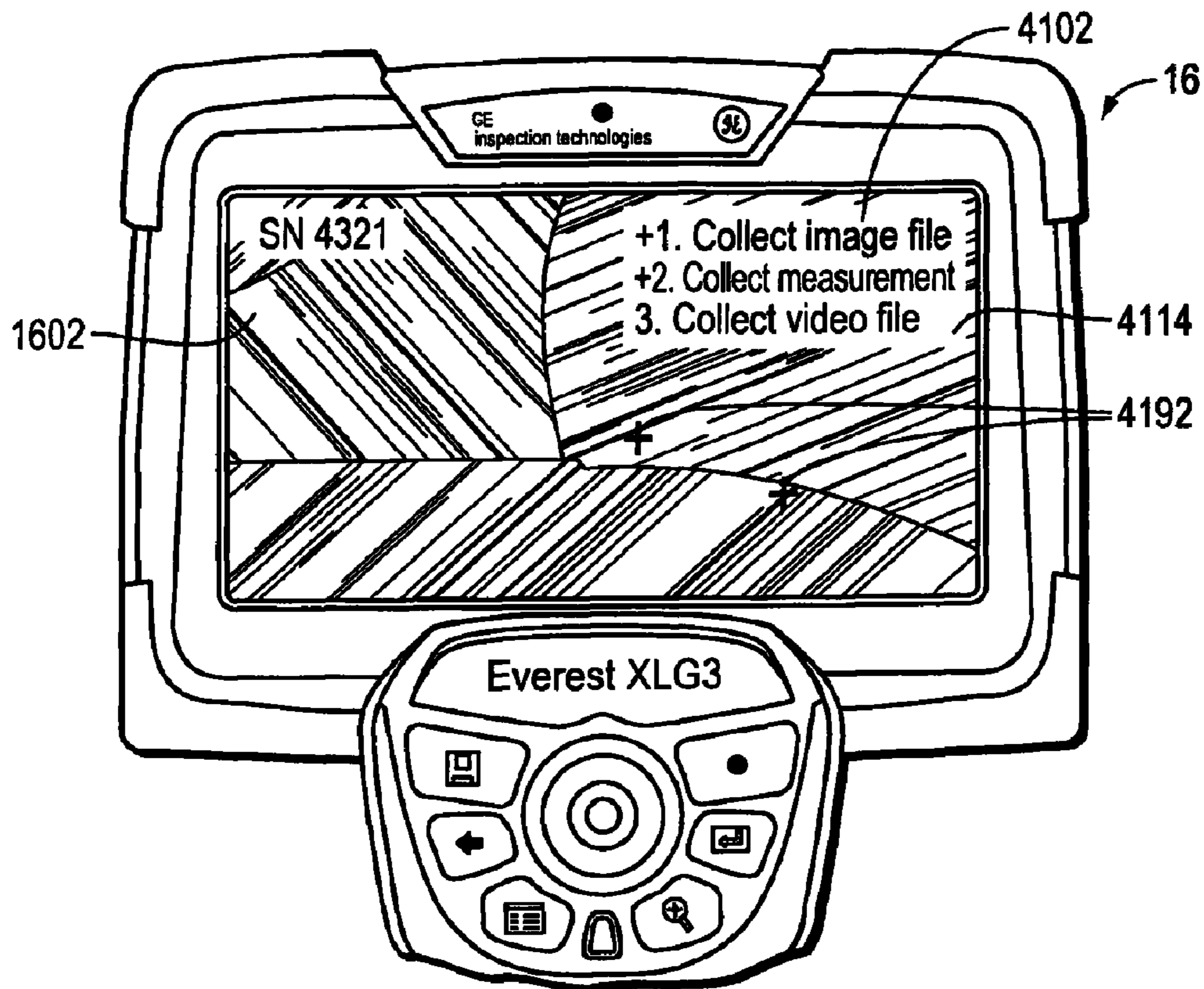
FIG. 4C
