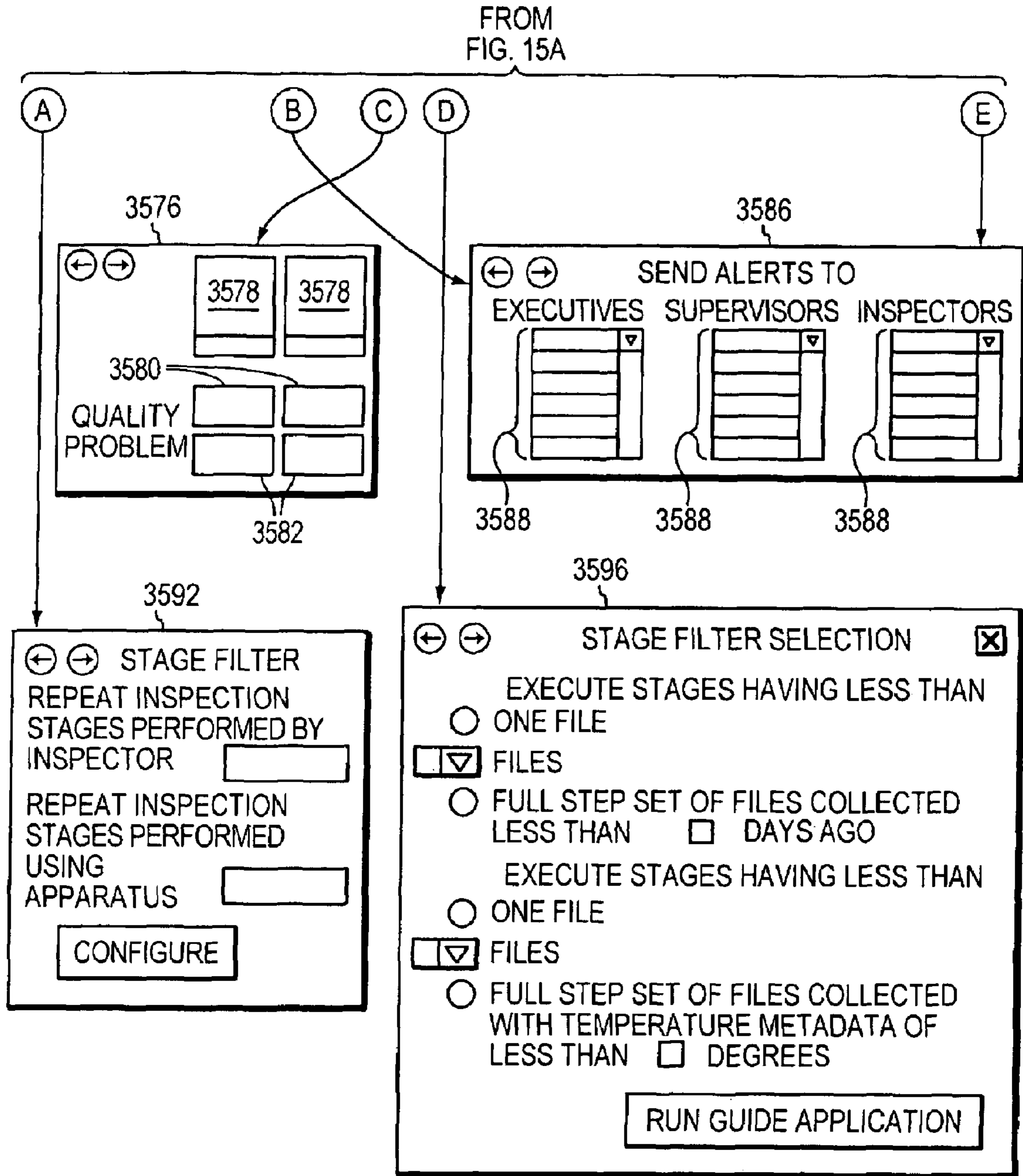
FIG. 15B
