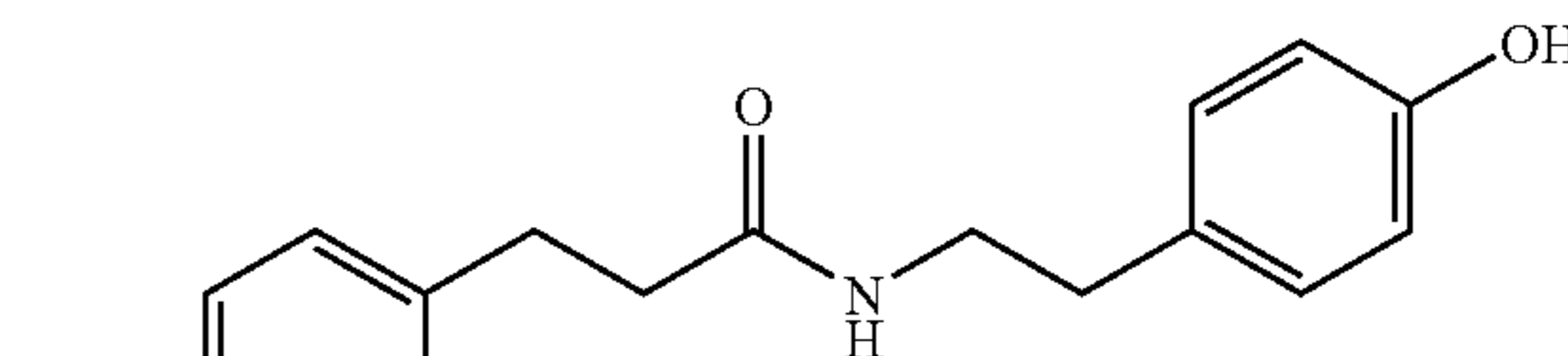
C_{17}H_{19}NO_3 Mol. Wt.: 285.34
