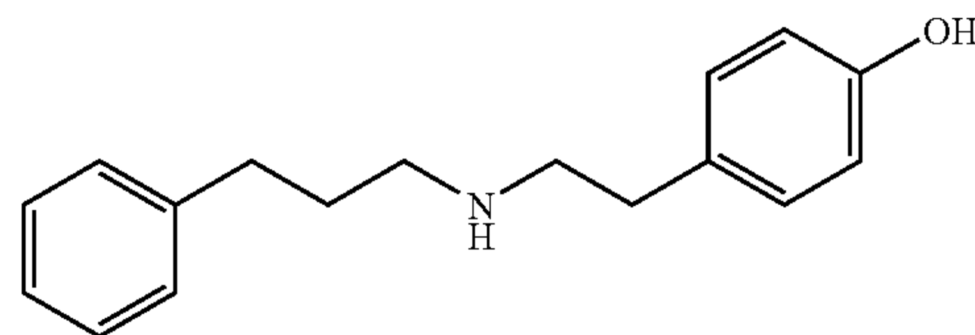
C_{17}H_{21}NO Mol. Wt.: 255.35
