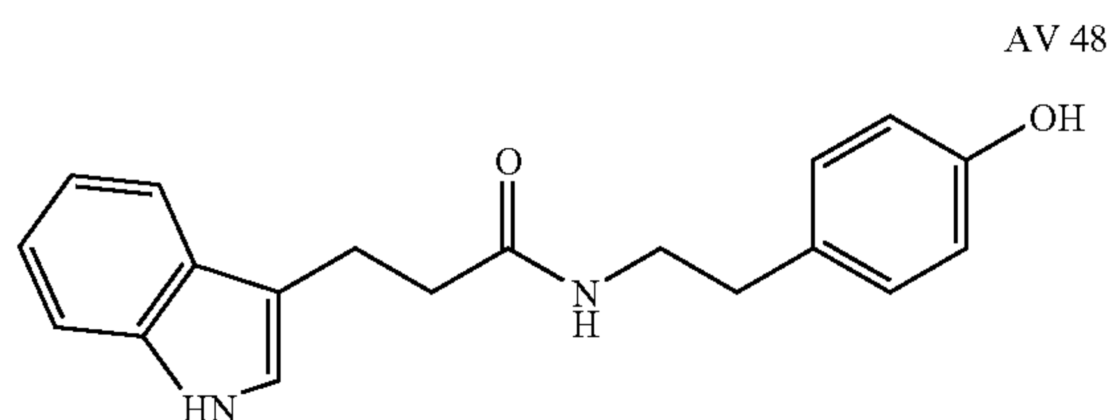
C_{19}H_{20}N_2O_2 Mol. Wt.: 308.37
