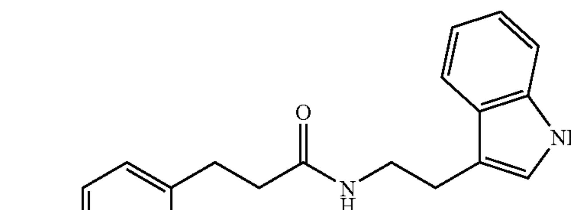
C_{19}H_{20}N_2O_2 Mol. Wt.: 308.37
