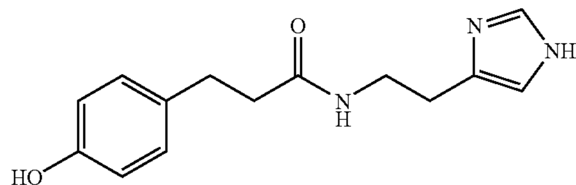
C_{14}H_{17}N_3O_2 Mol. Wt.: 259.30
