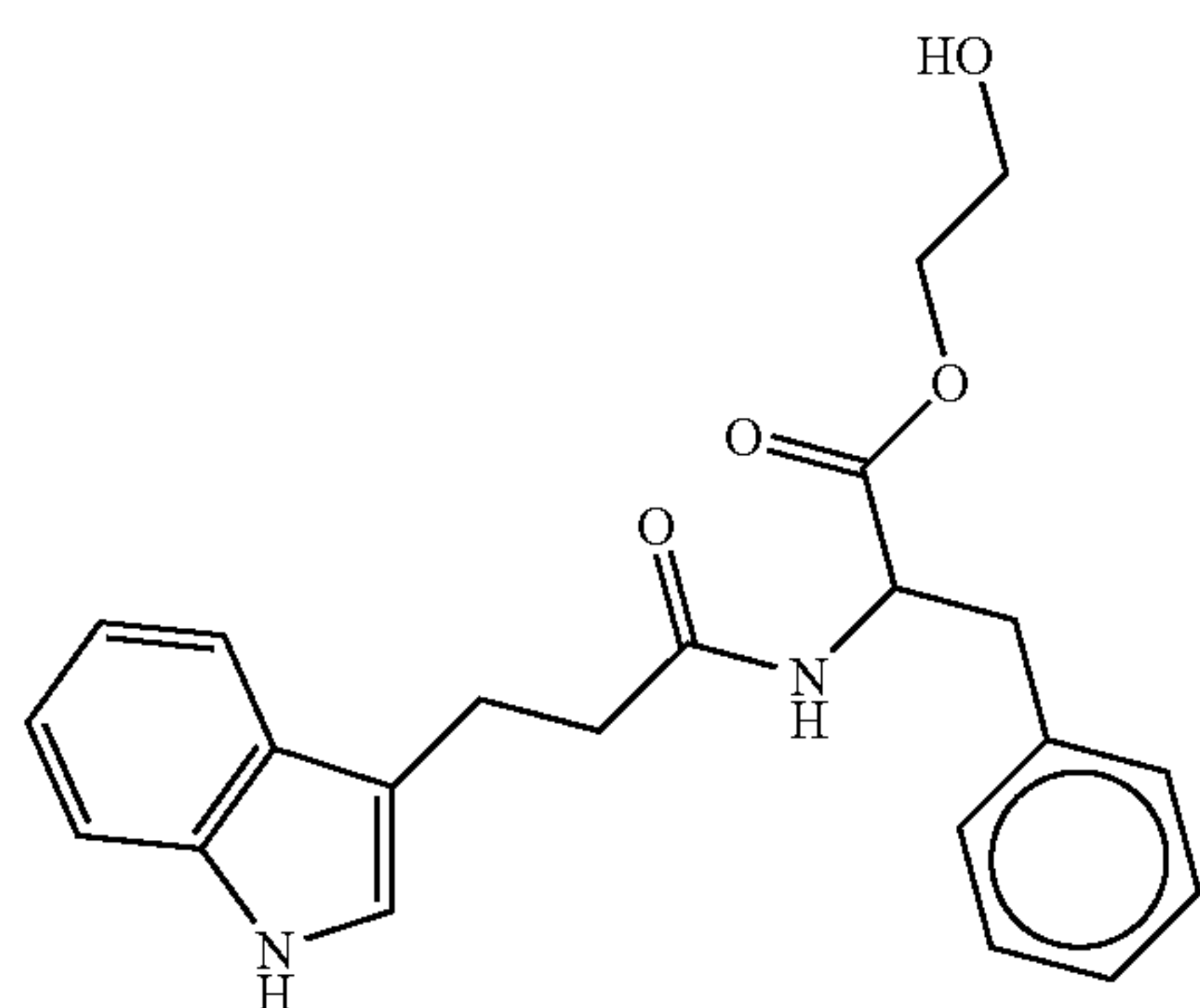
C_{22}H_{24}N_2O_4 Mol. Wt.: 380.44
