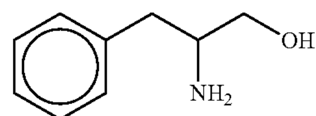
C_9H_{13}NO Mol. Wt.: 151.21
