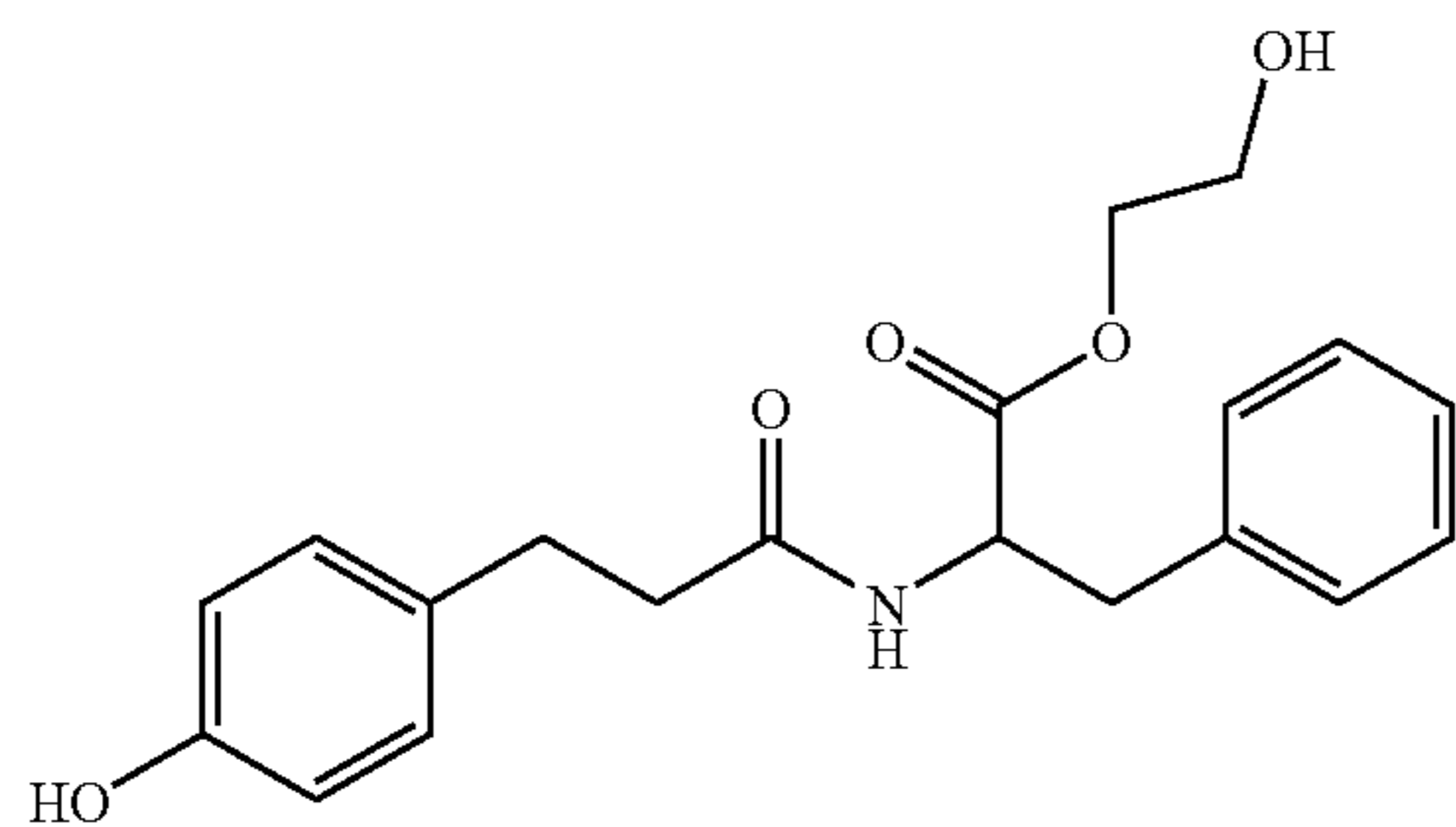
C_{20}H_{23}NO_5 Mol. Wt.: 357.40
