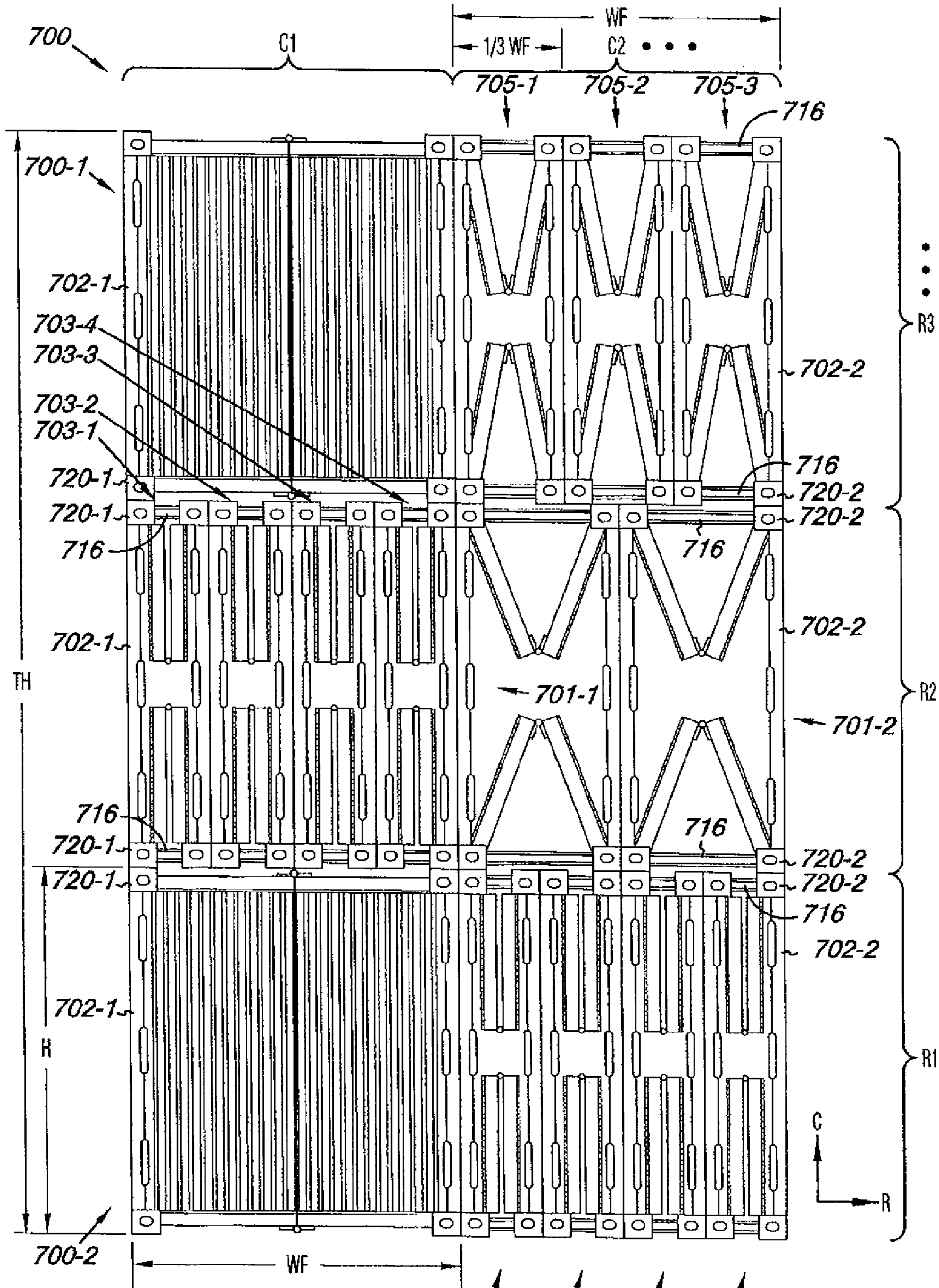
703-1 703-2 703-3 703-4 Fig. 7
