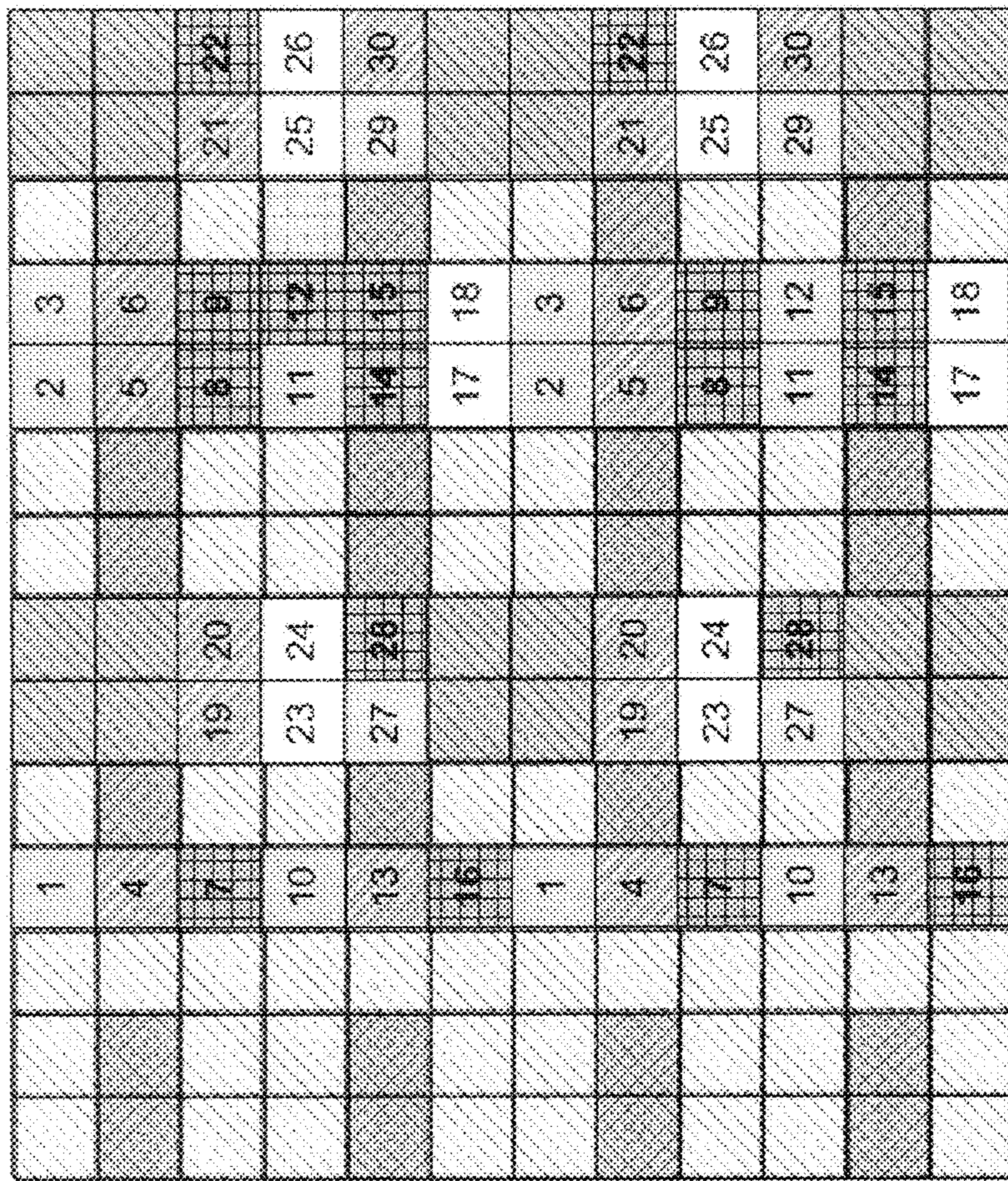
Subframe Y
