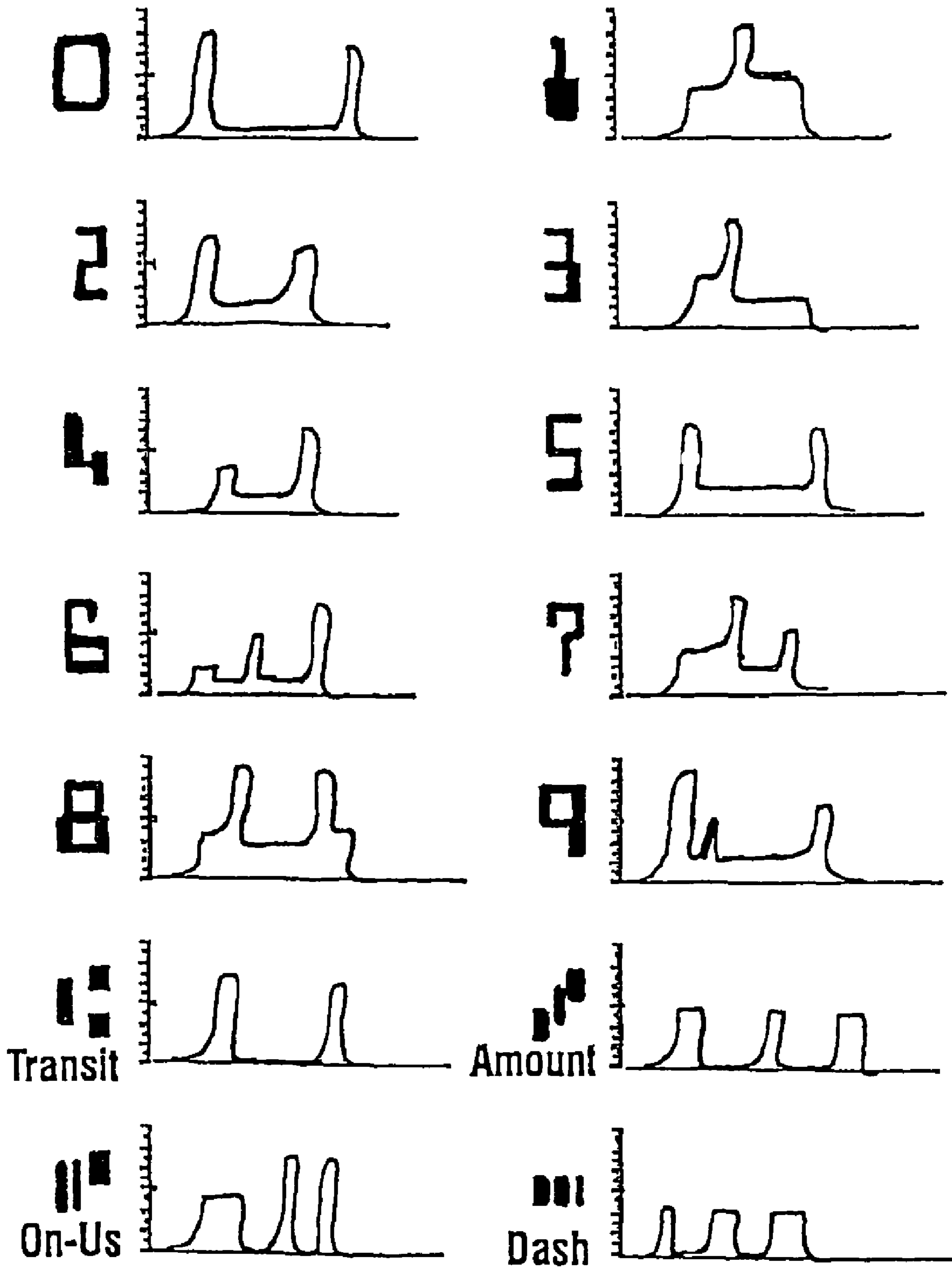
FIG. 49
