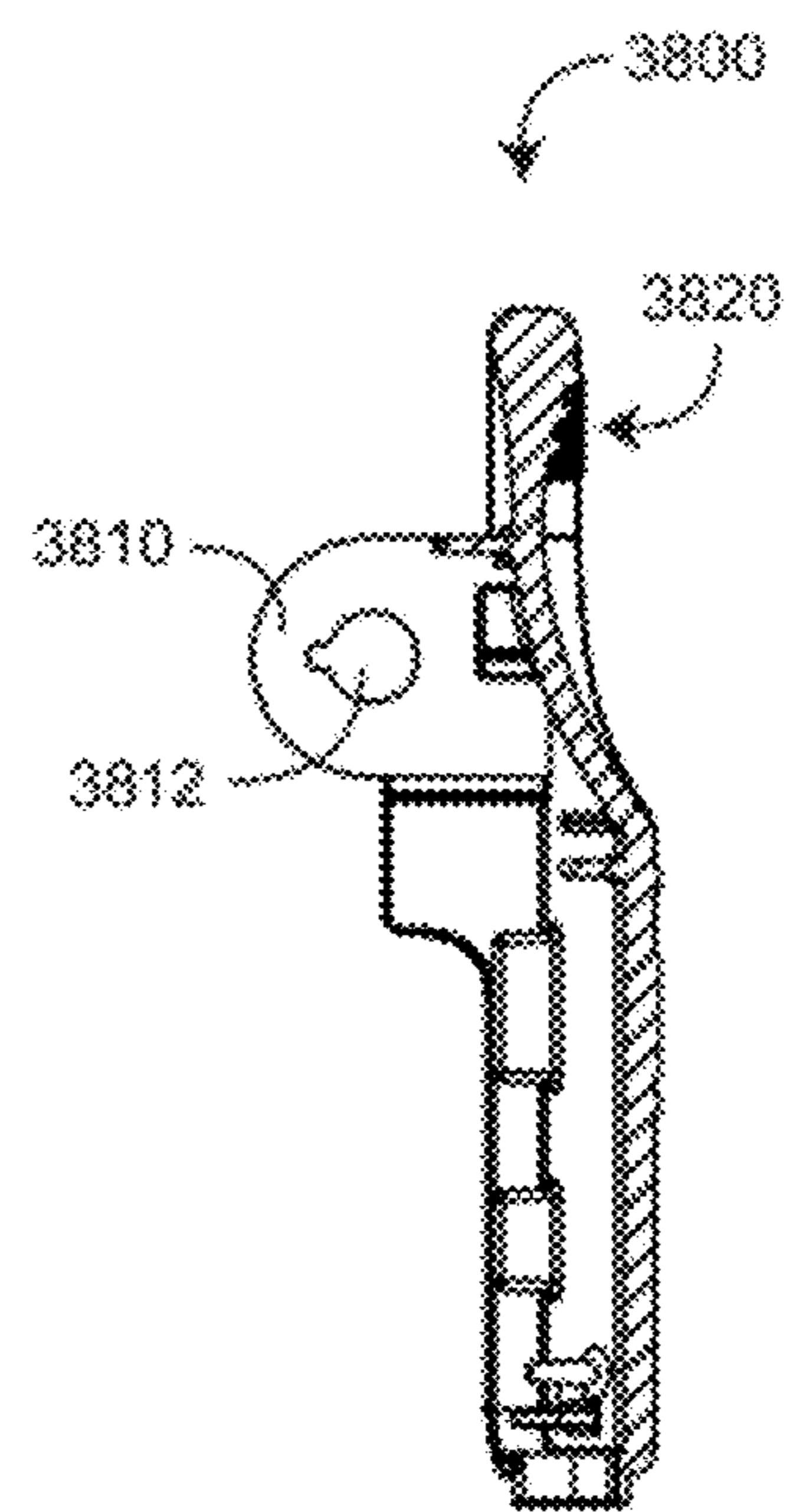
SECTION A-A FIG. 38D
