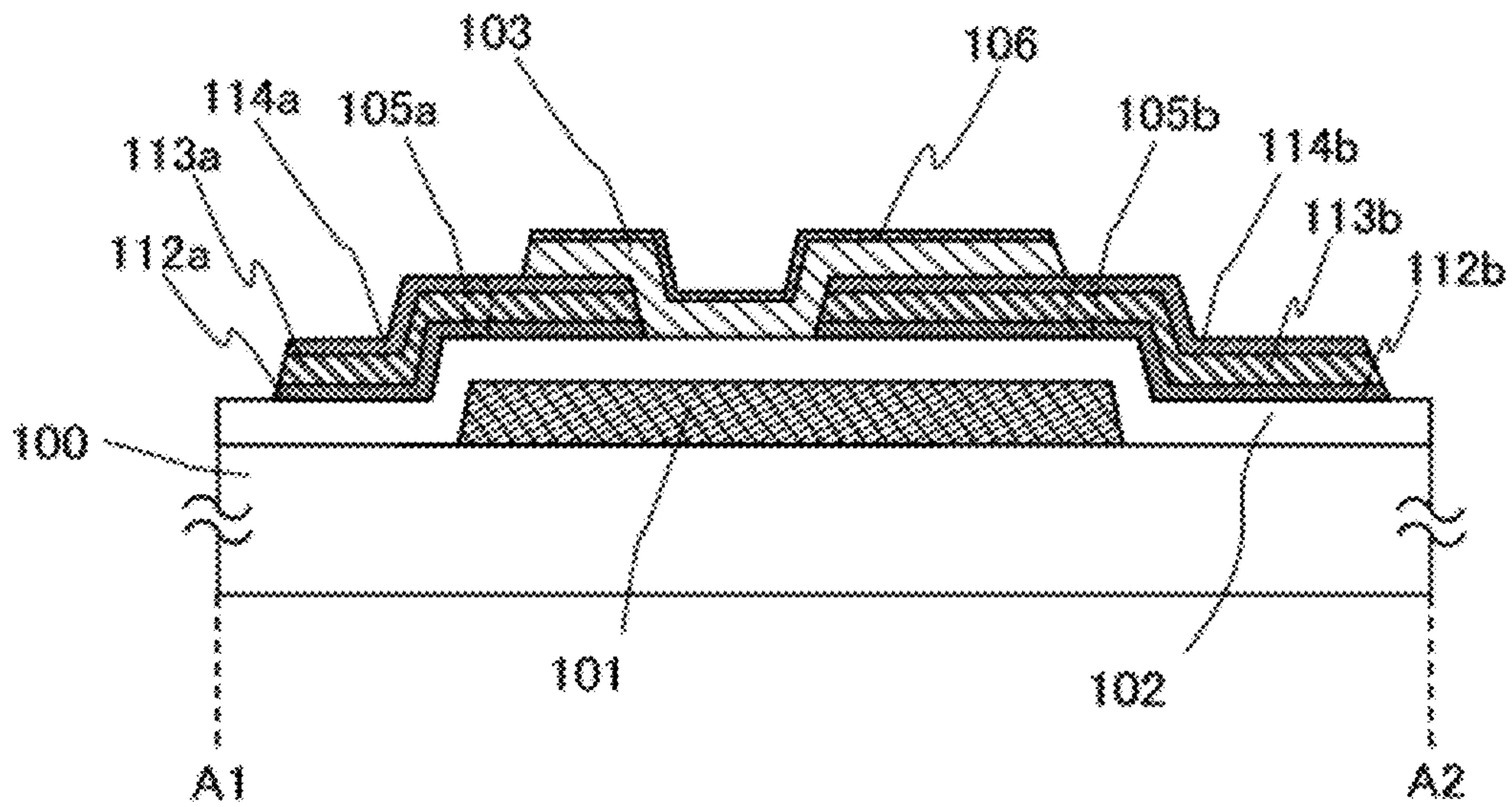
FIG. 1A
