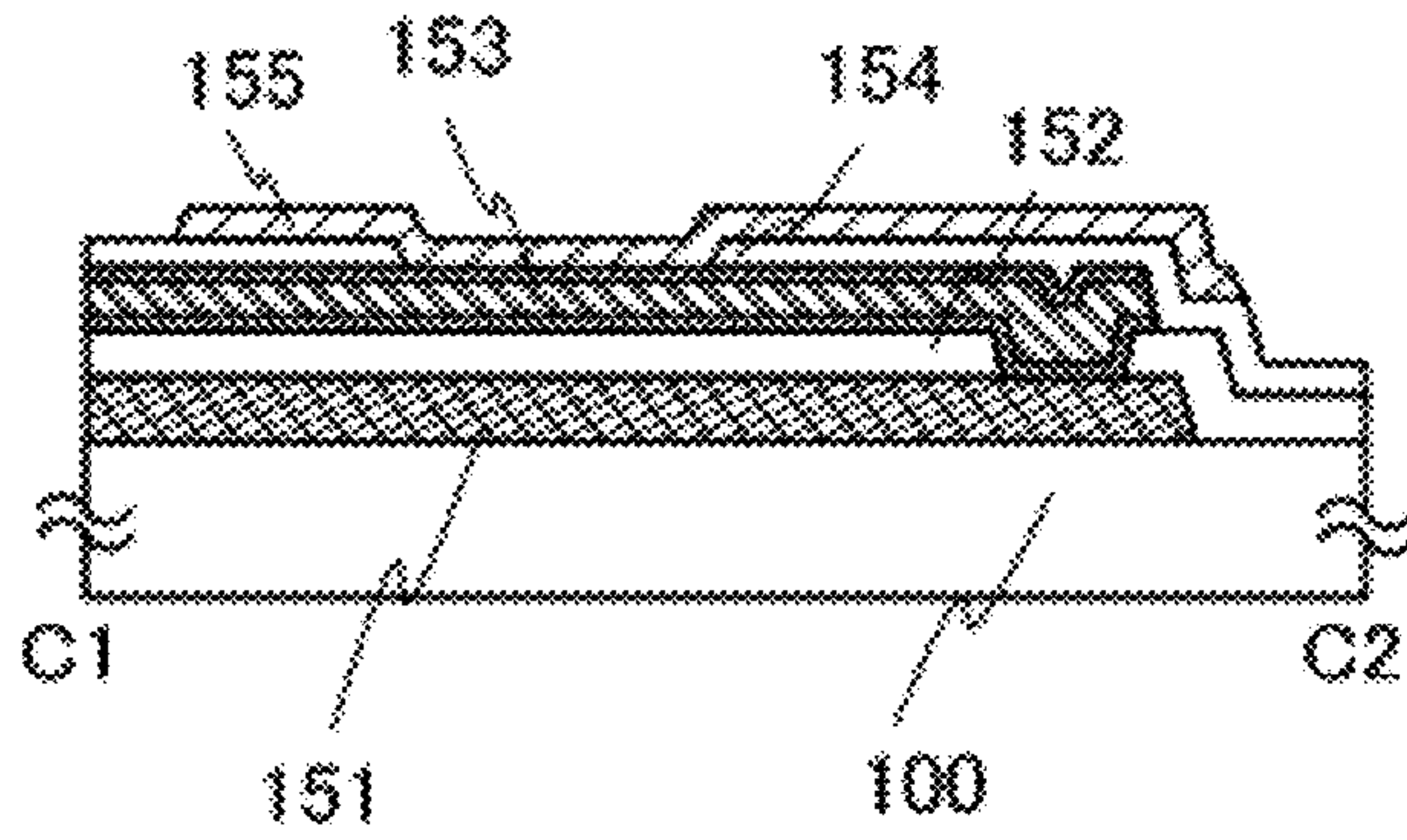
FIG. 8C
