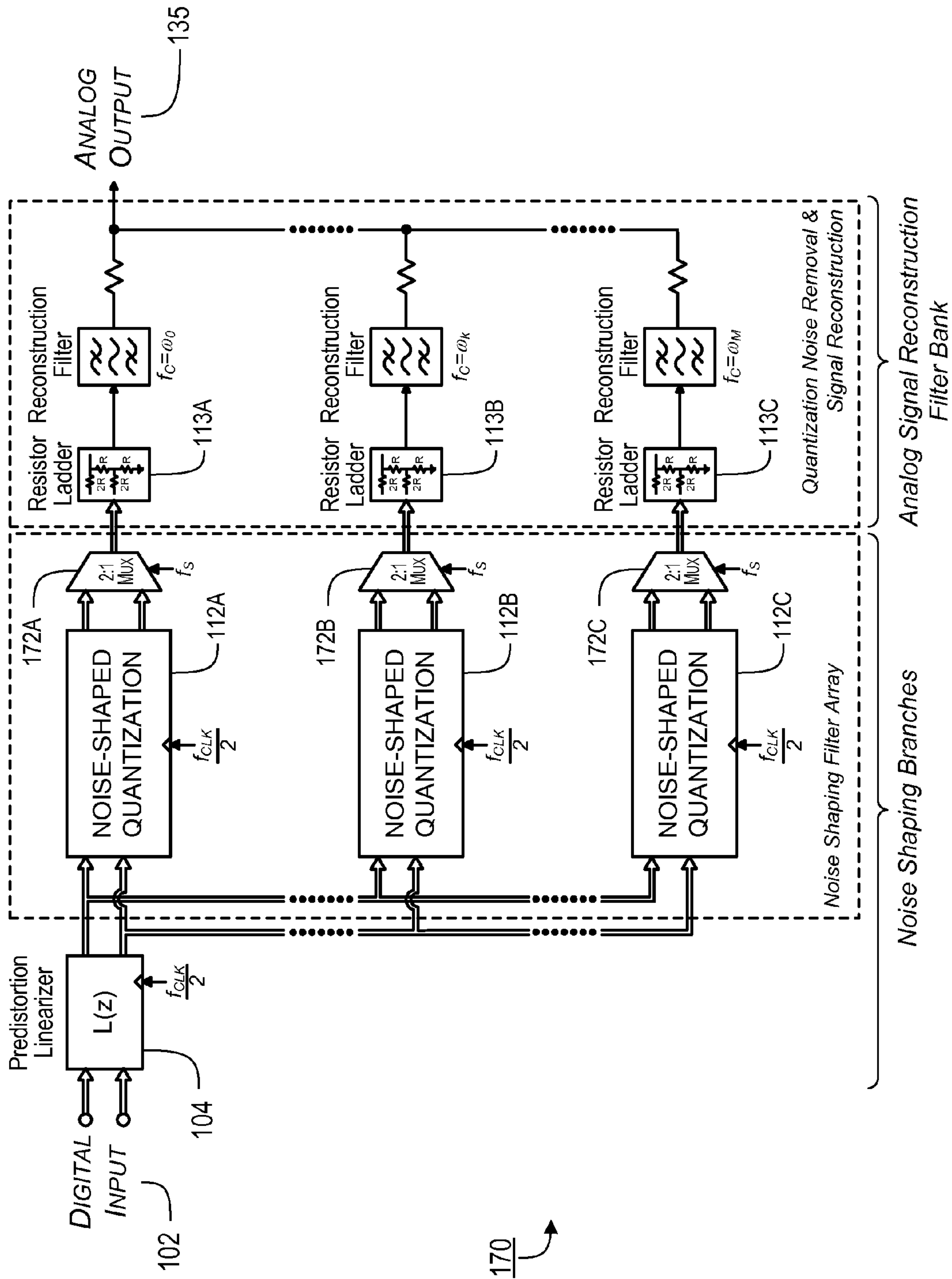
FIG. 16A
