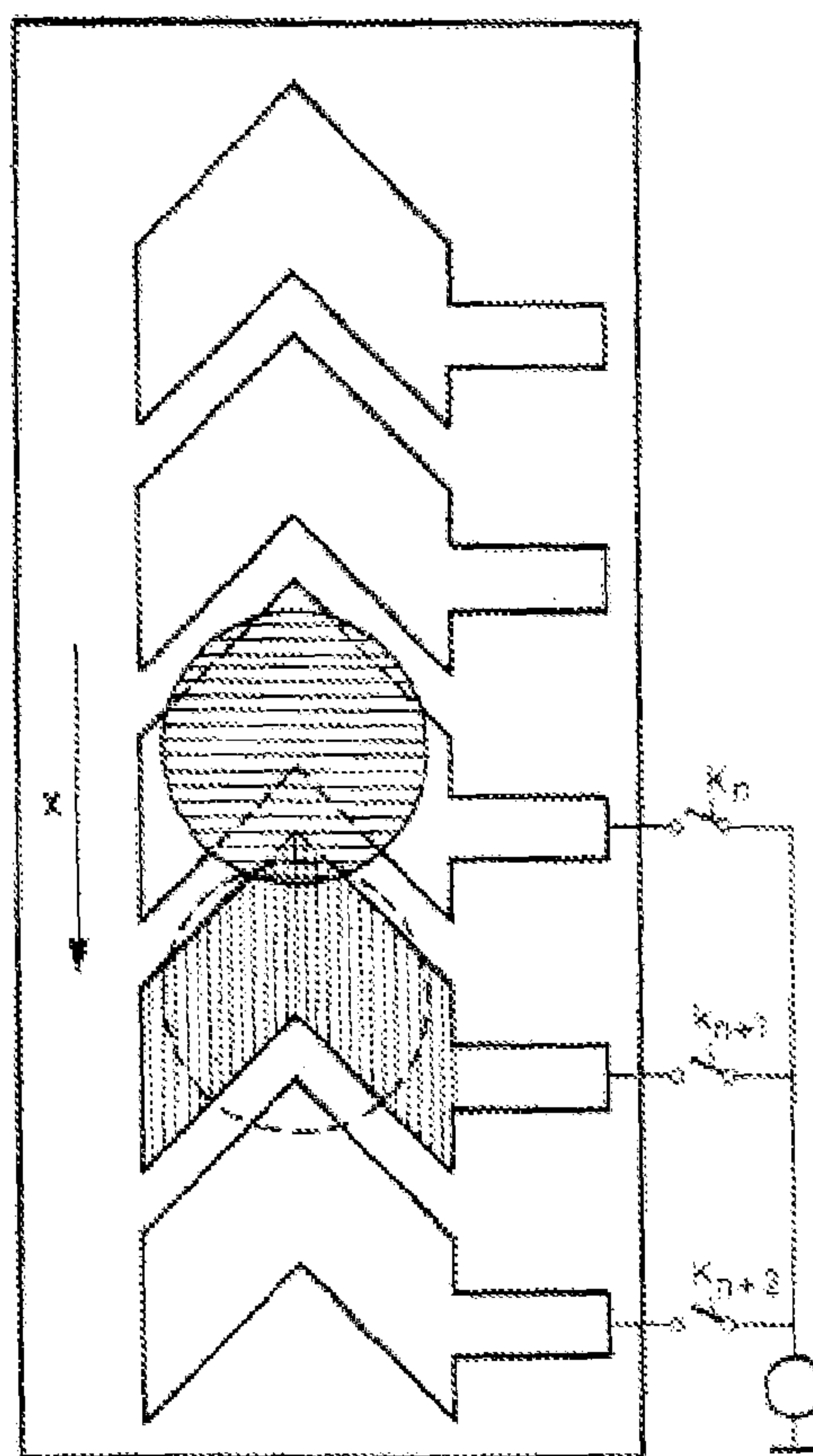
FIG. 106 (Le Pesant et al, US 4,569,575)
