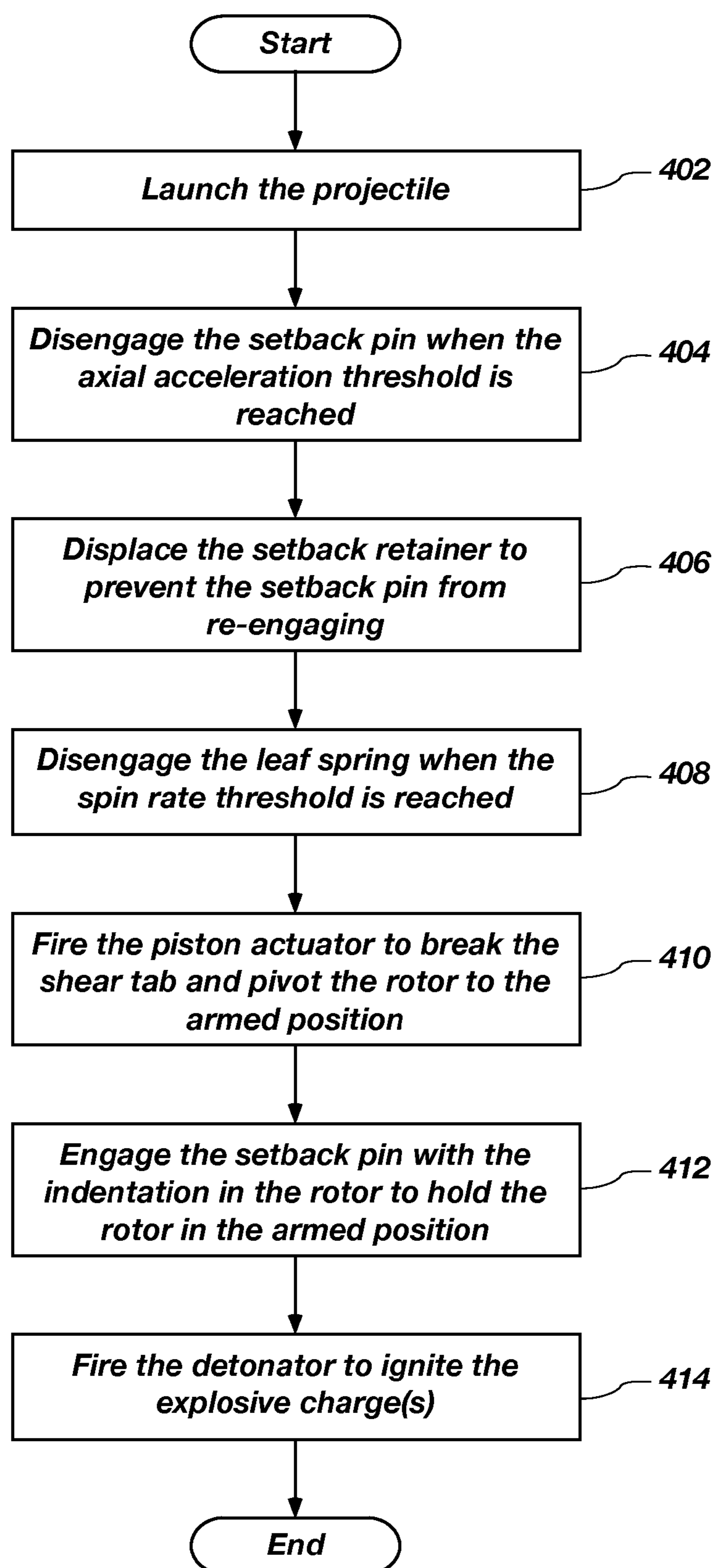
FIG. 8
