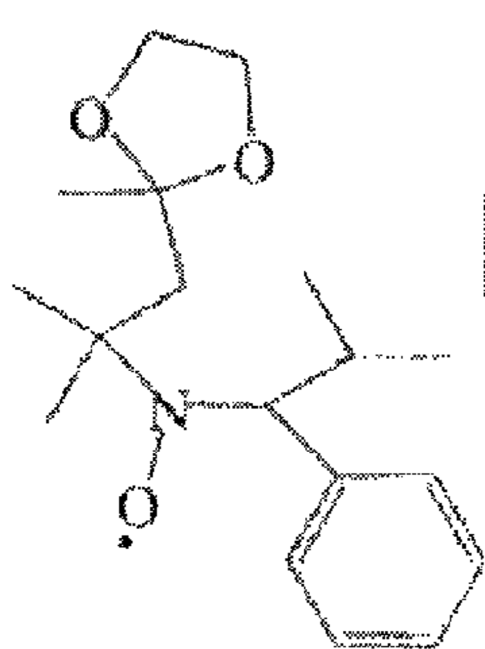
TIPNO-2, LogP=3.6
