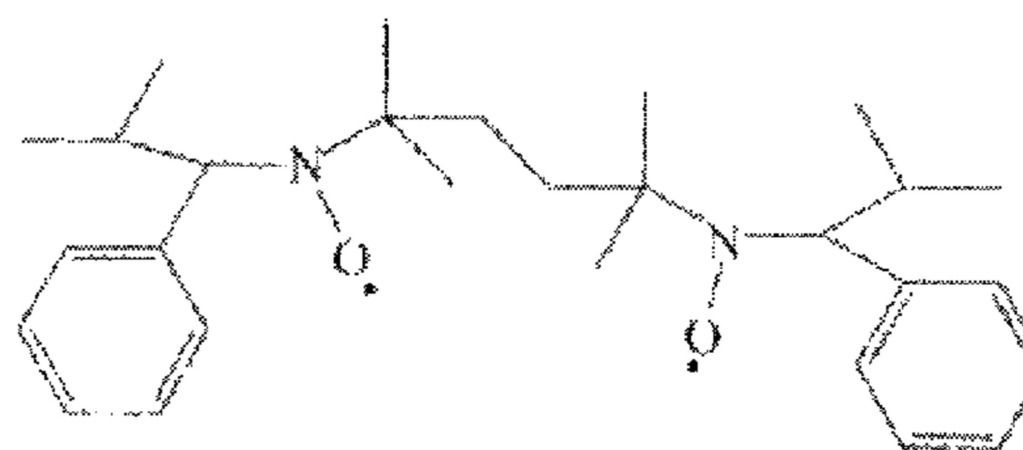
Bis-TIPNO, LogP=7.3
