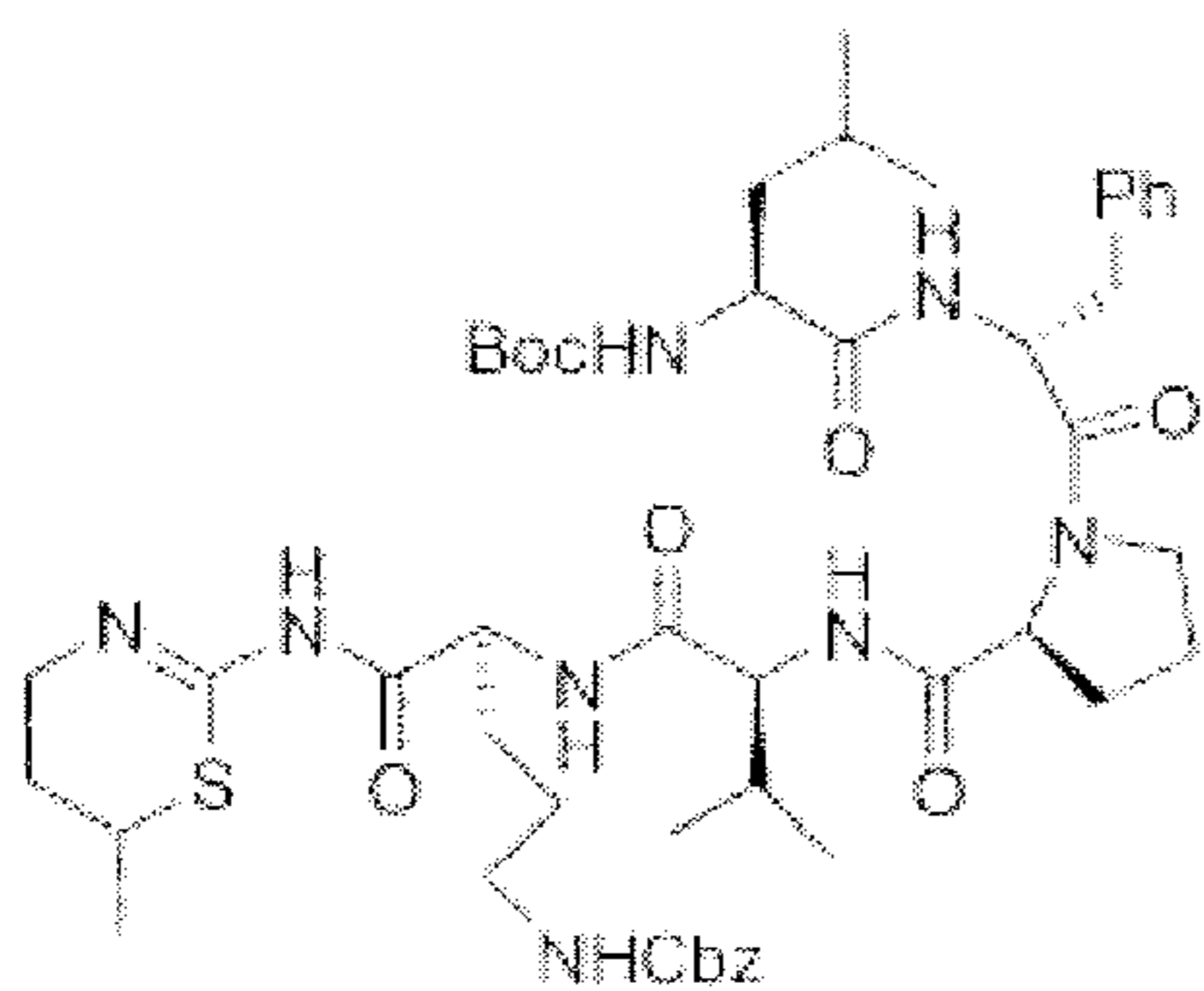
XJB-5-127
