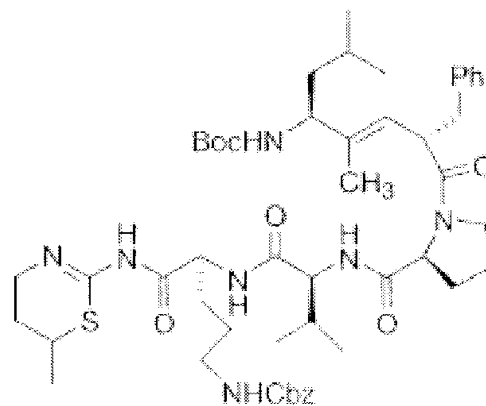
XJB-5-241
