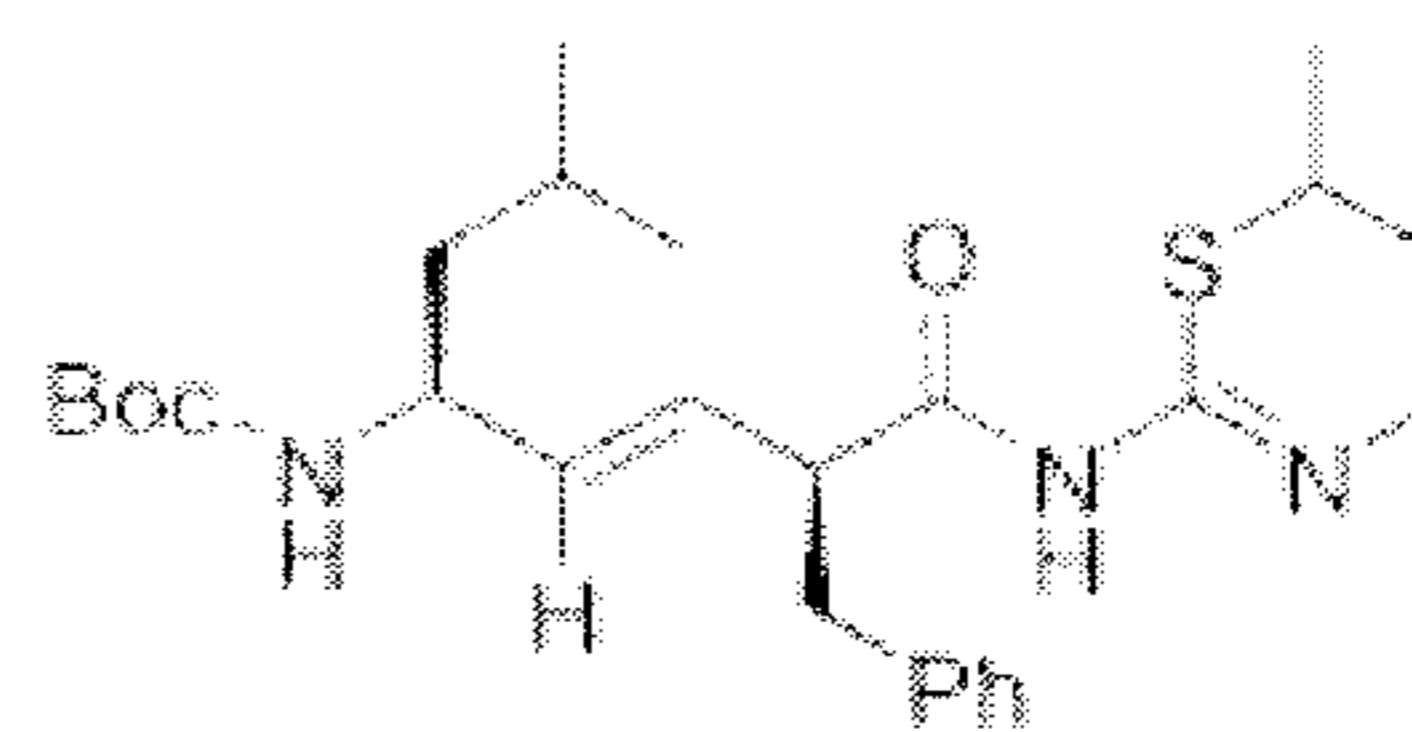
XJB-5-234
