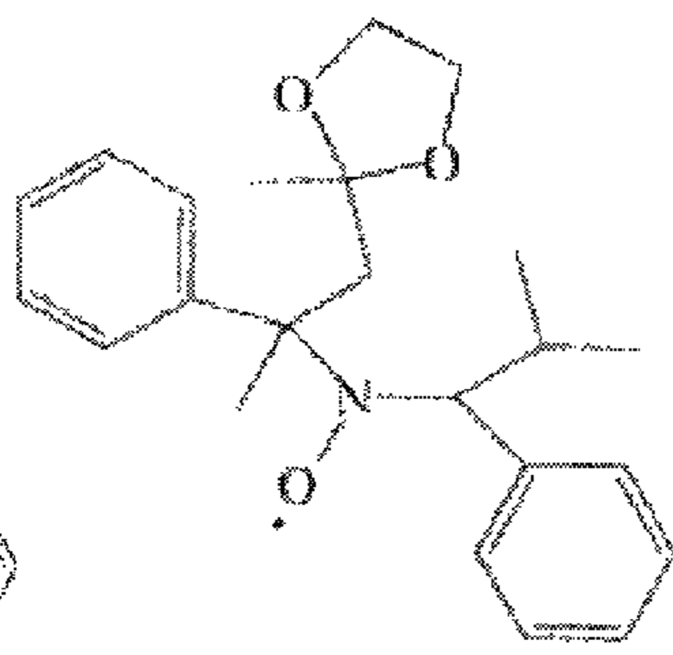
TIPNO-3, LogP=4.8
