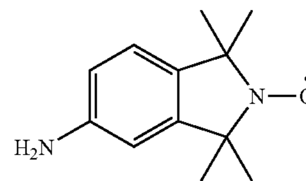
5-amino-TMIO
