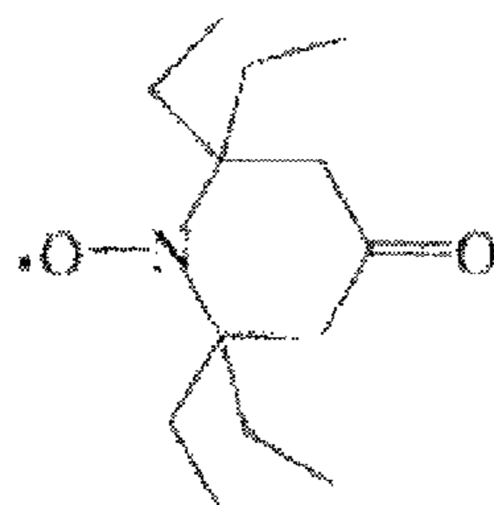
G6, LogP=3.2
